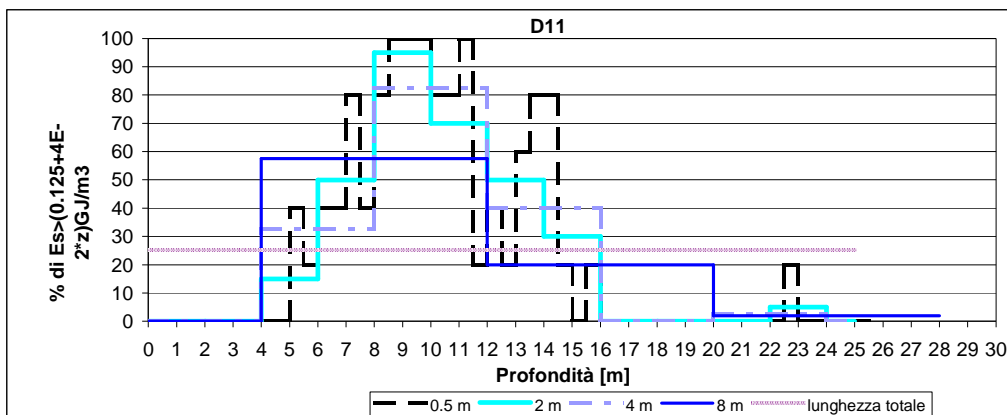
Figura 2 - Diagrafia D11, % di Es dei probabili livelli cementati con scansione: lungo tutto il sondaggio, ogni 8m, 4m, 2m, 0.5m
