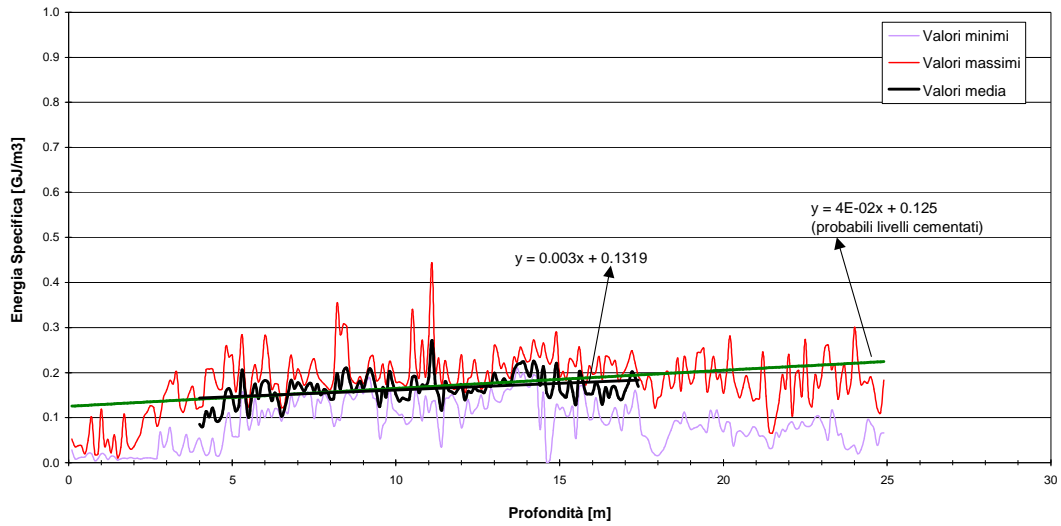
Figura 15 - Andamento dei valori minimi, medi e massimi (tra 0m e 17m circa) dell'energia specifica con relativa retta interpolante delle diagrafie D38, D11, D39
