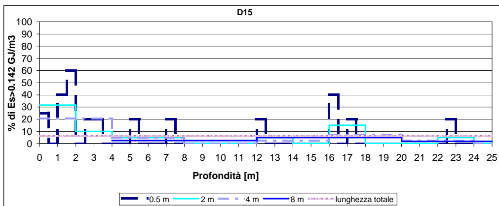
Figura 12 - Diagrafia D15, [%] di Es > 0,142 GJ/m3 con scansione: lungo tutto il sondaggio, ogni 8m, 4m, 2m, 0.5m
