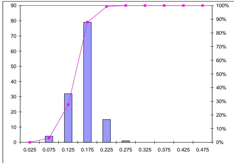
Figura 17 - Analisi statistica damento dei valori dell'energia specifica (tra 0m e 17m) delle diagrafie D38, D11, D39
