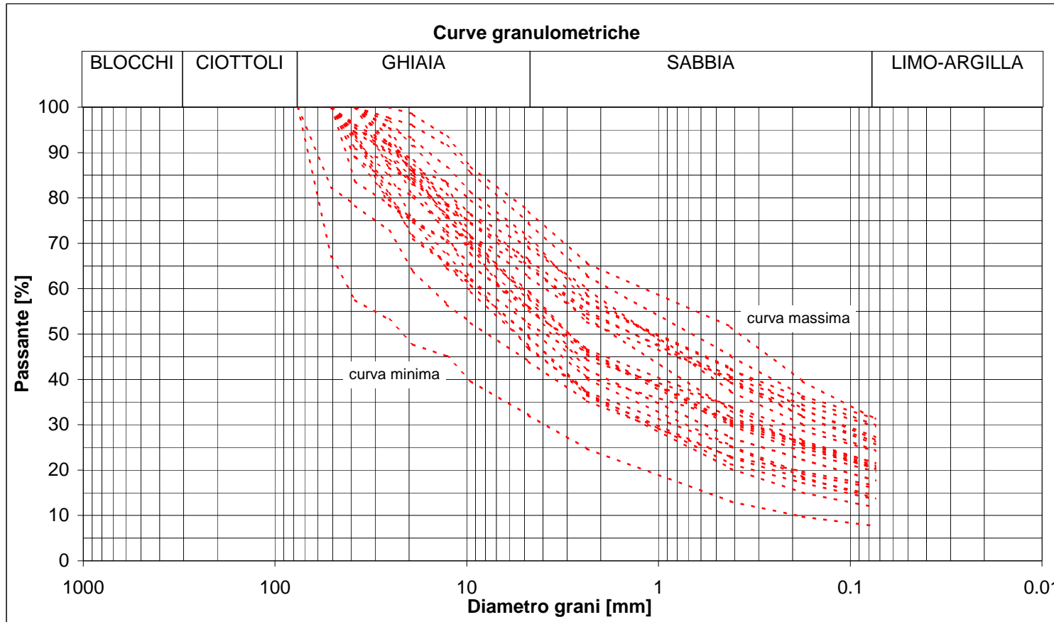
Figura 24 - Curve granulometriche dei campioni provenienti dai sondaggi (non è considerata la percentuale di ciottoli \geq 100 mm)
