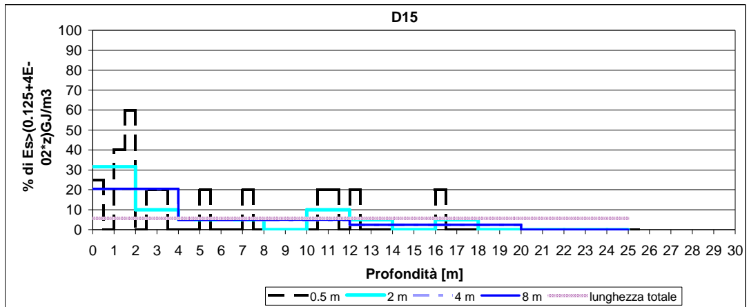
Figura 6 - Diagrafia D15, % di Es dei probabili livelli cementati con scansione: lungo tutto il sondaggio, ogni 8m, 4m, 2m, 0.5m
