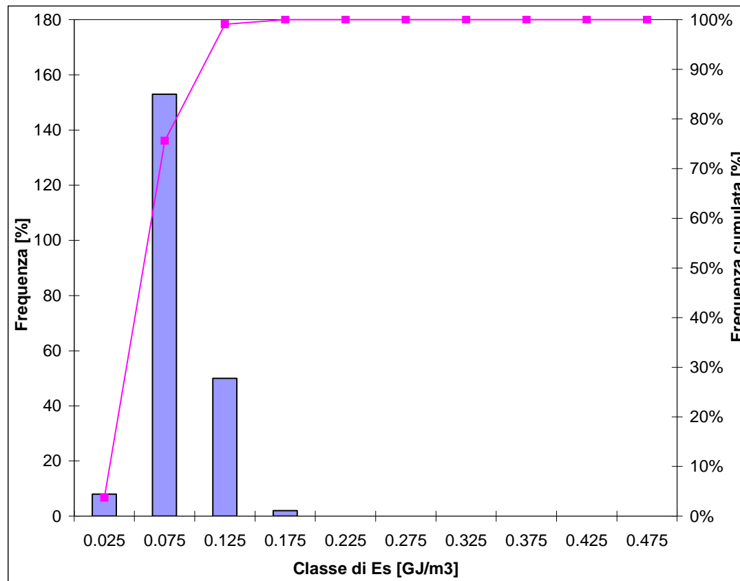
Figura 21 - Analisi statistica damento dei valori dell'energia specifica delle diagrafie D12, D40, D15
