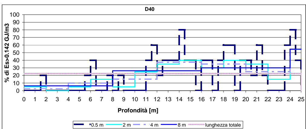
Figura 11 - Diagrafia D40, [%] di Es > 0,142 GJ/m3 con scansione: lungo tutto il sondaggio, ogni 8m, 4m, 2m, 0.5m
