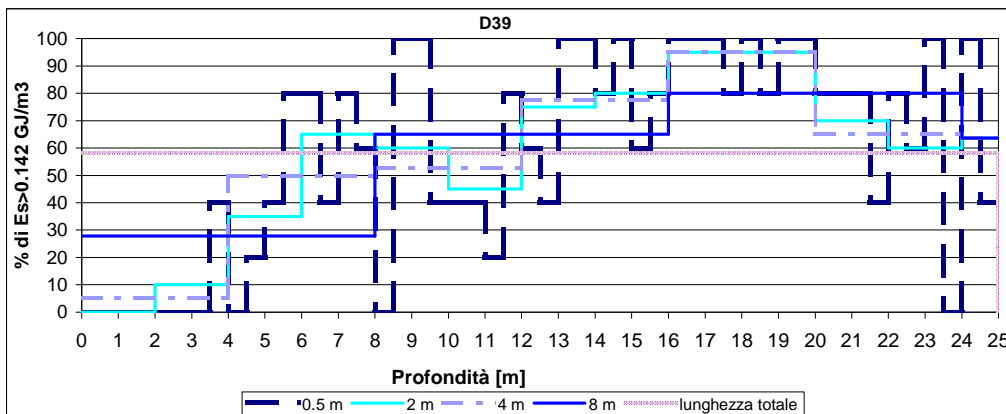
Figura 9 - Diagrafia D39, [%] di Es > 0,142 GJ/m3 con scansione: lungo tutto il sondaggio, ogni 8m, 4m, 2m, 0.5m
