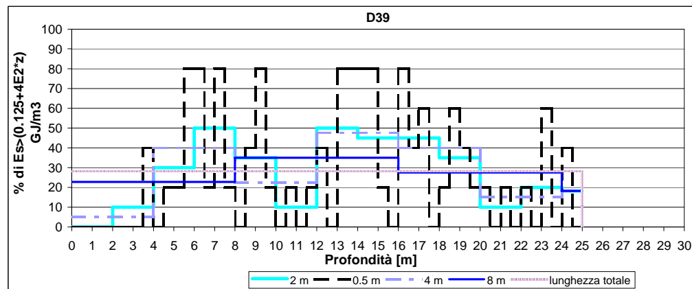
Figura 3- Diagrafia D39, % di Es dei probabili livelli cementati con scansione: lungo tutto il sondaggio, ogni 8m, 4m, 2m, 0.5m
