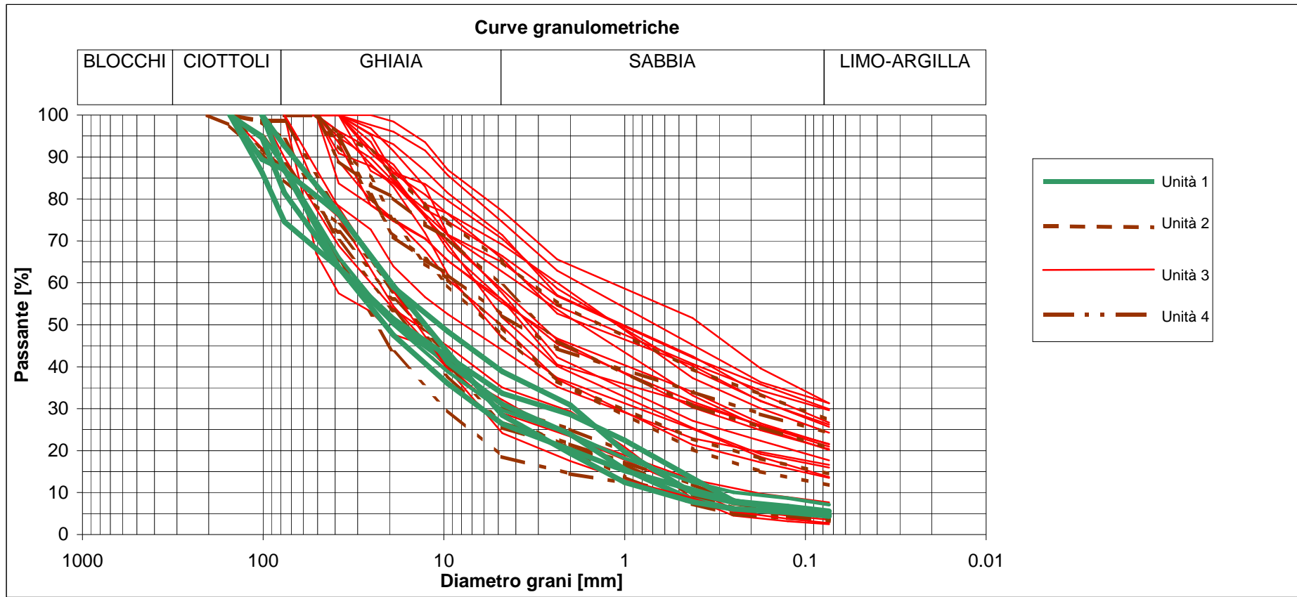
Figura 26 - Curve granulometriche dei campioni provenienti dai sondaggi e dai pozzi, suddivisi per unità geotecniche
