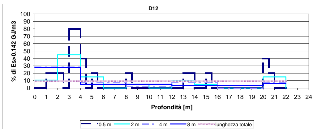
Figura 10 - Diagrafia D12, [%] di Es > 0,142 GJ/m3 con scansione: lungo tutto il sondaggio, ogni 8m, 4m, 2m, 0.5m
