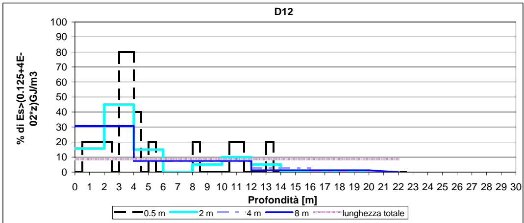
Figura 4- Diagrafia D12, % di Es dei probabili livelli cementati con scansione: lungo tutto il sondaggio, ogni 8m, 4m, 2m, 0.5m
