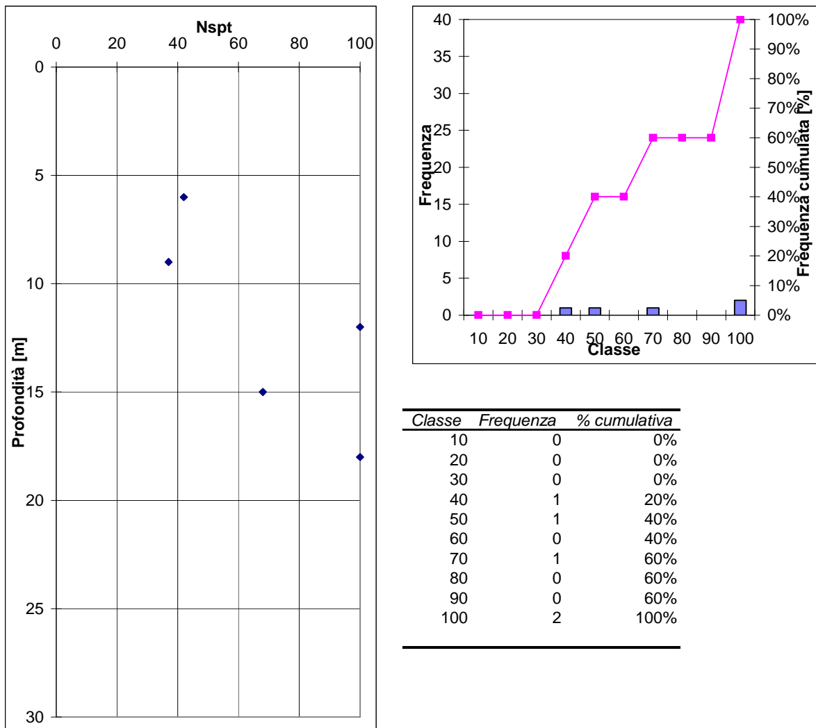
Figura 23 - Interpretazione dei dati di SPT: zona Racconigi-Acaja
