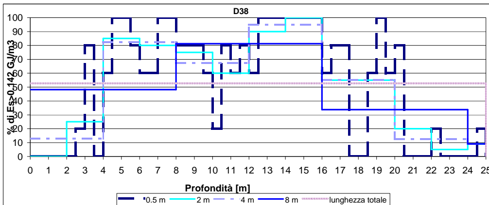
Figura 7 - Diagrafia D38, [%] di Es > 0,142 GJ/m3 con scansione: lungo tutto il sondaggio, ogni 8m, 4m, 2m, 0.5m
