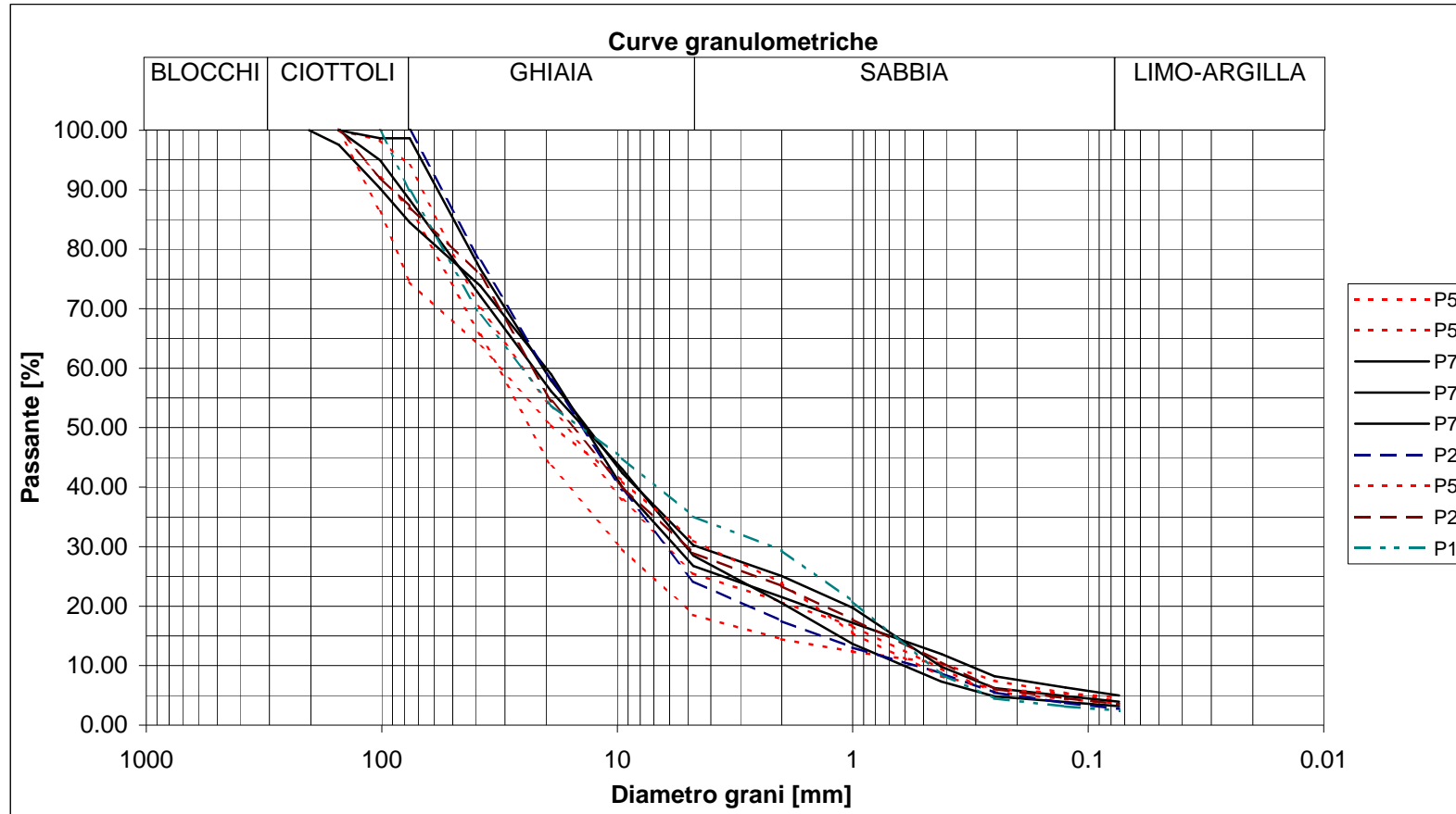
Figura 25 - Curve granulometriche integrali dei campioni provenienti dai pozzi P1, P2, P5 e P7 (è considerata la percentuale di ciottoli \geq 100\text{mm} )
