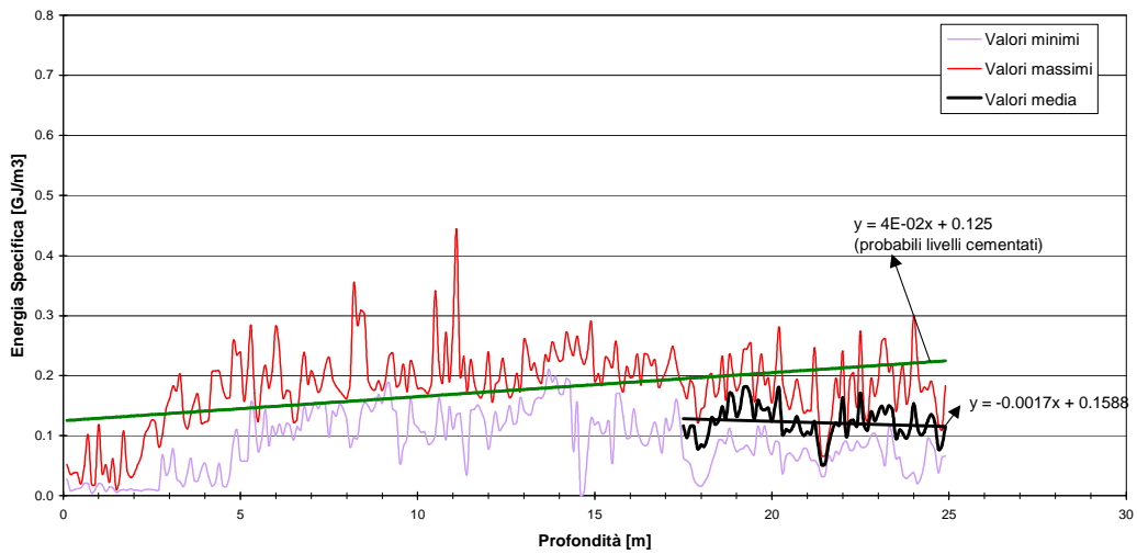
Figura 16 - Andamento dei valori minimi, medi e massimi (tra 17m circa e 25m) dell'energia specifica con relativa retta interpolante delle diagrafie D38, D11, D39
