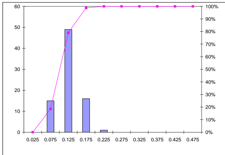
Figura 18 - Analisi statistica damento dei valori dell'energia specifica (tra 17m e 25m) delle diagrafie D38, D11, D39
