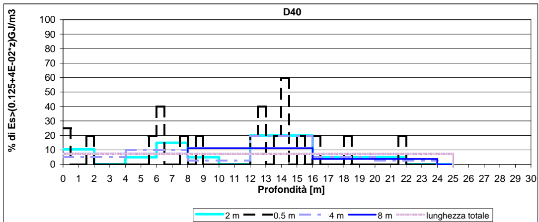
Figura 5- Diagrafia D40, % di Es dei probabili livelli cementati con scansione: lungo tutto il sondaggio, ogni 8m, 4m, 2m, 0.5m
