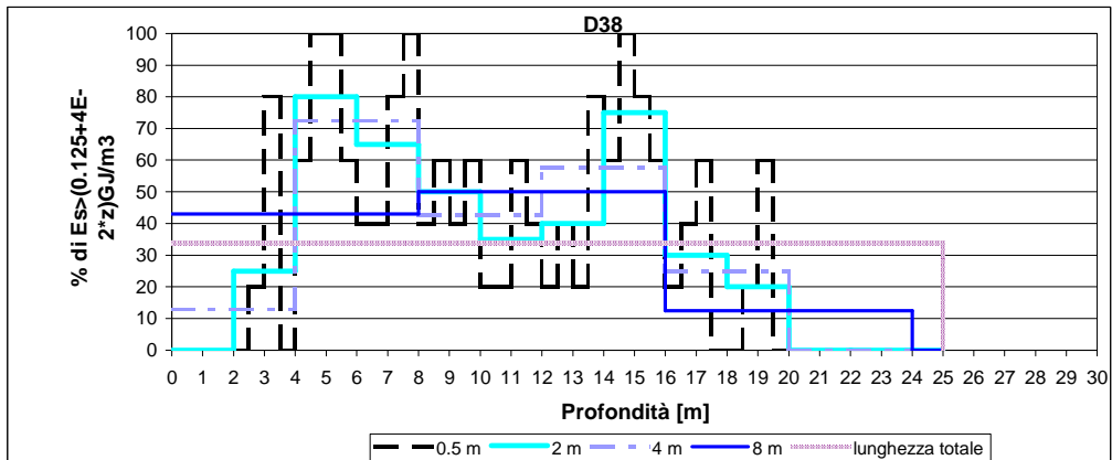
Figura 1 - Diagrafia D38, % di Es dei probabili livelli cementati con scansione: lungo tutto il sondaggio, ogni 8m, 4m, 2m, 0.5m
