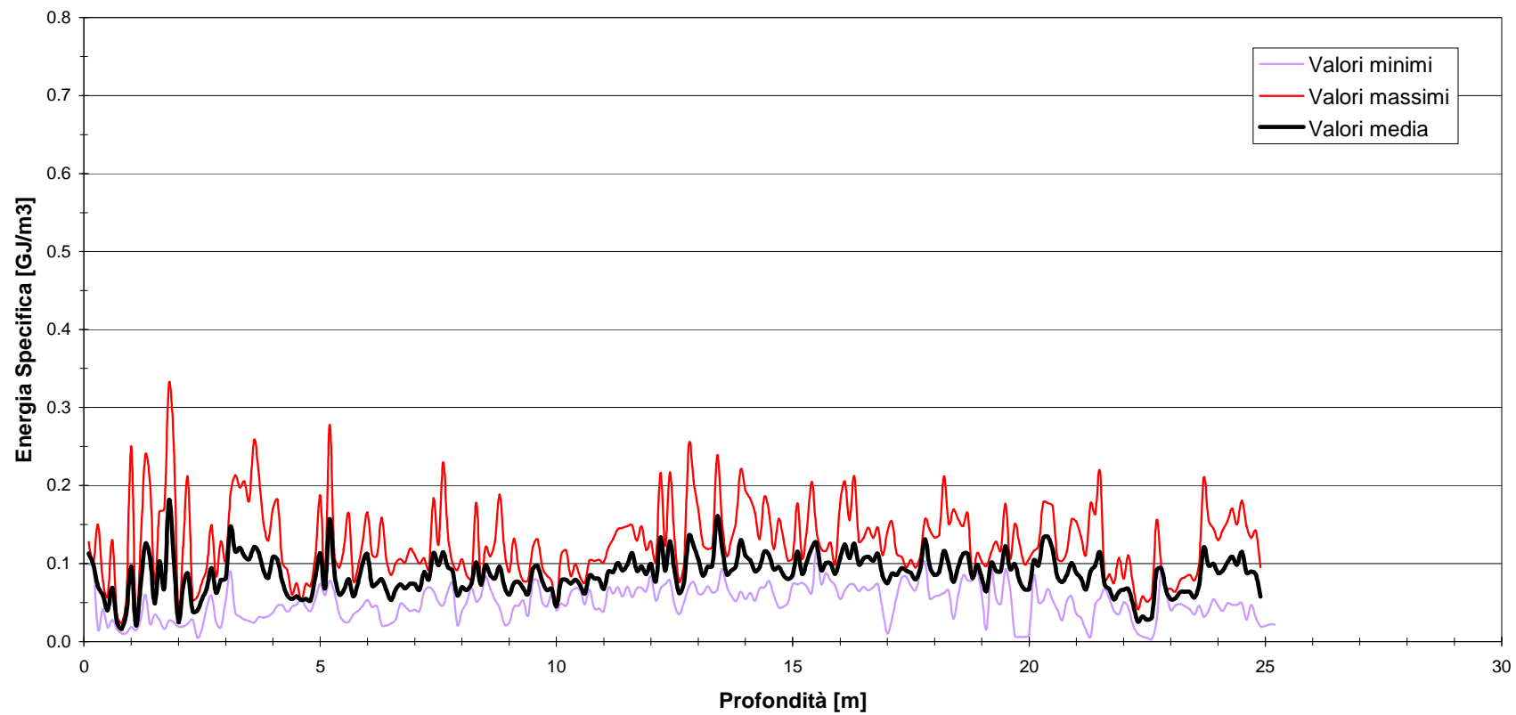
Figura 19 - Andamento dei valori minimi, medi e massimi dell'energia specifica delle diagrafie D12, D40, D15
