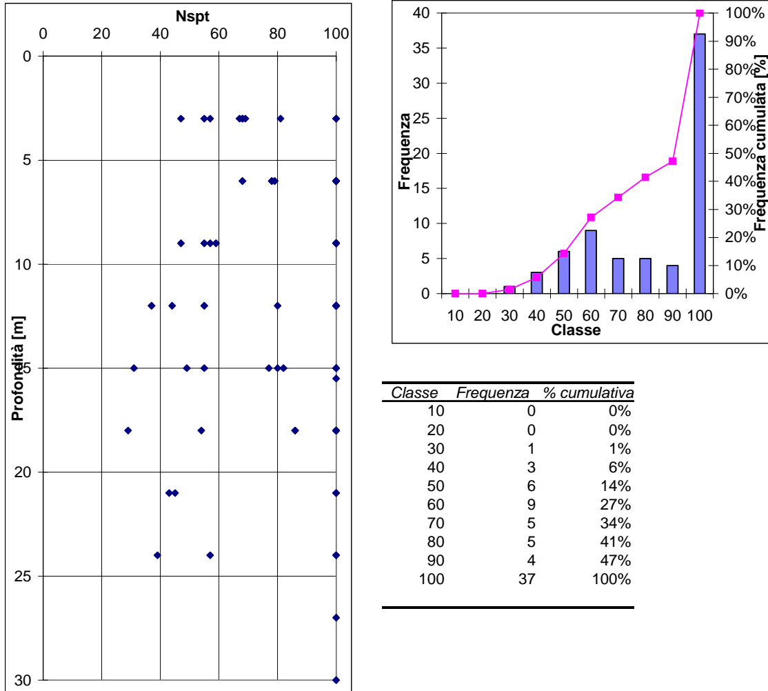
Figura 22 - Interpretazione dei dati di SPT: zona Deposito-Racconigi
