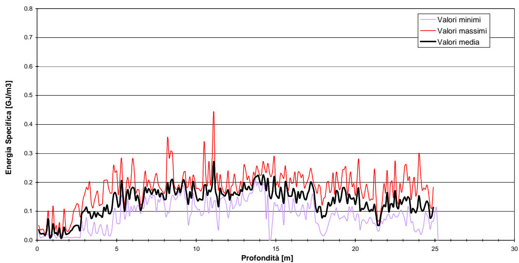
Figura 14 - Andamento dei valori minimi, medi e massimi dell'energia specifica delle diagrafie D38, D11, D39
