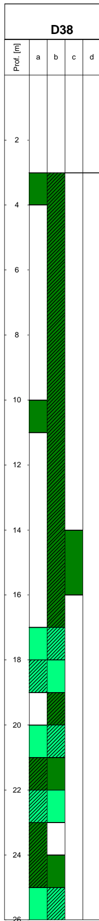
Diagrafia D38 – Andamento dell'affidabilità con la profondità
