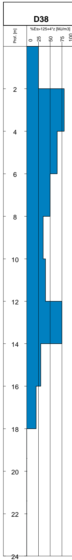
Diagrafia D38 - Andamento della cementazione con la profondità
