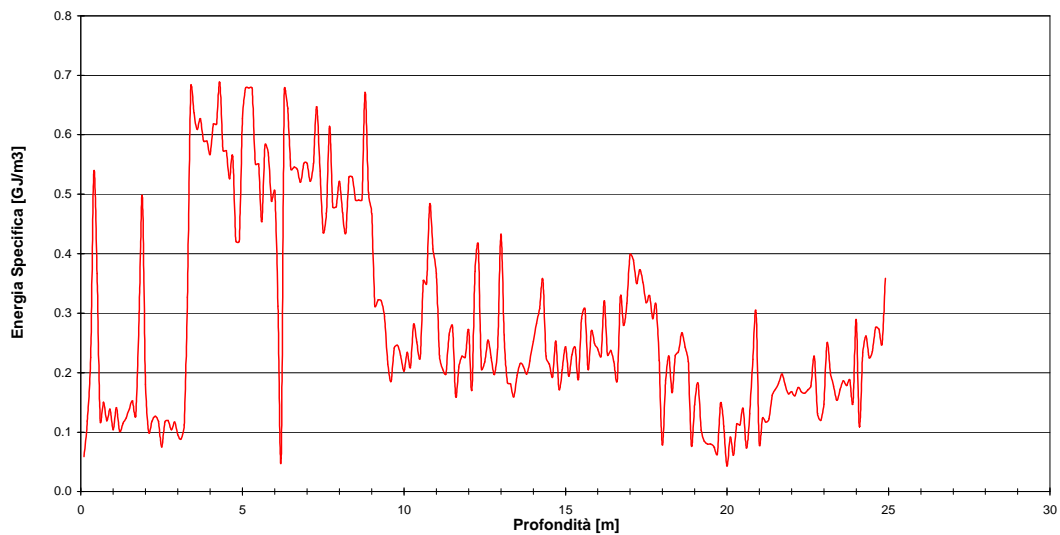
Figura 13 - Andamento dei valori dell'energia specifica della diagrafia D8
