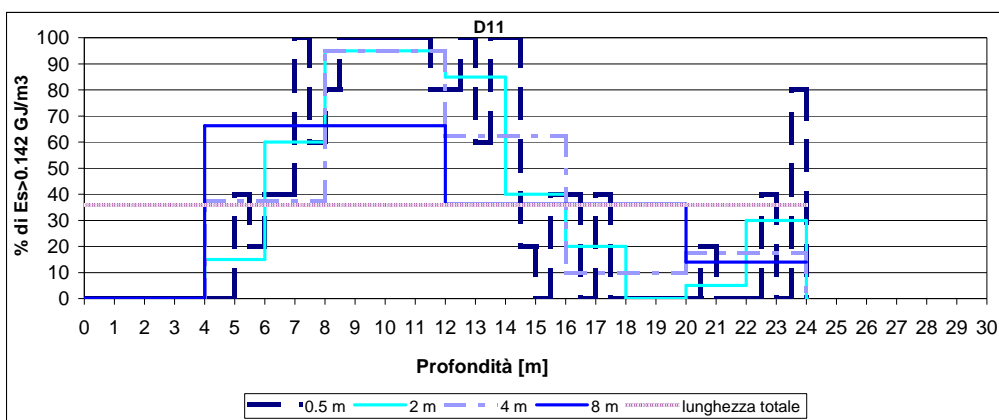
Figura 8 - Diagrafia D11, [%] di Es > 0,142 GJ/m3 con scansione: lungo tutto il sondaggio, ogni 8m, 4m, 2m, 0.5m
