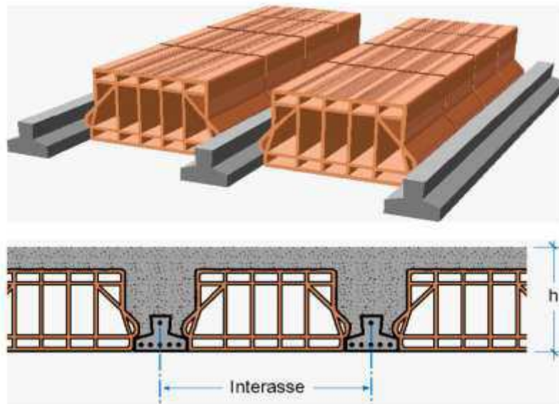
Esempio di solaio in cemento armato a travetti in cemento armato e blocchi interposti (fonte: Laterificio Pugliese s.p.a.)
