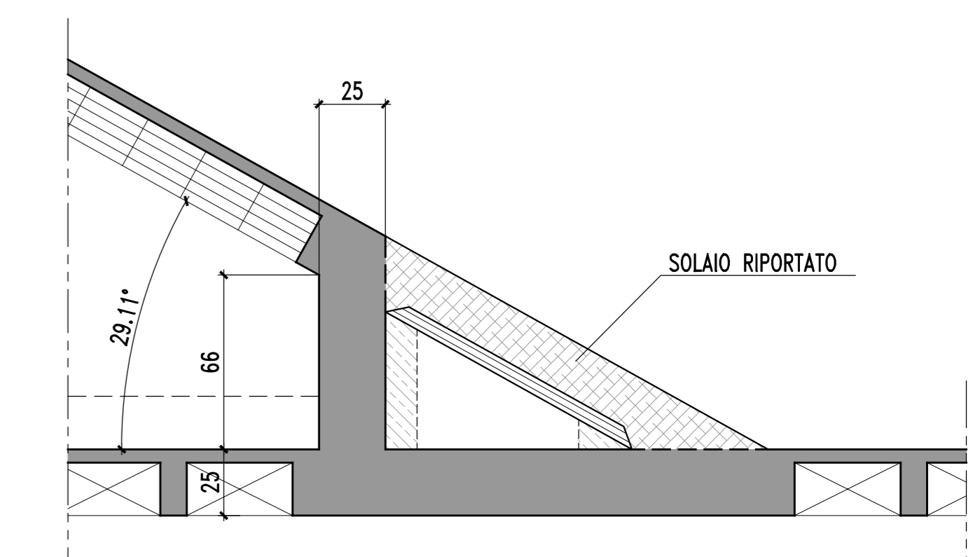
SEZIONE S2 scala 1:20
