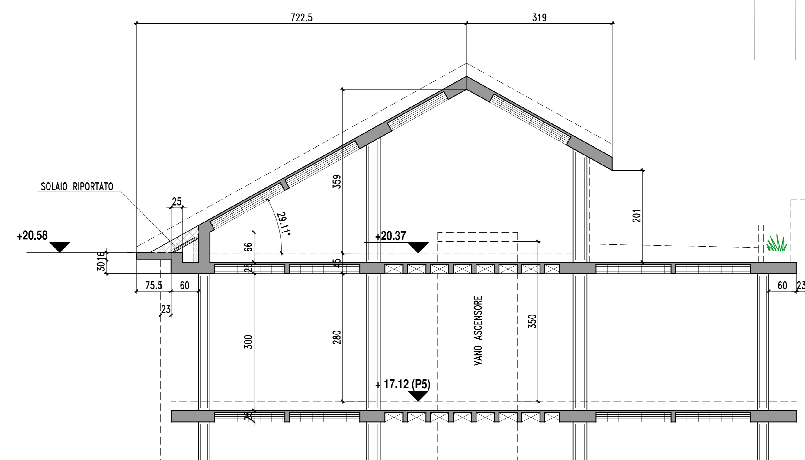
SEZIONE S1
