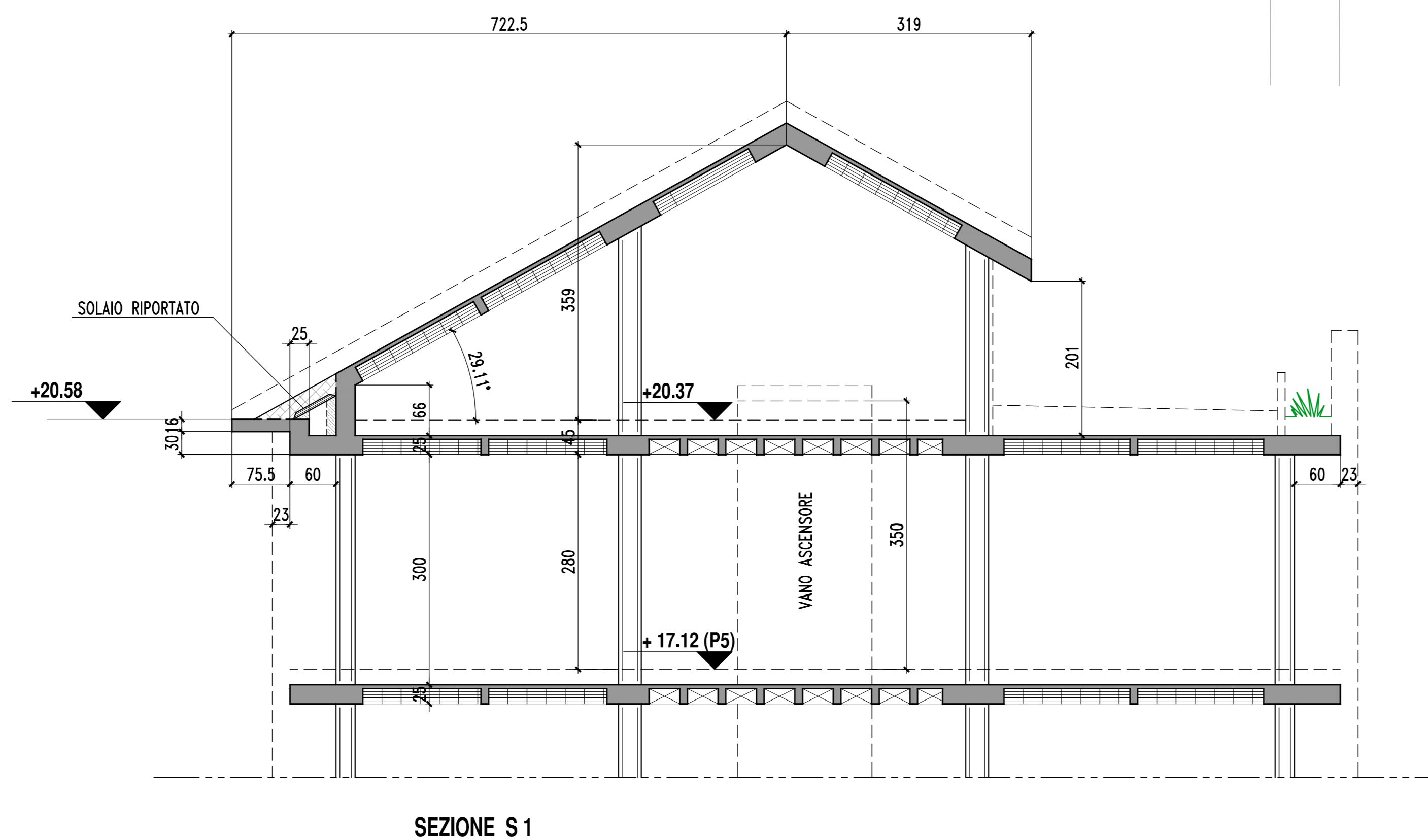
SEZIONE S1
