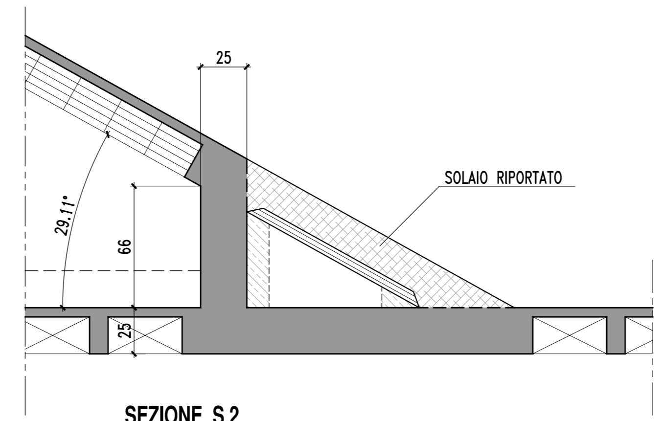
SEZIONE S 2 scala 1:20
