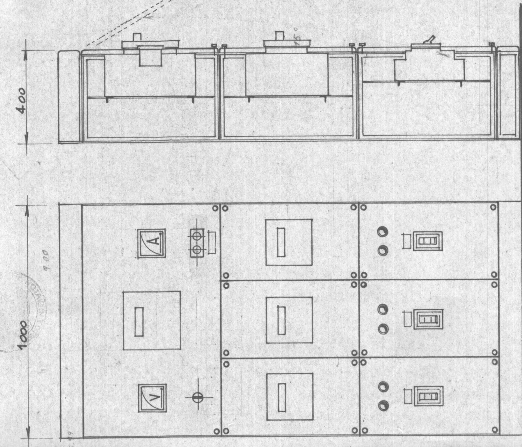
QUADRO GENERALE CENTRALE TERMICA # 11.10
