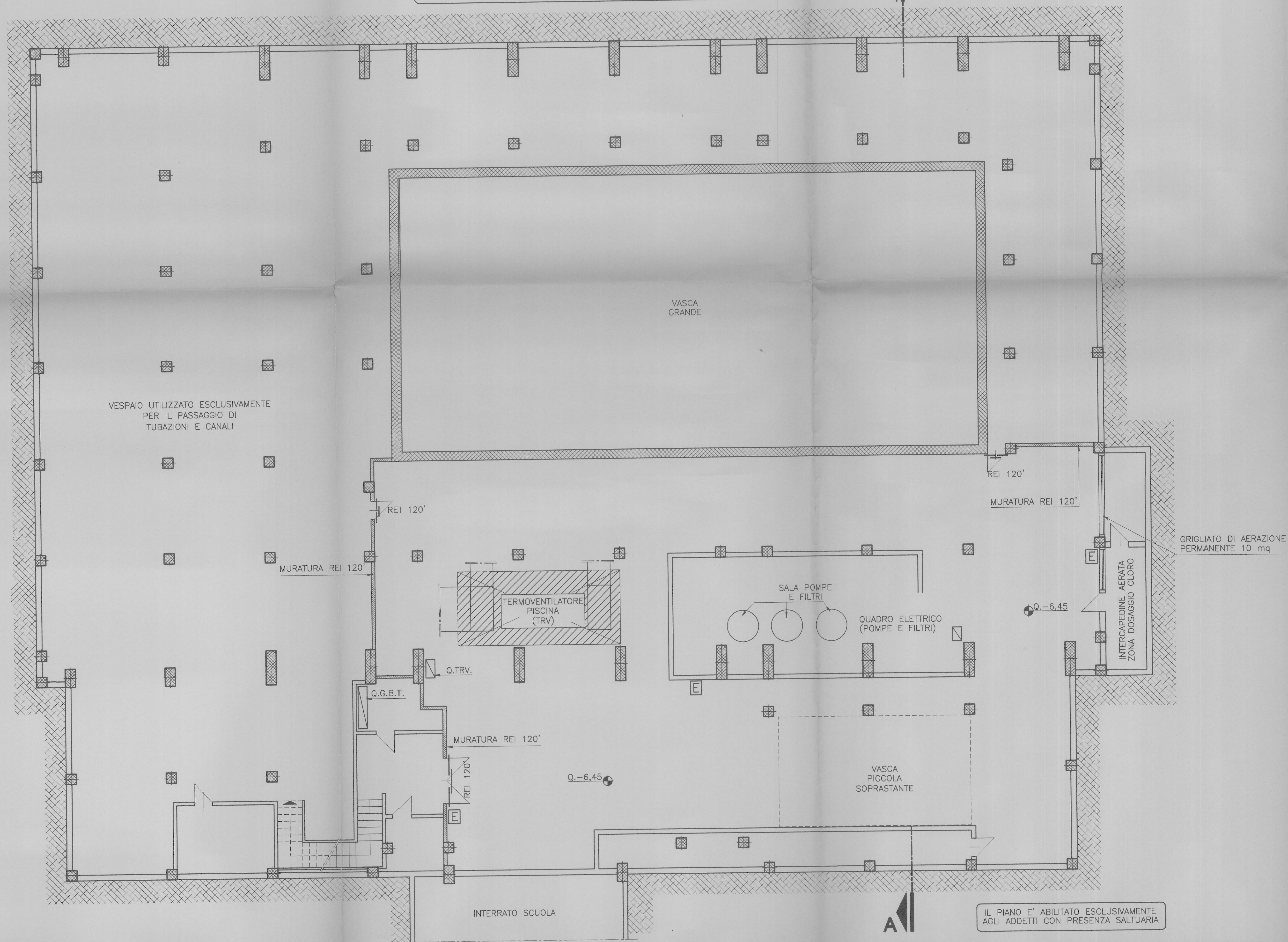
PIANTA PIANO INTERRATO SCALA 1:100
