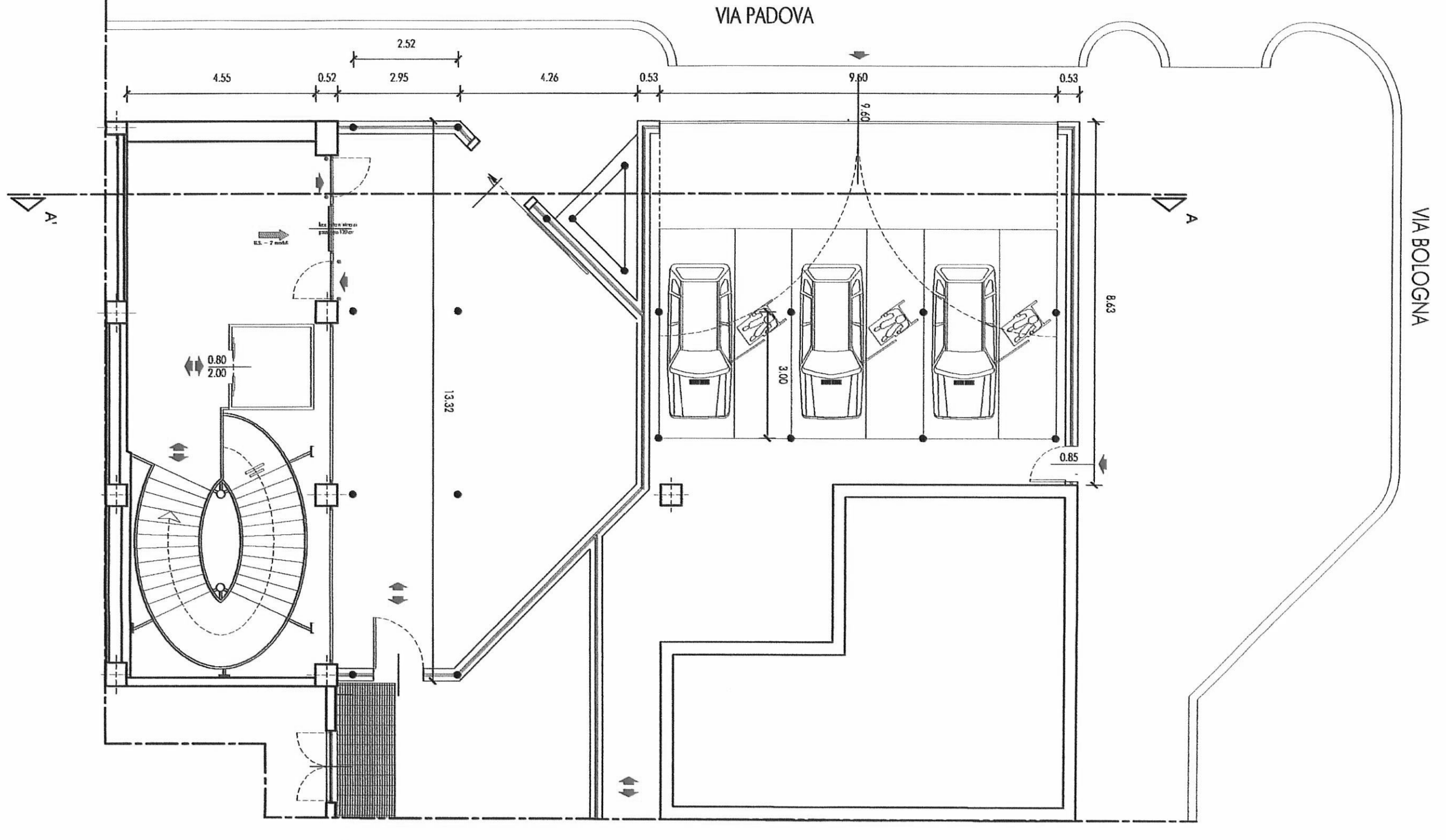
STRALCIO DI PIANTA PIANO TERRA SCALA 1:100
