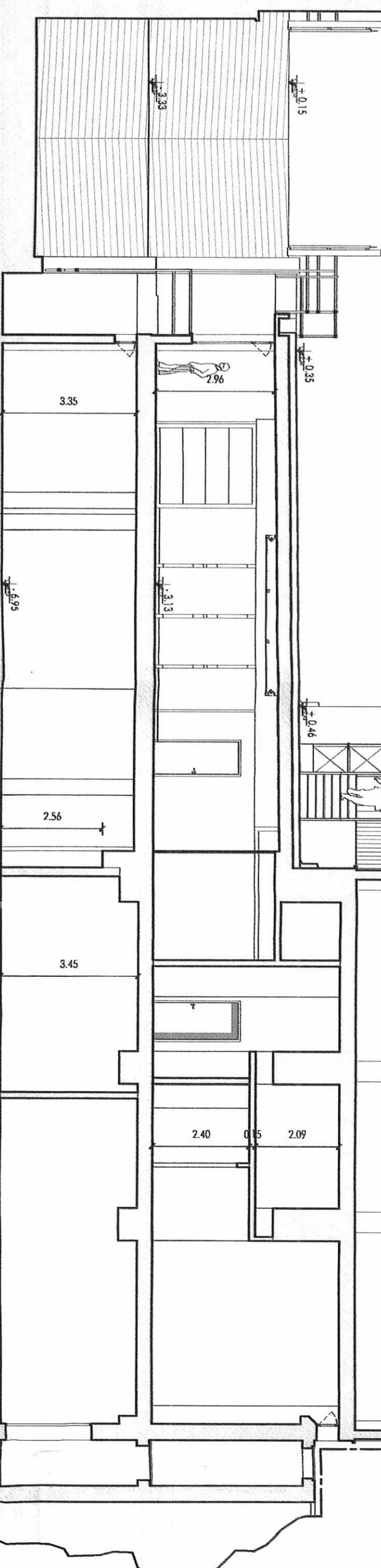
STRALCIO SEZIONE B-B'
