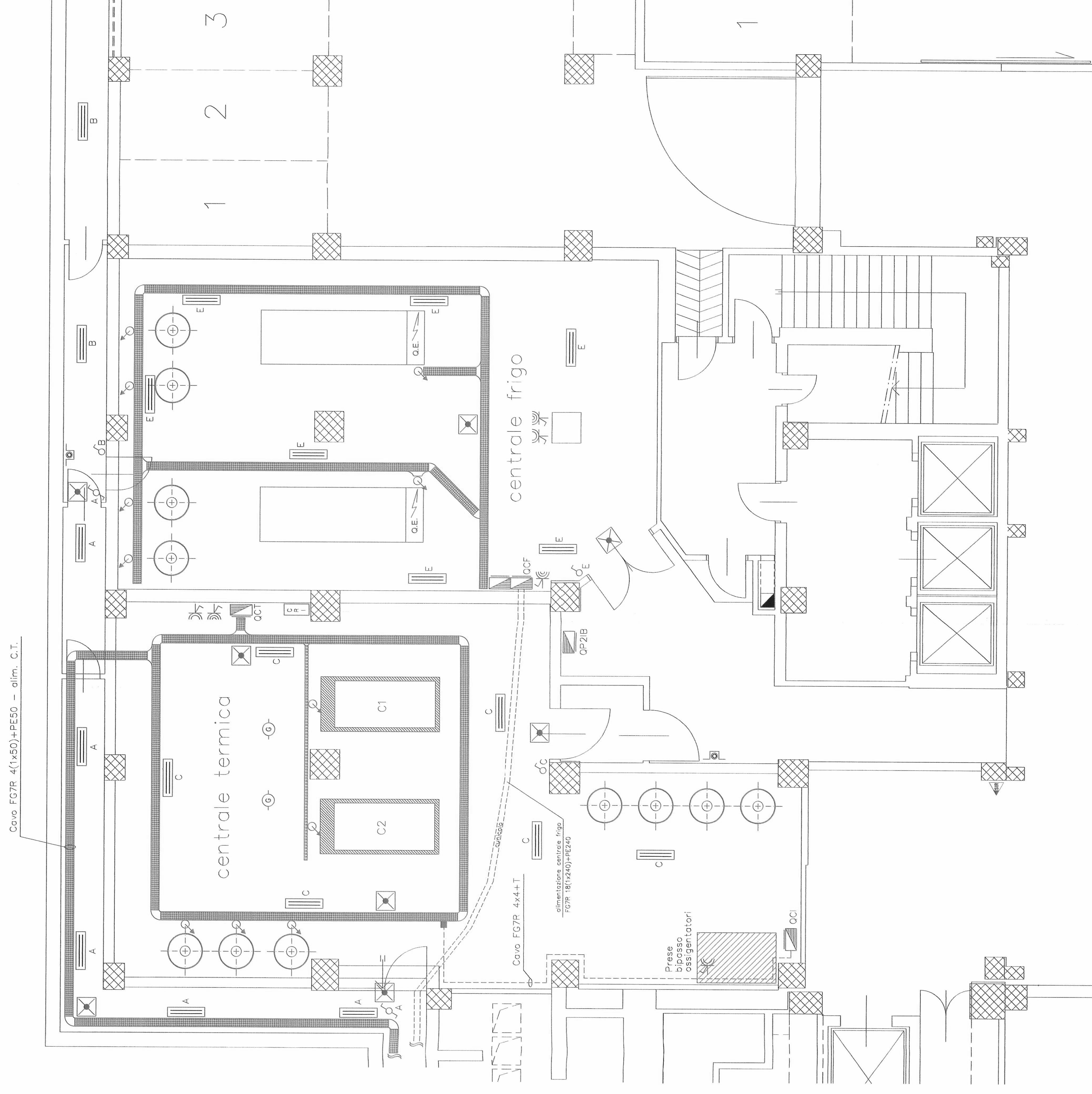
STRALCIOPIANTA PIANO SEMINTERRATO P-2 SCALA 1:50 (CENTRALE TERMICA E FRIGORIGENA)
