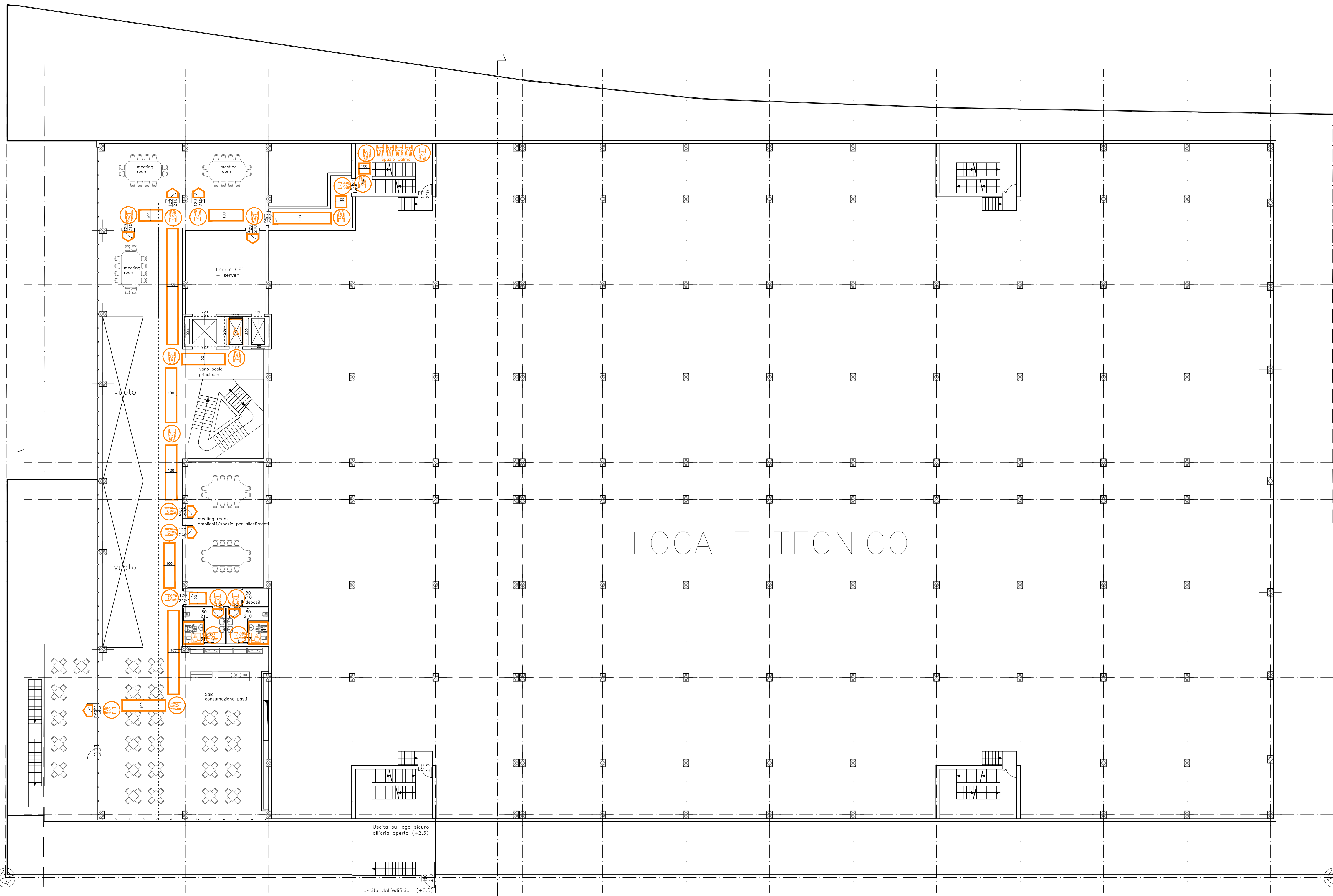
PIANTA DEL PIANO PRIMO
