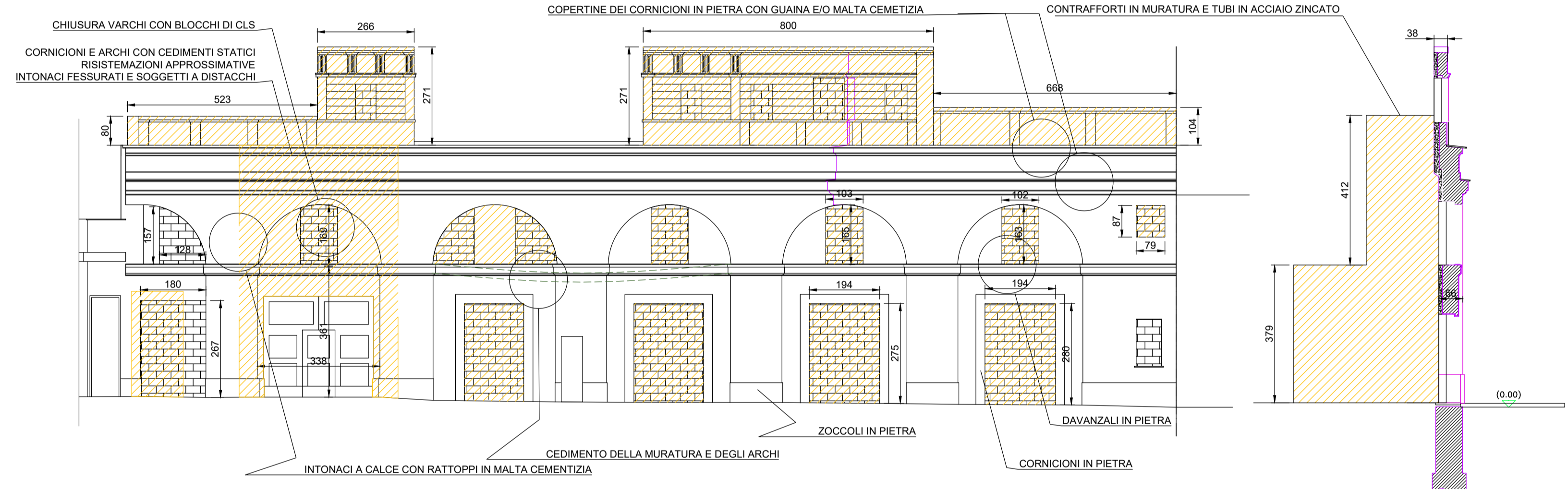
Particolare A: muratura da conservare su Piazza della Repubblica e contrafforti
