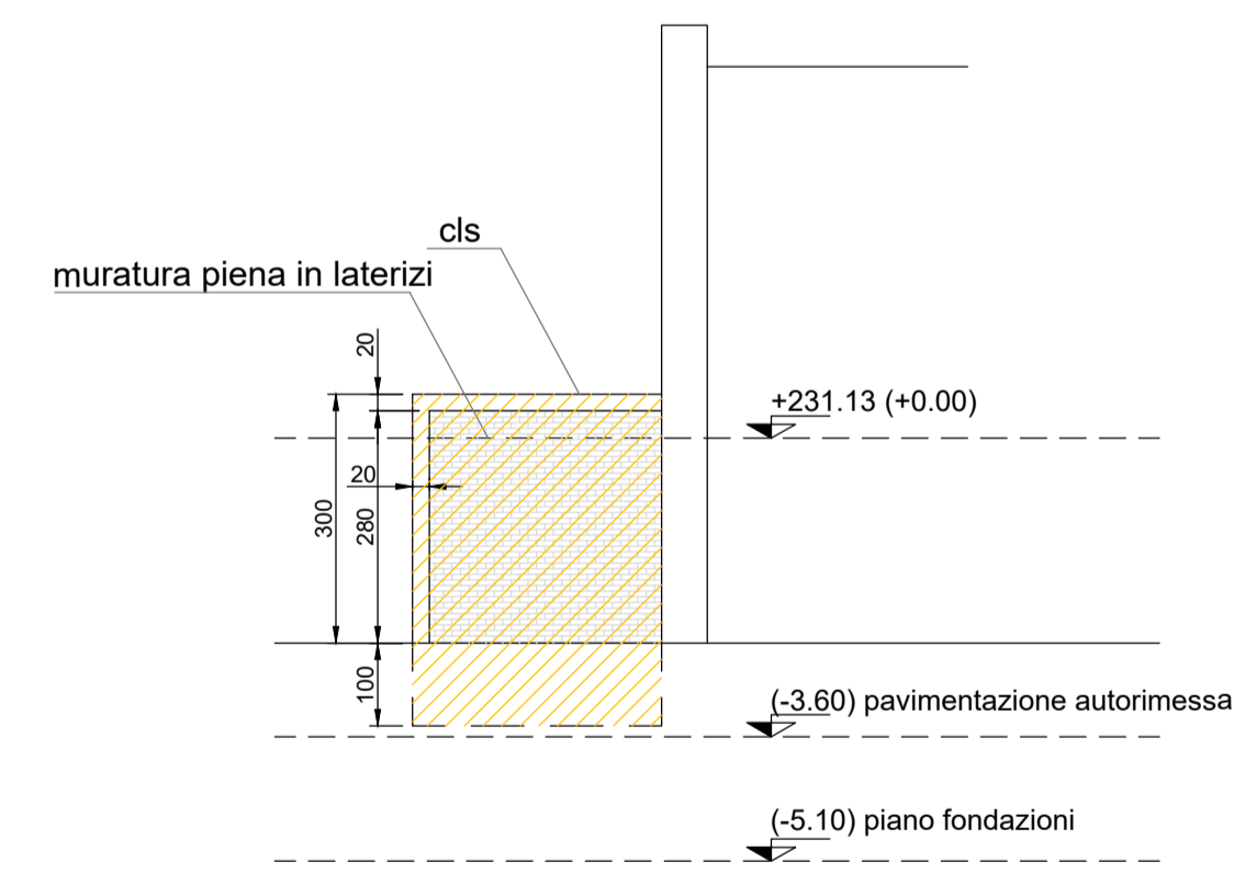
Particolare contrafforti C
