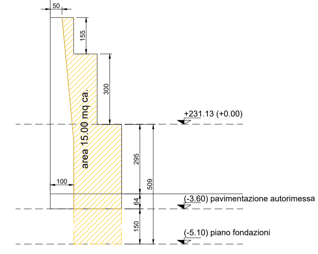
Particolare contrafforti B
