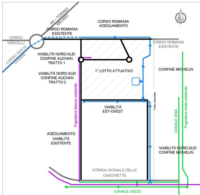
Figura 20: Schema della rete bianca in progetto – fase definitiva
