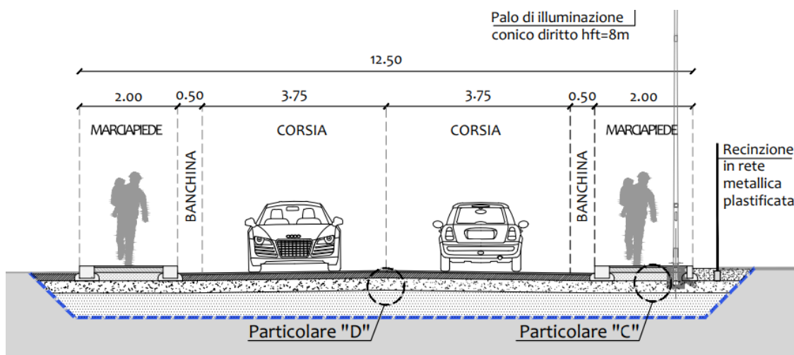
Figura 9 - sezione tipologica viabilità di confine sud
