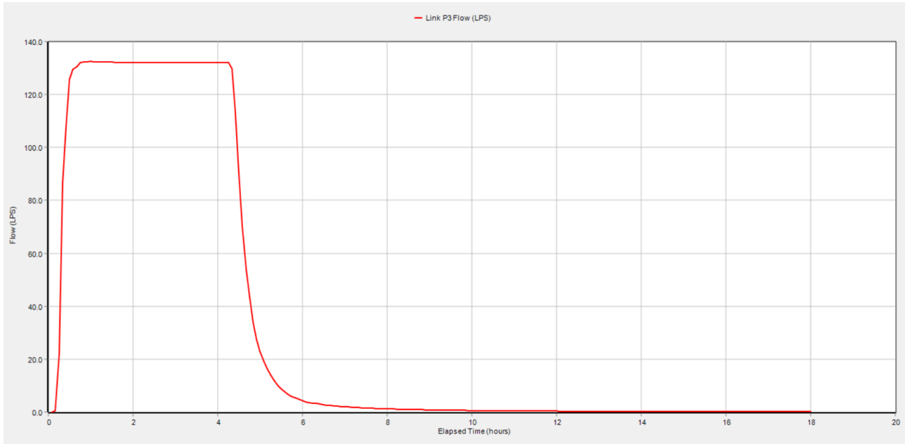
Figura 35: portata addotta al canale SNIA per evento intenso e di breve durata (picco a 10 minuti) TR50
