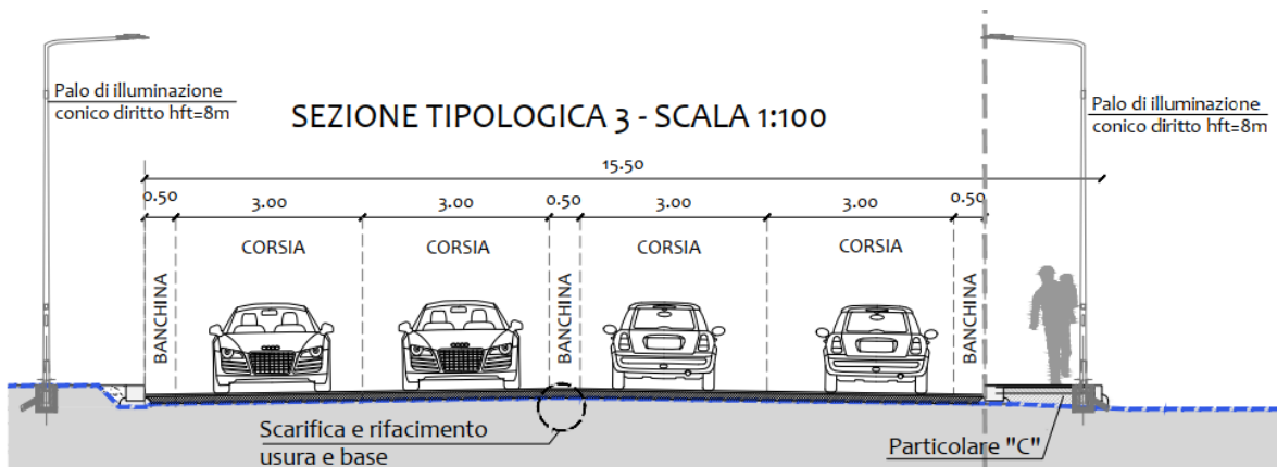
Figura 7 - sezione tipologica viabilità di confine ovest – tratto 1
