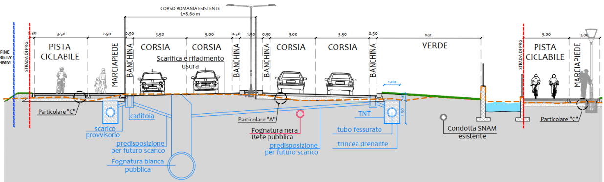
Figura 5a - sezione tipologica 1 adeguamento Corso Romania
