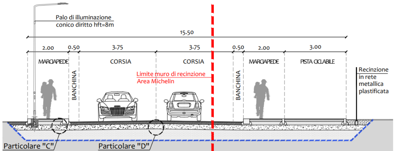
Figura 10 - sezione tipologica viabilità di confine est
