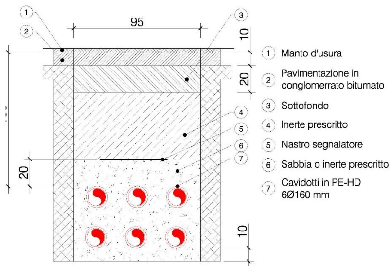
Figura 38 - sezione scavo tipo cavidotti MT
