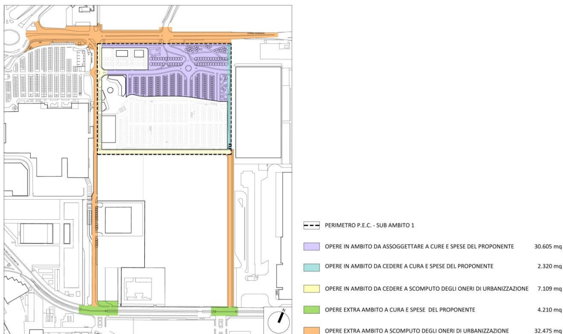
Figura 4a – Planimetria con la definizione della tipologia delle opere di urbanizzazione
