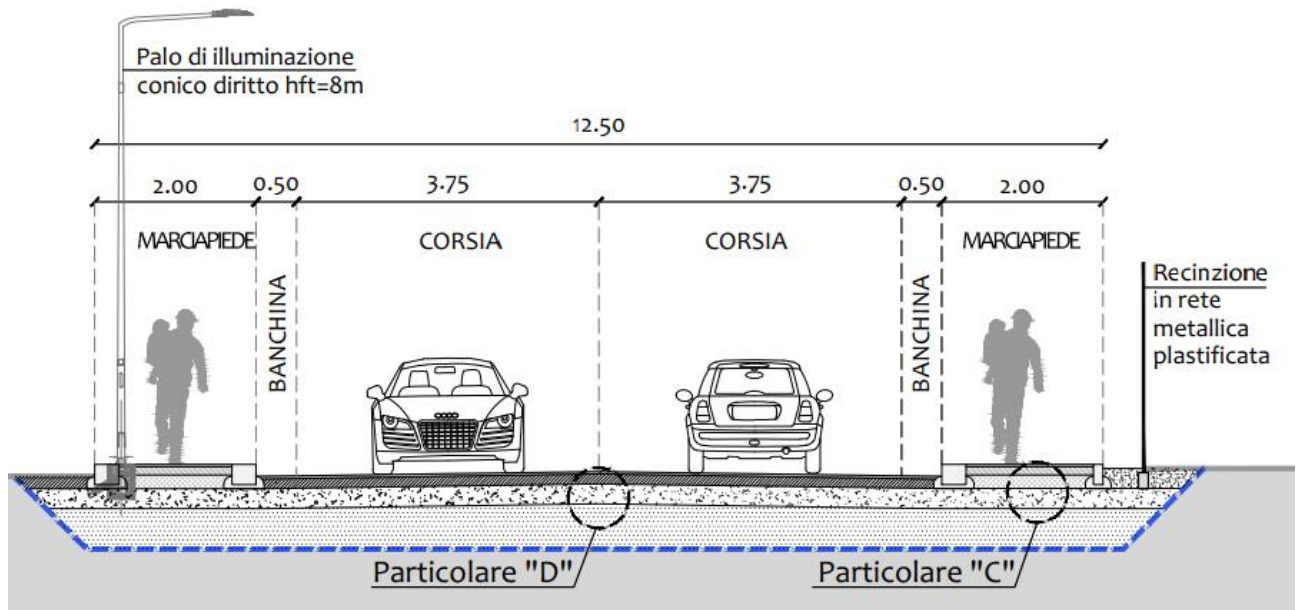
Figura 11 - sezione tipologica viabilità interne al lotto
