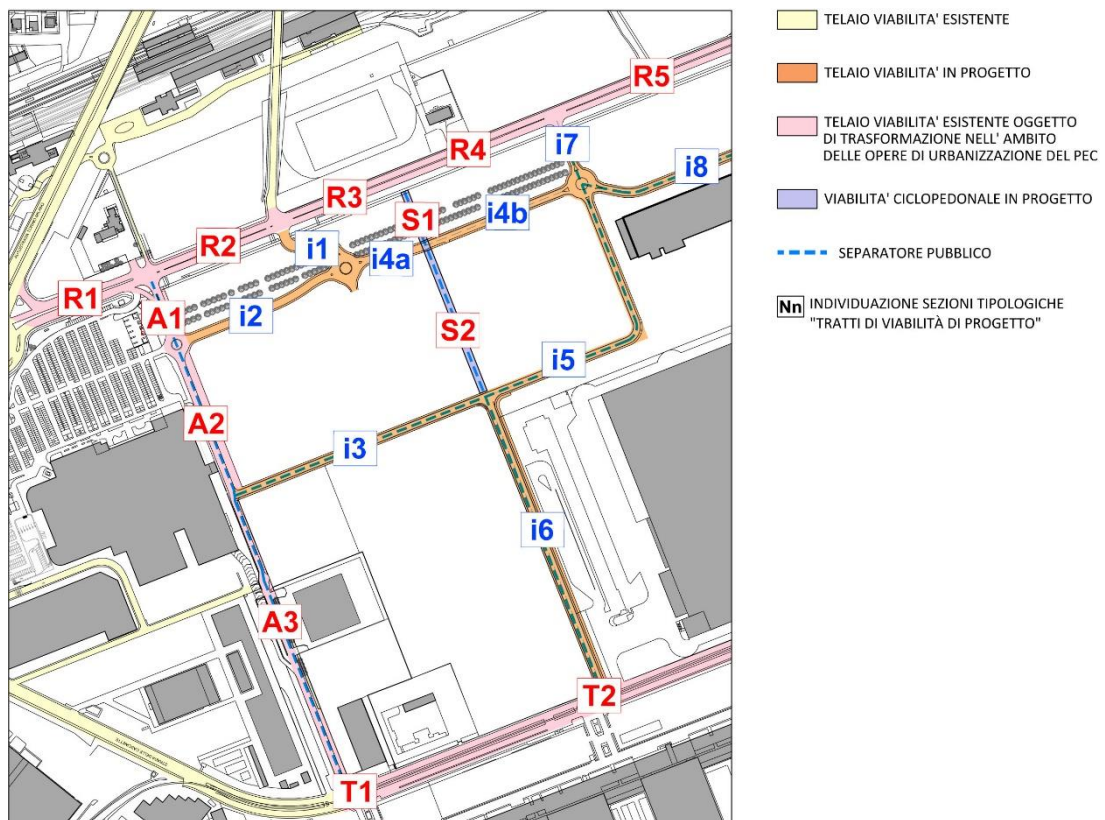
Figura 4c – Estratto Tav. 9 Masterplan "Telaio Viabilità"
