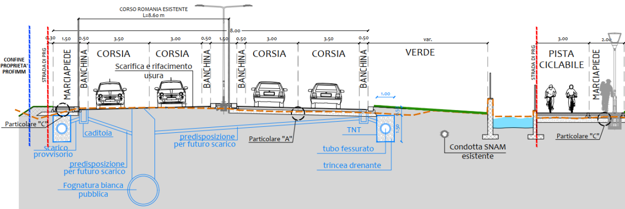
Figura 5b - sezione tipologica 2 adeguamento Corso Romania
