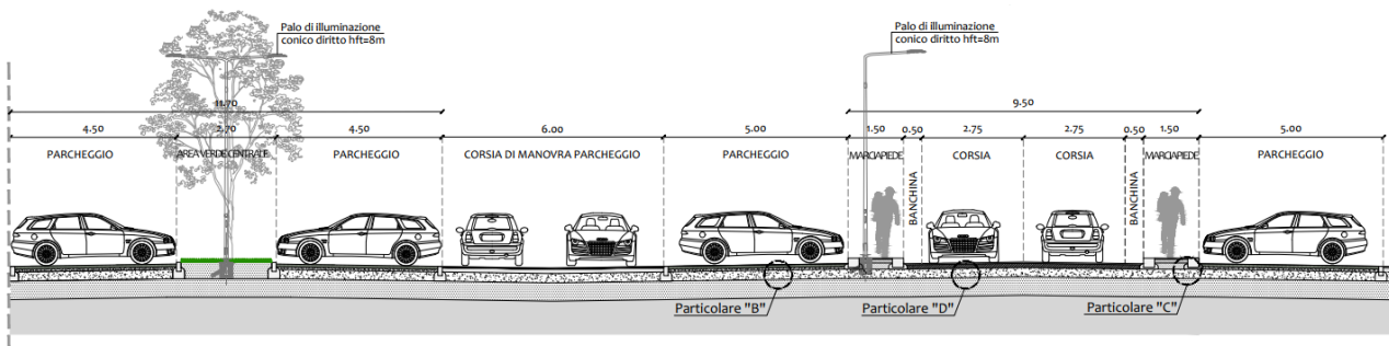
Figura 12 - sezione tipologica parcheggio
