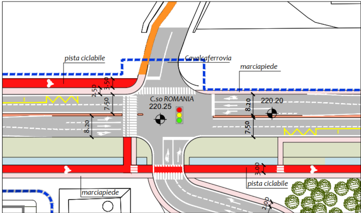
Figura 6 - esempio di incrocio semaforizzato su Corso Romania
