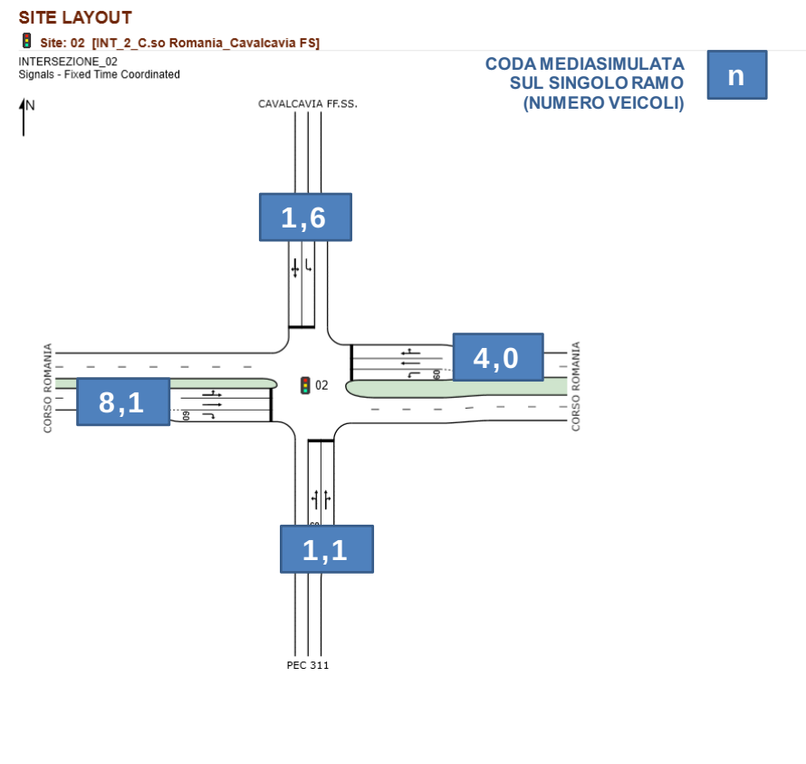
Figura 88 – Intersezione 2: Layout e lunghezza media simulata delle code (n° veicoli)
