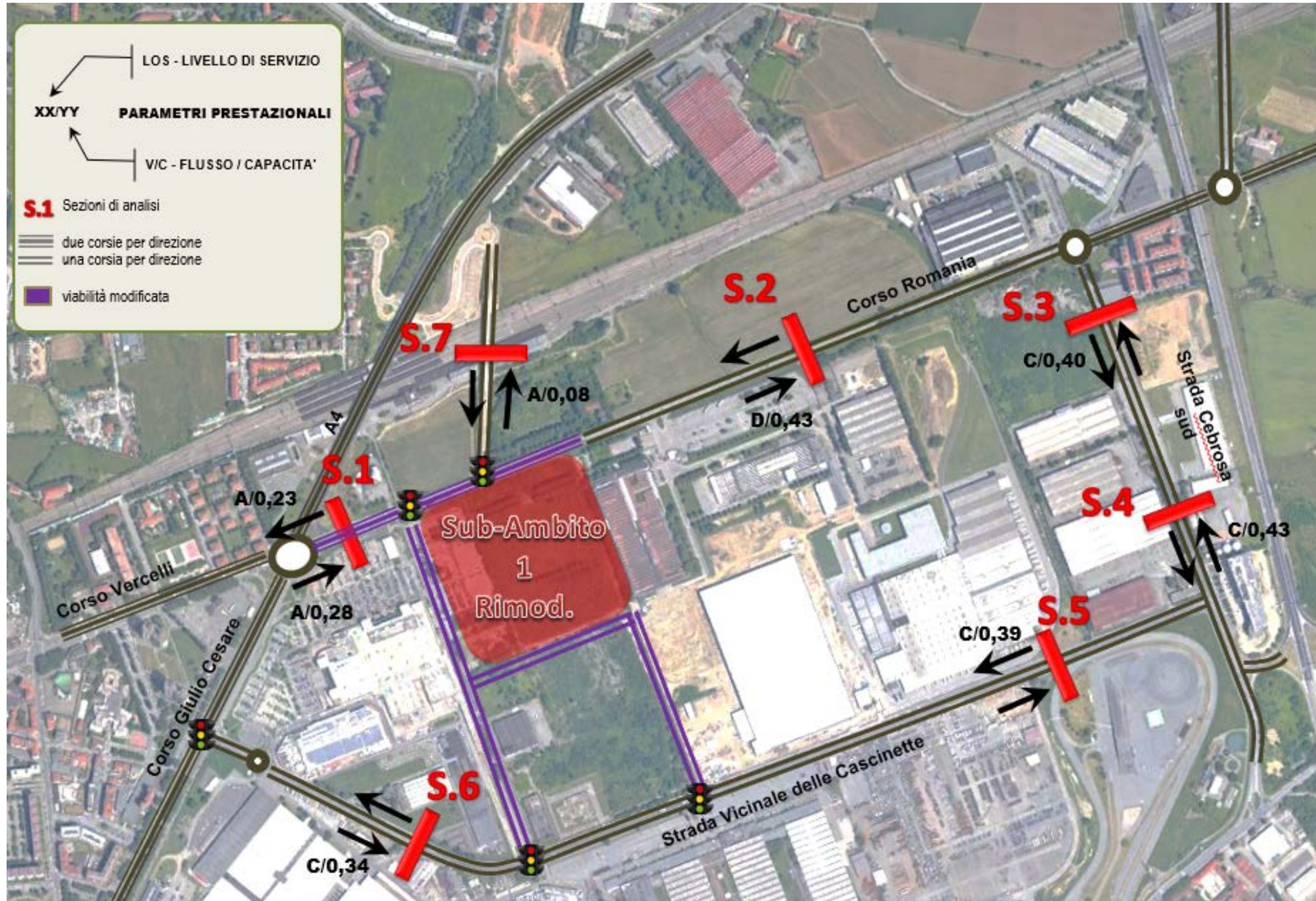
Figura 86 – Scenario 2: Livello di Servizio e rapporto VIC in sezione
