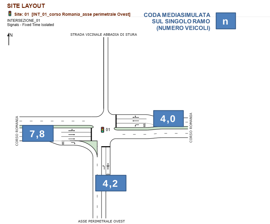
Figura 87 – Intersezione 1: Layout e lunghezza media simulata delle code (n° veicoli)
