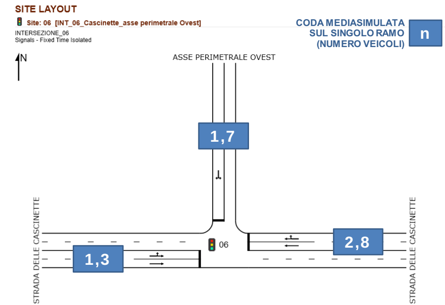
Figura 80 – Intersezione 6: Layout e lunghezza media simulata delle code (n° veicoli)
