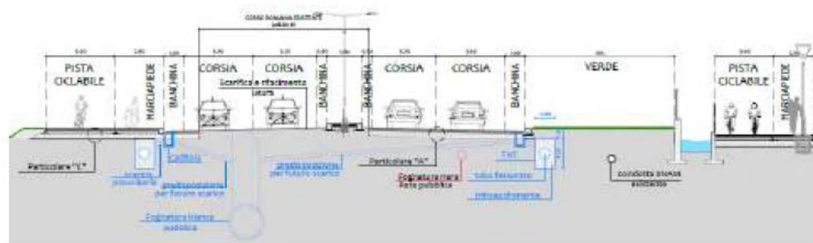
Figura 38 - Sezione nuova configurazione corso Romania Tratto 2
