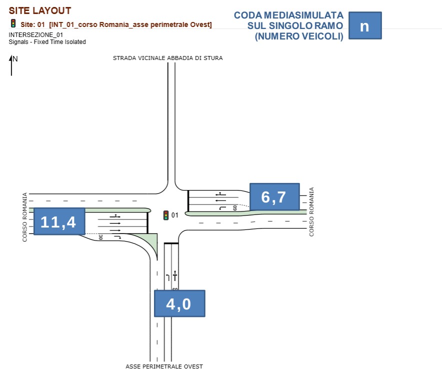
Figura 109 – Intersezione 1: Layout e lunghezza media simulata delle code (n° veicoli)
