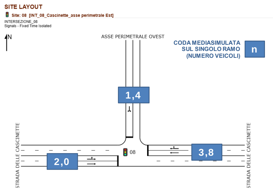
Figura 93 – Intersezione 8: Layout e lunghezza media simulata delle code (n° veicoli)
