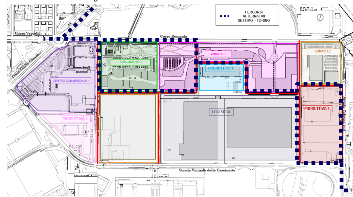
Figura 120 – Percorsi alternativi Torino – S.R. 11
