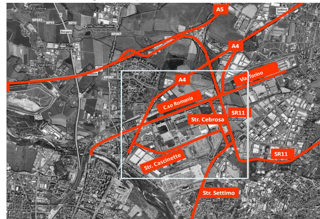
Figura 3 - Inquadramento Infrastrutturale
