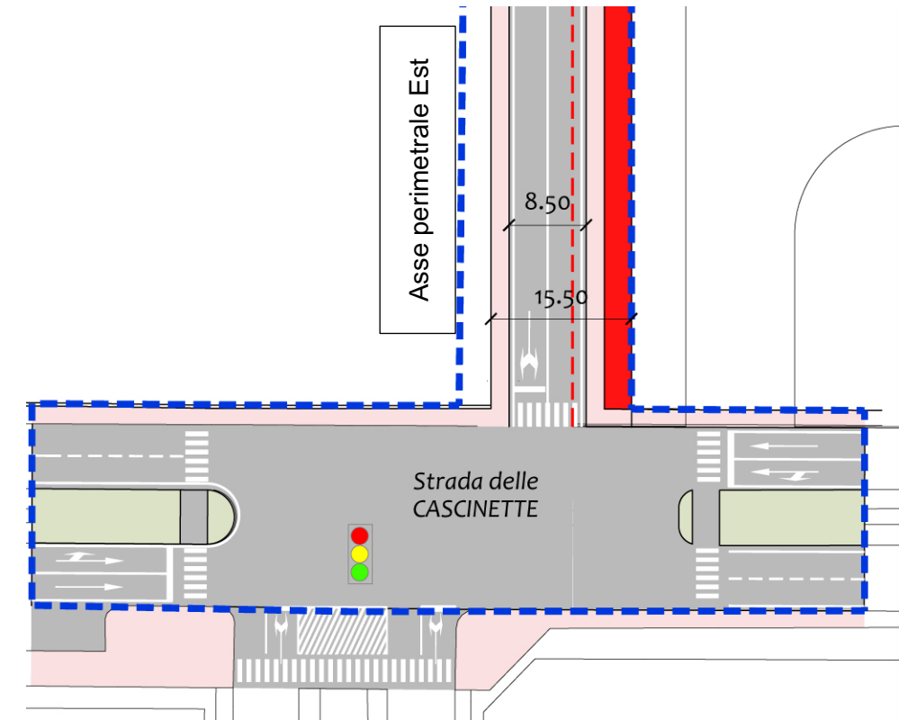
Figura 46 – Intersezione asse perimetrale Est – strada delle Cascinette
