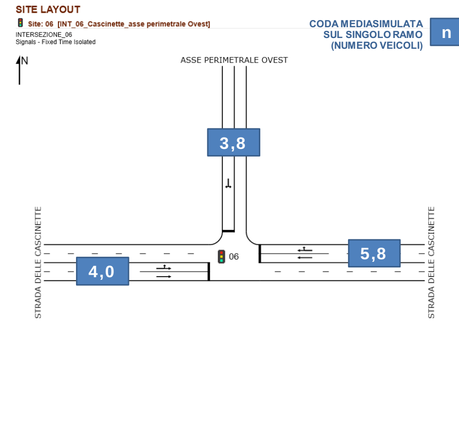
Figura 92 – Intersezione 6: Layout e lunghezza media simulata delle code (n° veicoli)
