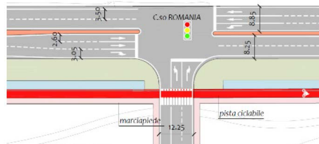
Figura 49 – Schema tipo intersezione semaforizzata
