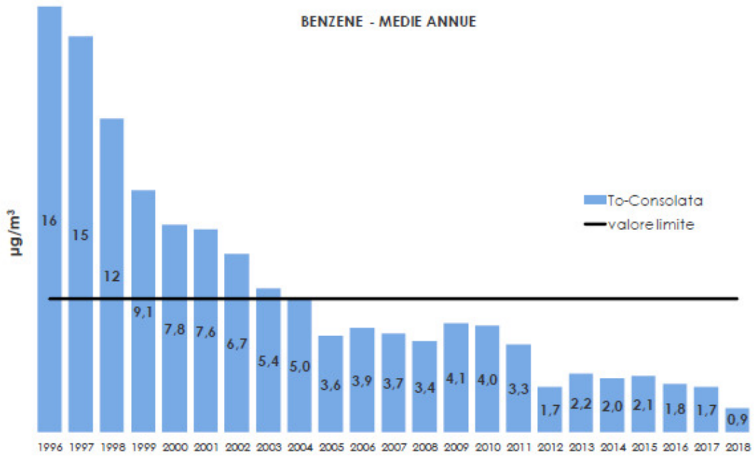
Figura 2-11 Benzene Concentrazione media annua
