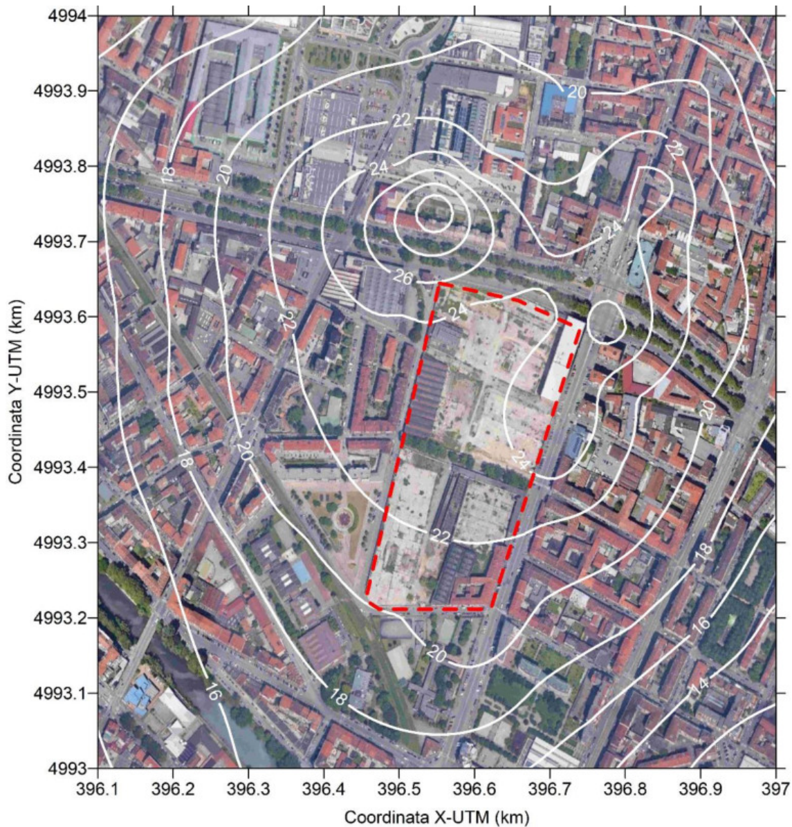
Figura 4-10: Scenario VARIANTE PRIN - Distribuzione spaziale del 99.8° percentile delle concentrazioni orarie di NO 2 (valori in \mu\text{g}/\text{m}^3 )
