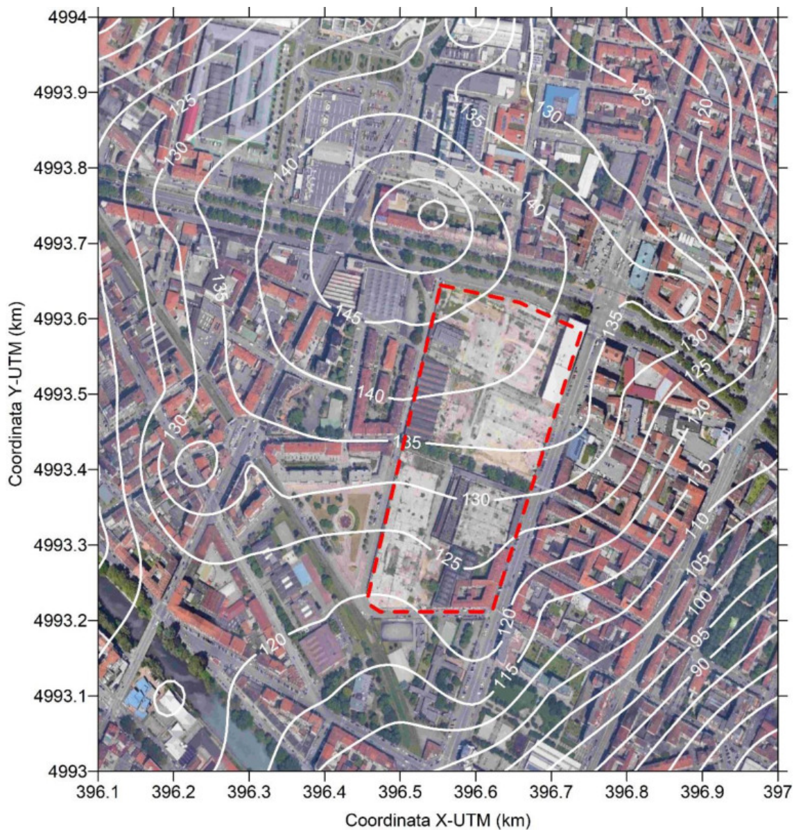
Figura 4-9: Scenario INT - Distribuzione spaziale del 99.8° percentile delle concentrazioni orarie di NO 2 (valori in µg/m 3 )
