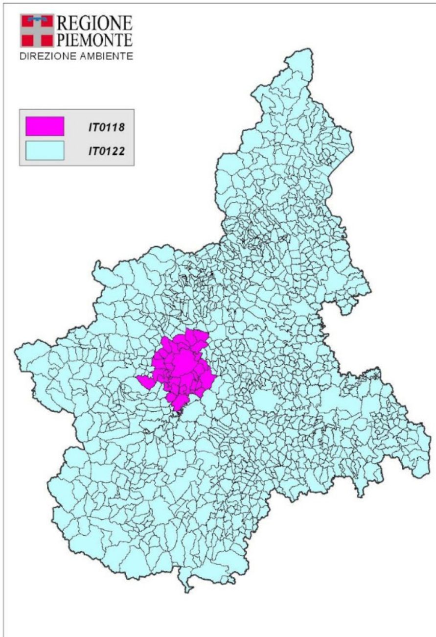
Figura 2-2 Rappresentazione grafica zonizzazione regionale per l'ozono
