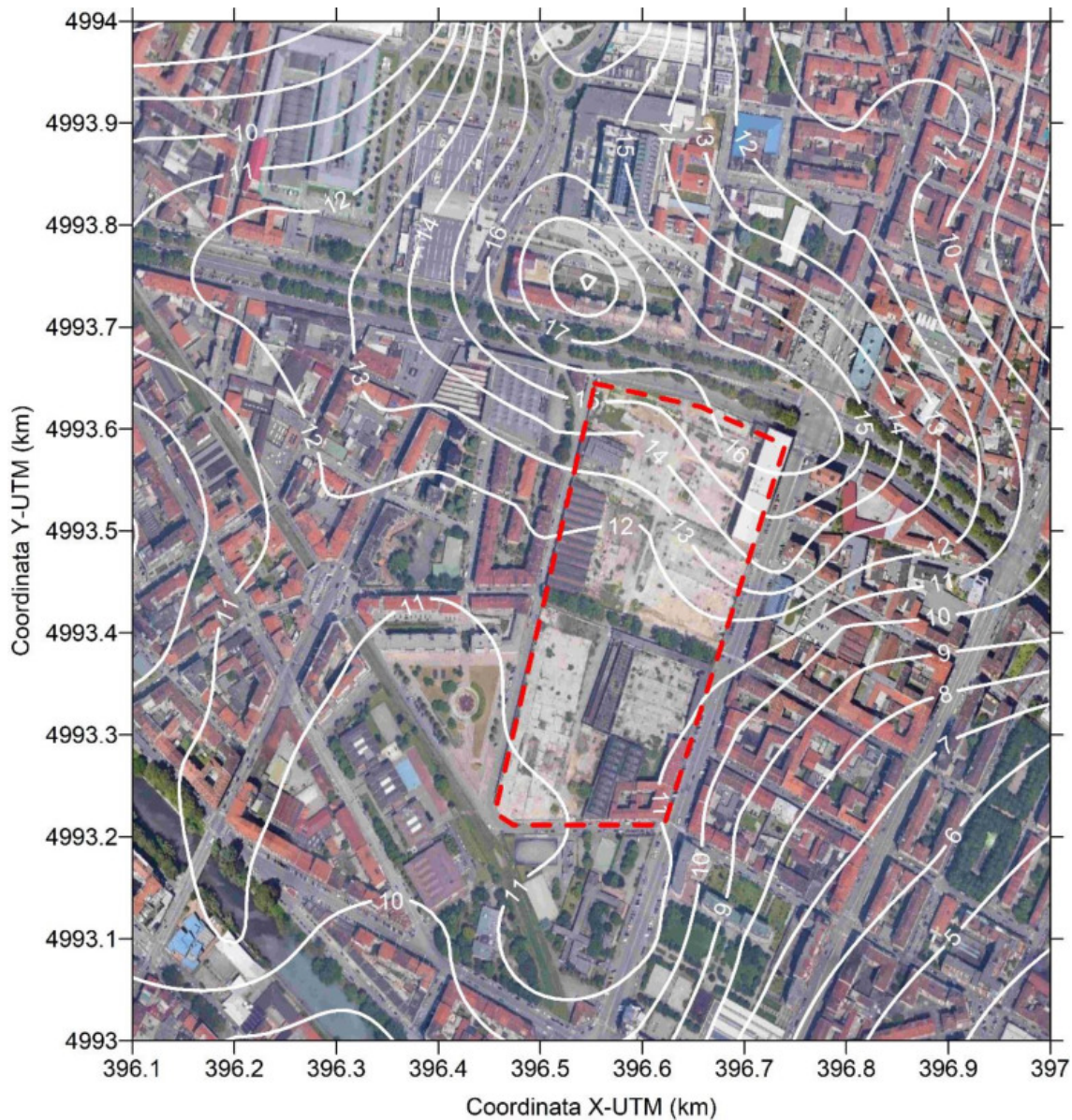
Figura 4-12: Scenario INT - Distribuzione spaziale delle concentrazioni medie annue di NO 2 (valori in µg/m 3 )
