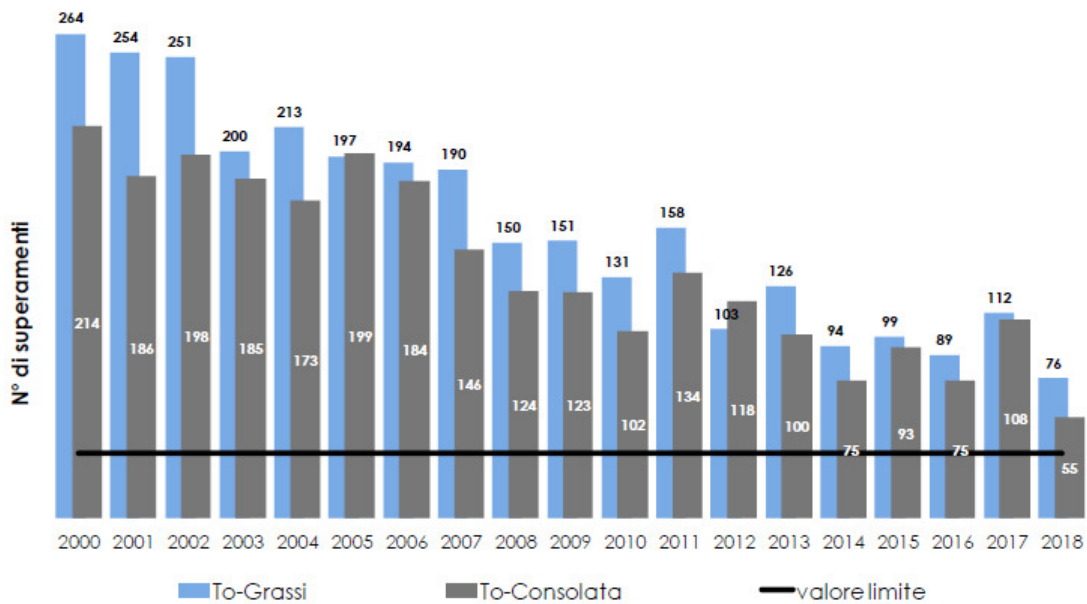
Figura 2-9 PM10 Numero di superamenti del valore limite giornaliero
