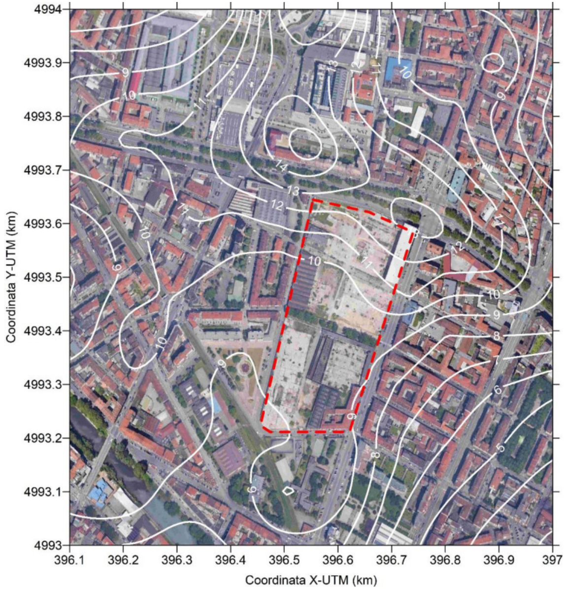
Figura 4-11: Scenario SDF - Distribuzione spaziale delle concentrazioni medie annue di NO 2 (valori in µg/m 3 )
