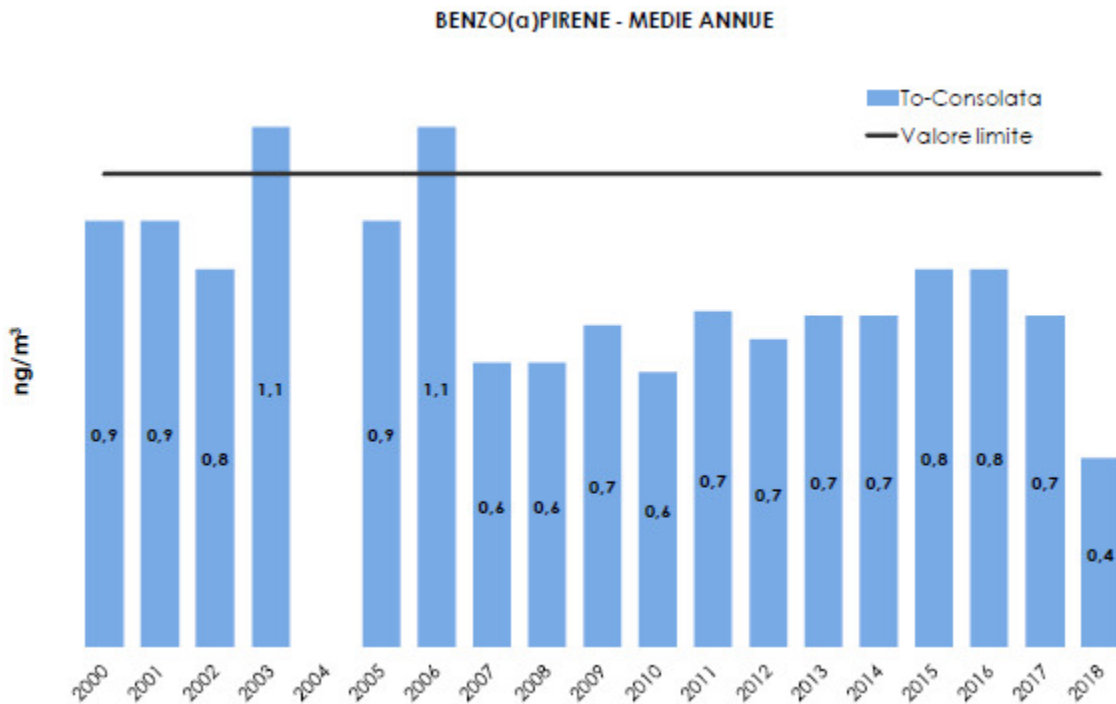
Figura 2-12 Benzo(a)pirene Concentrazione media annua
