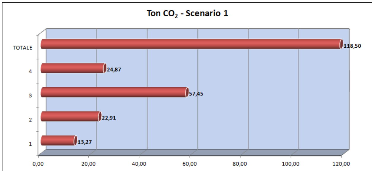
Figura 55: Grafico dei quantitativi di CO2 emessi per l'esecuzione delle attività dello Scenario 1
