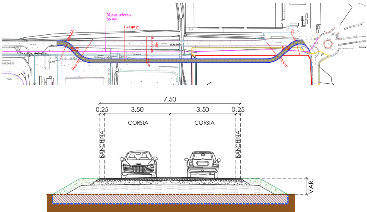
Figura 3 – planimetria e sezione tipologica "By-Pass"
