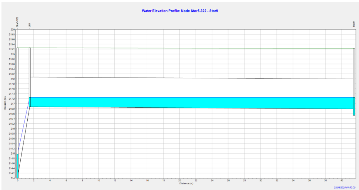
Figura 4: massimo riempimento delle condotte per evento intenso e di breve durata (picco a 10 minuti) TR50 anni
