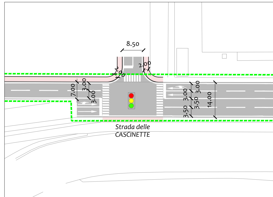
INCROCIO SEMAFORICO STRADA DELLE CASCINETTE - SCALA 1:750
