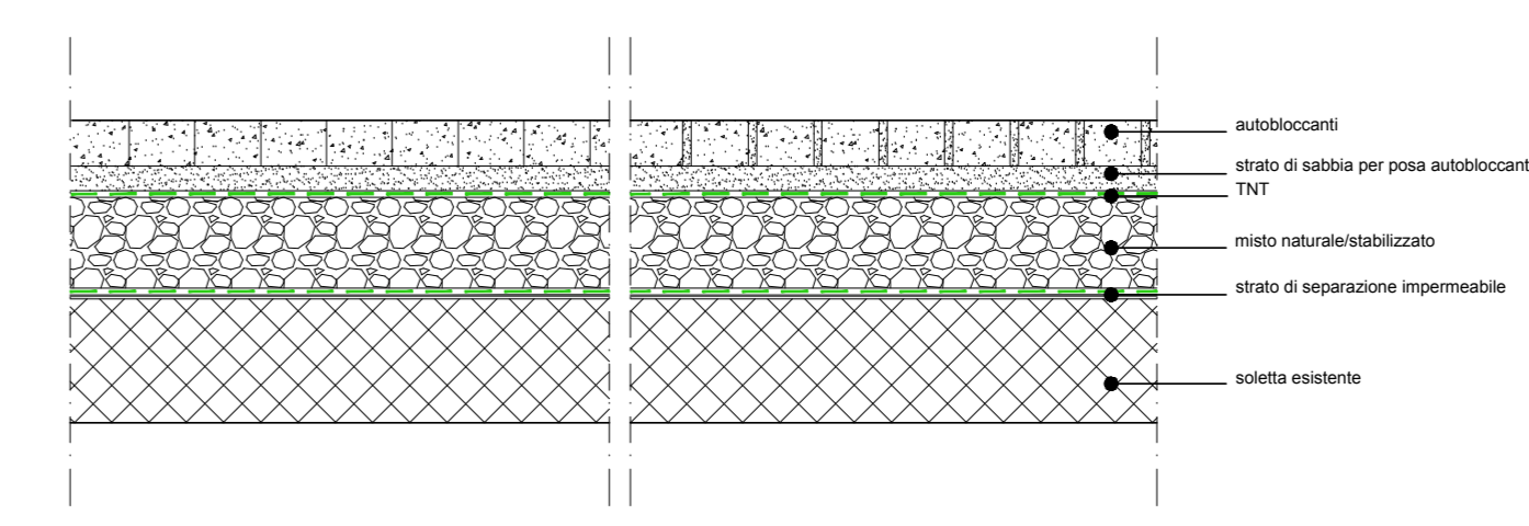
STRATIGRAFIA DI PROGETTO
