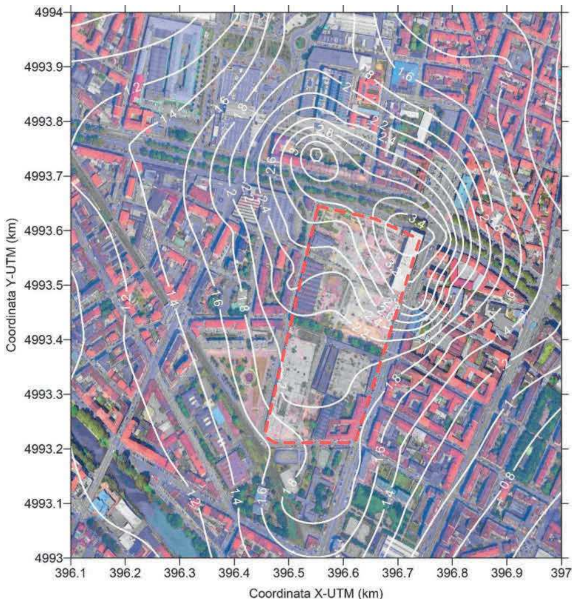
Figura 4-13: Scenario VARIANTE PRIN - Distribuzione spaziale delle concentrazioni medie annue di NO2 (valori in µg/m³)
