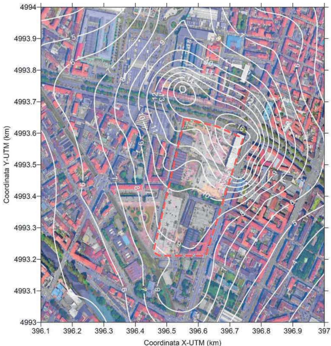
Figura 4-19: Scenario VARIANTE PRIN - Distribuzione spaziale delle concentrazioni medie annue di CO (valori in µg/m³)
