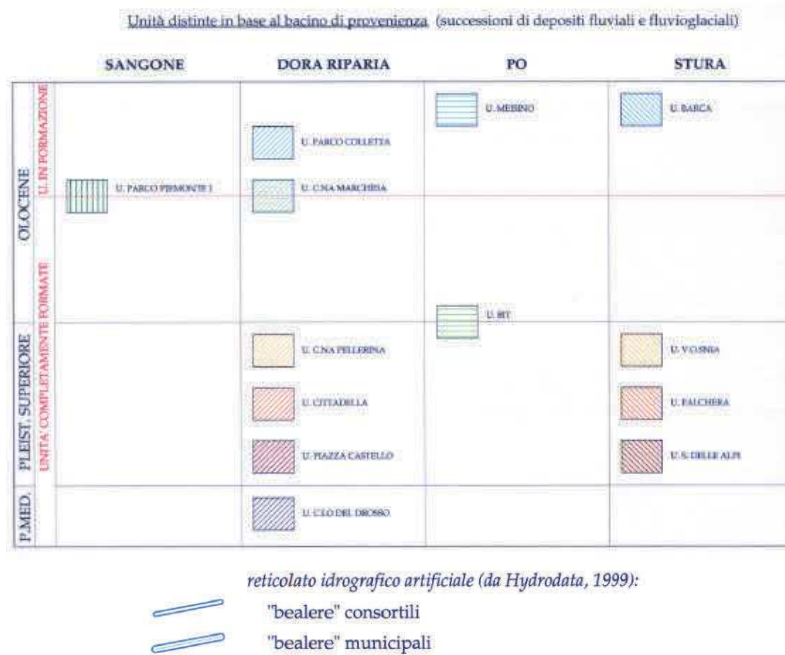
Figura c - Stralcio della Carta Geologico-strutturale e Geomorfologica del PRG del Comune di Torino
