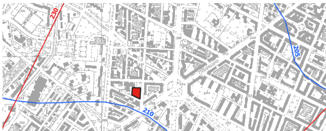
Figura 2.10 Estratto di C.T.R. con indicazione delle linee isopiezometriche (rosso) e delle linee della base dell'acquifero superficiale (blu – D.D. 900 del 03/12/2012)
