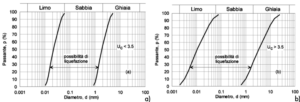
Fig. 7.11.1 NTC 2018 – Fusi granulometrici di terreni suscettibili di liquefazione
