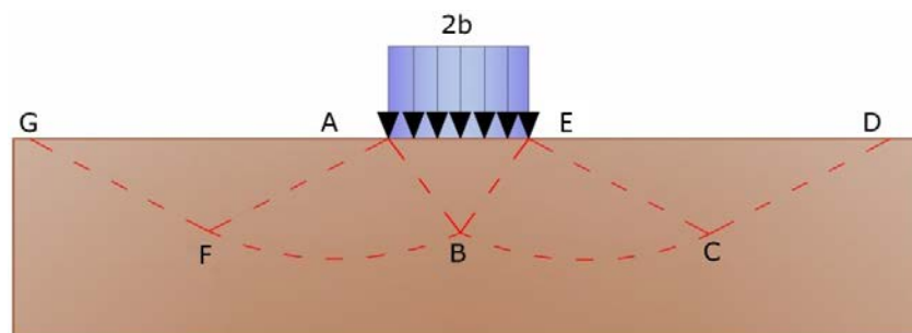
Meccanismo di rottura di Prandtl
