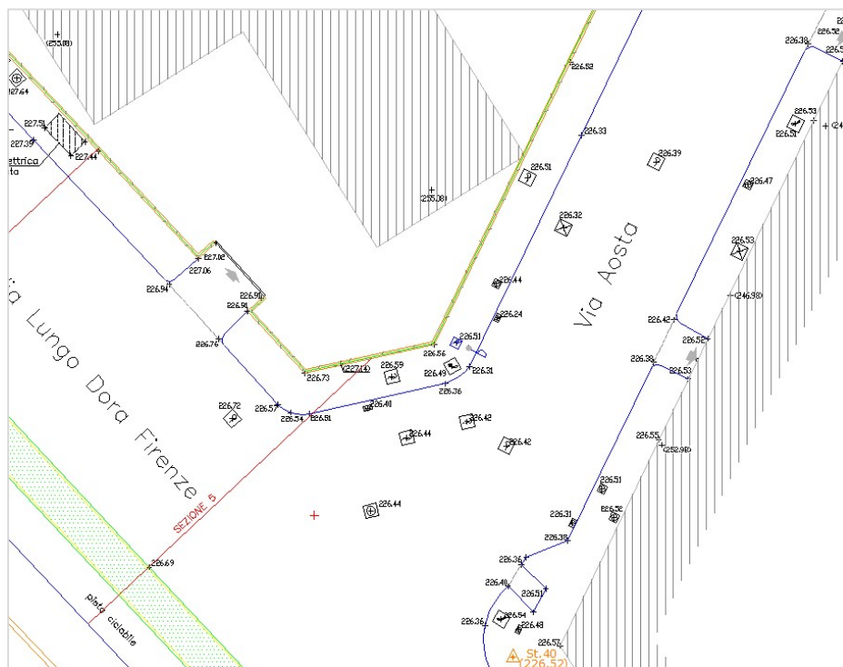
Figura 5.5: Rilievo area di intervento Stato di Fatto – ingrandimento area potenzialmente critica idraulicamente
