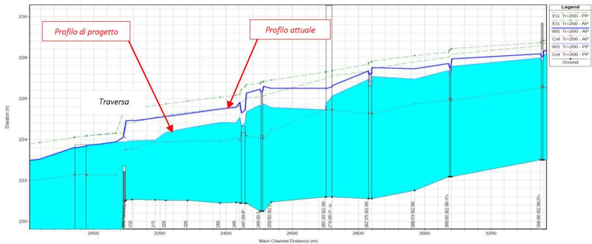
Figura 4.15: Confronto tra modello prima e dopo traversa – Tr 200 anni (630 mc/s)
