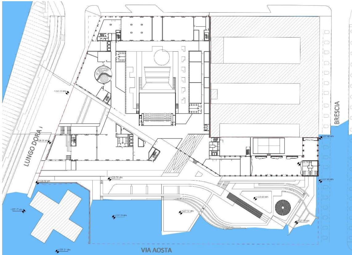
Figura 5.11: planimetria di progetto e in blu aree aventi elevazione inferiore a 227,50 m s.l.m.
