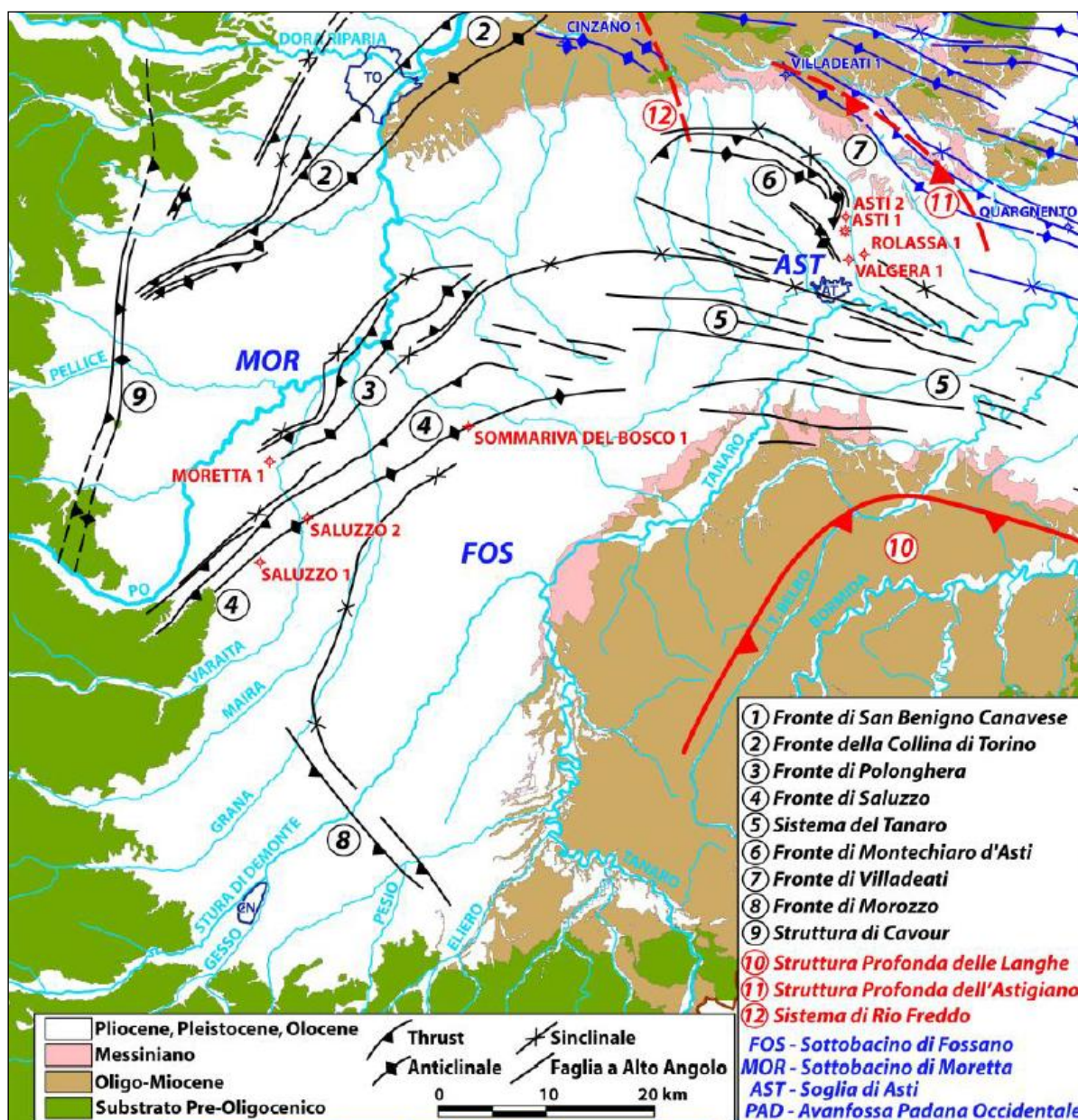
Figura 11 – Lineamenti strutturali e sottobacini del Bacino di Savigliano. La mappa è basata sul rilievo sismico 2D Eni (Ghielmi et al., 2019).
