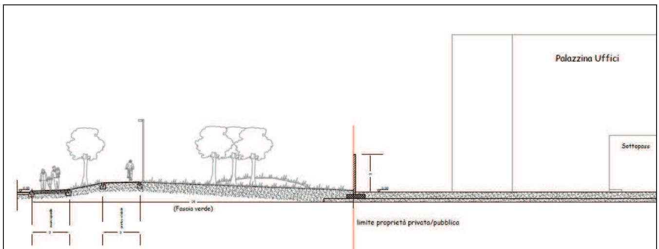
Figura 3: Stralcio della Tavola "Allegato 2" della Proposta di Modifica al Permesso di Costruire Convenzionato del 9 luglio 2010 - maggio 2014 – Sezione della fascia verde lungo il fronte di via Anselmetti
