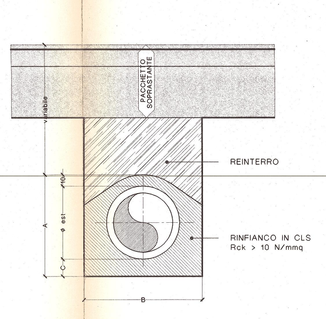
PARTICOLARE COSTRUTTIVO TUBAZIONE FOGNATURA BIANCA SCALA 1:20
