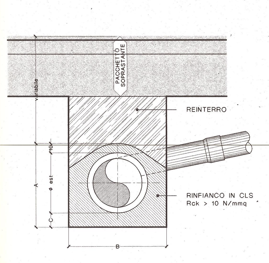
PARTICOLARE COSTRUTTIVO TUBAZIONE FOGNATURA BIANCA - ALLACCIAMENTO SCALA 1:20
