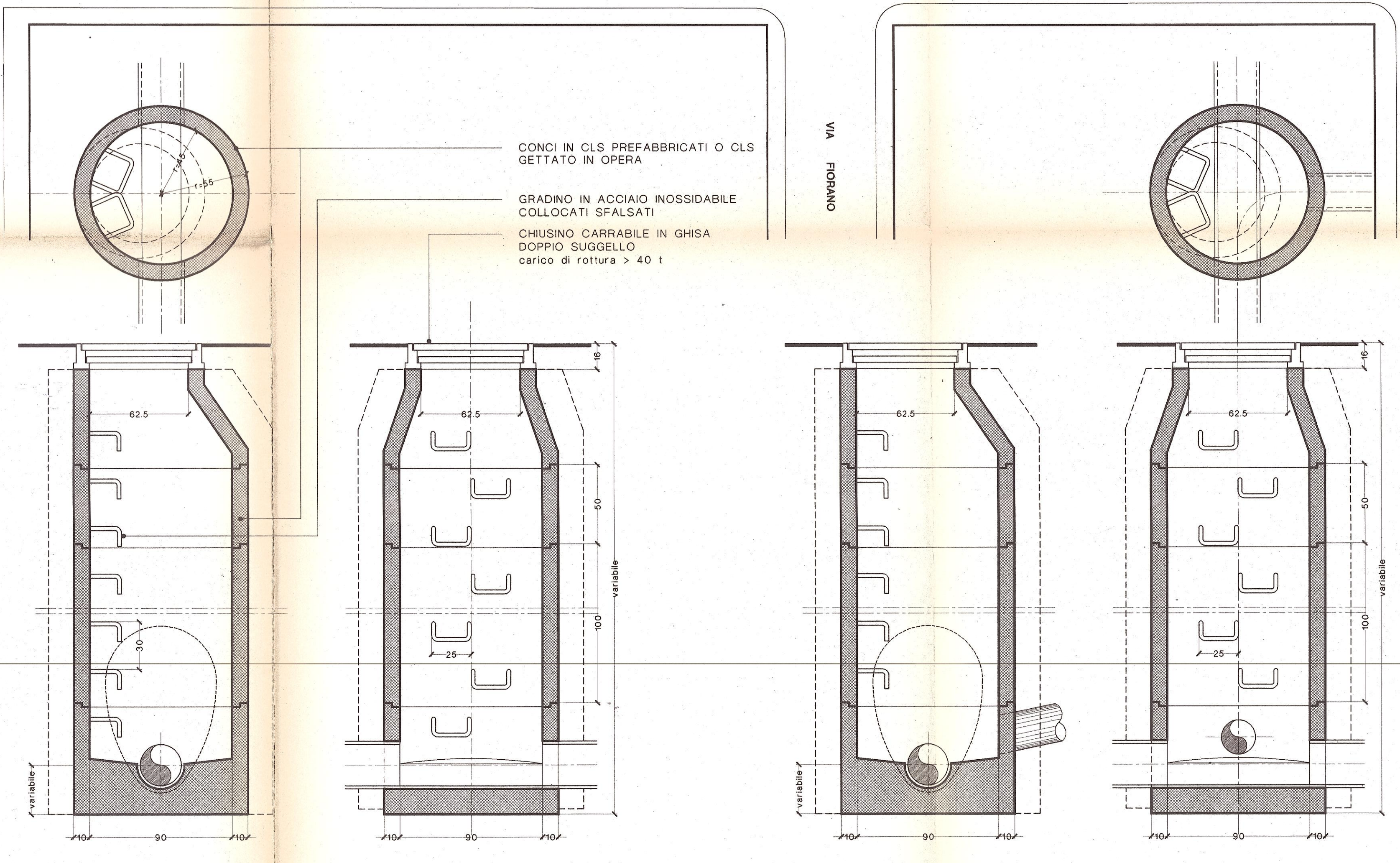
PARTICOLARE POZZETTO D'ISPEZIONE FOGNATURA BIANCA SCALA 1:20
