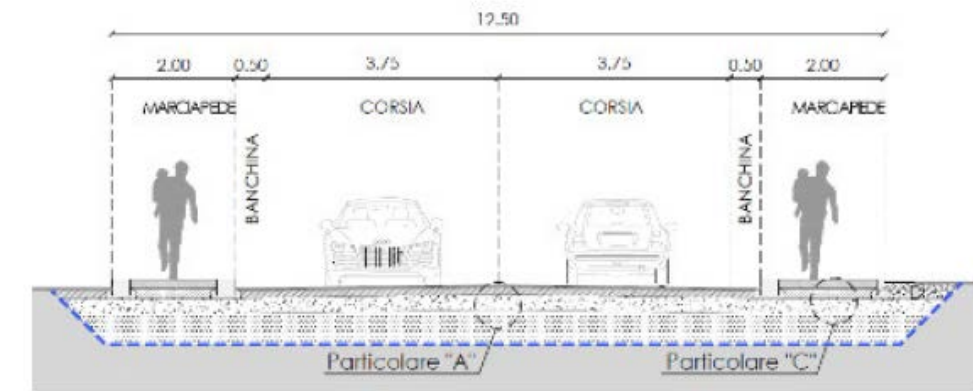
Figura 70 – Schema tipo intersezione semaforizzata corso Romania
