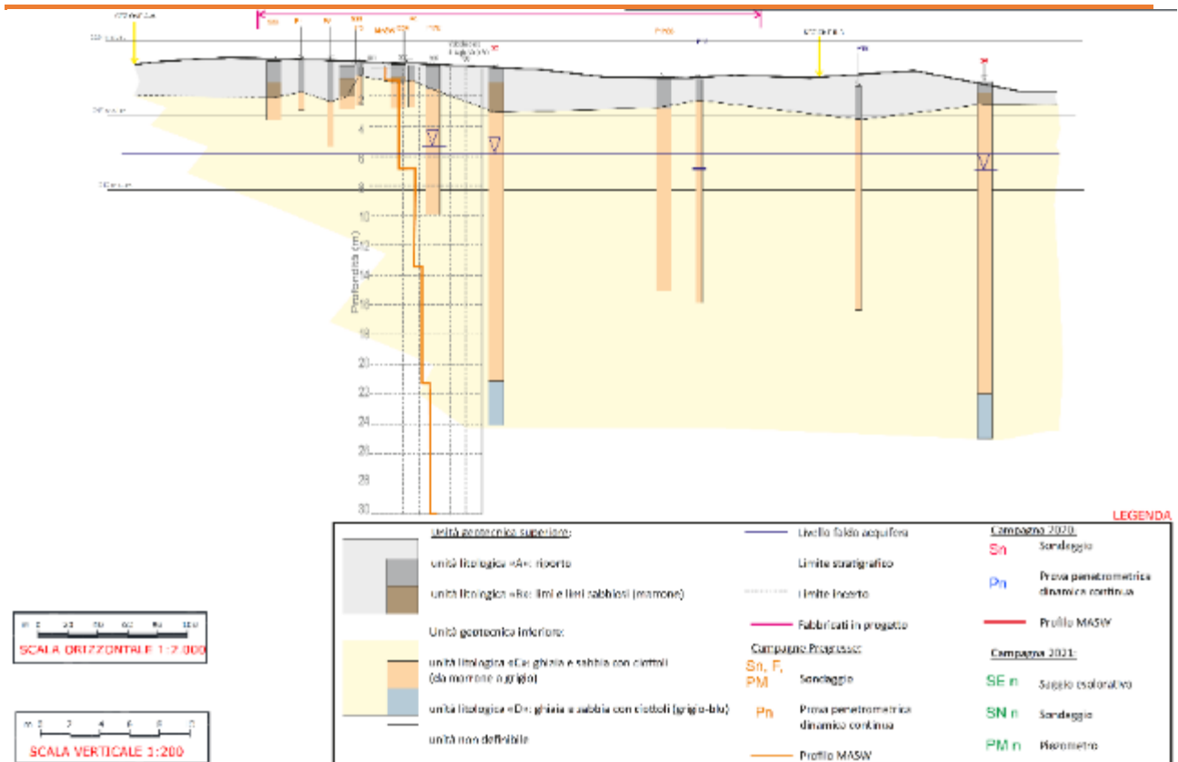
Figura 11: Sezione stratigrafica CC
