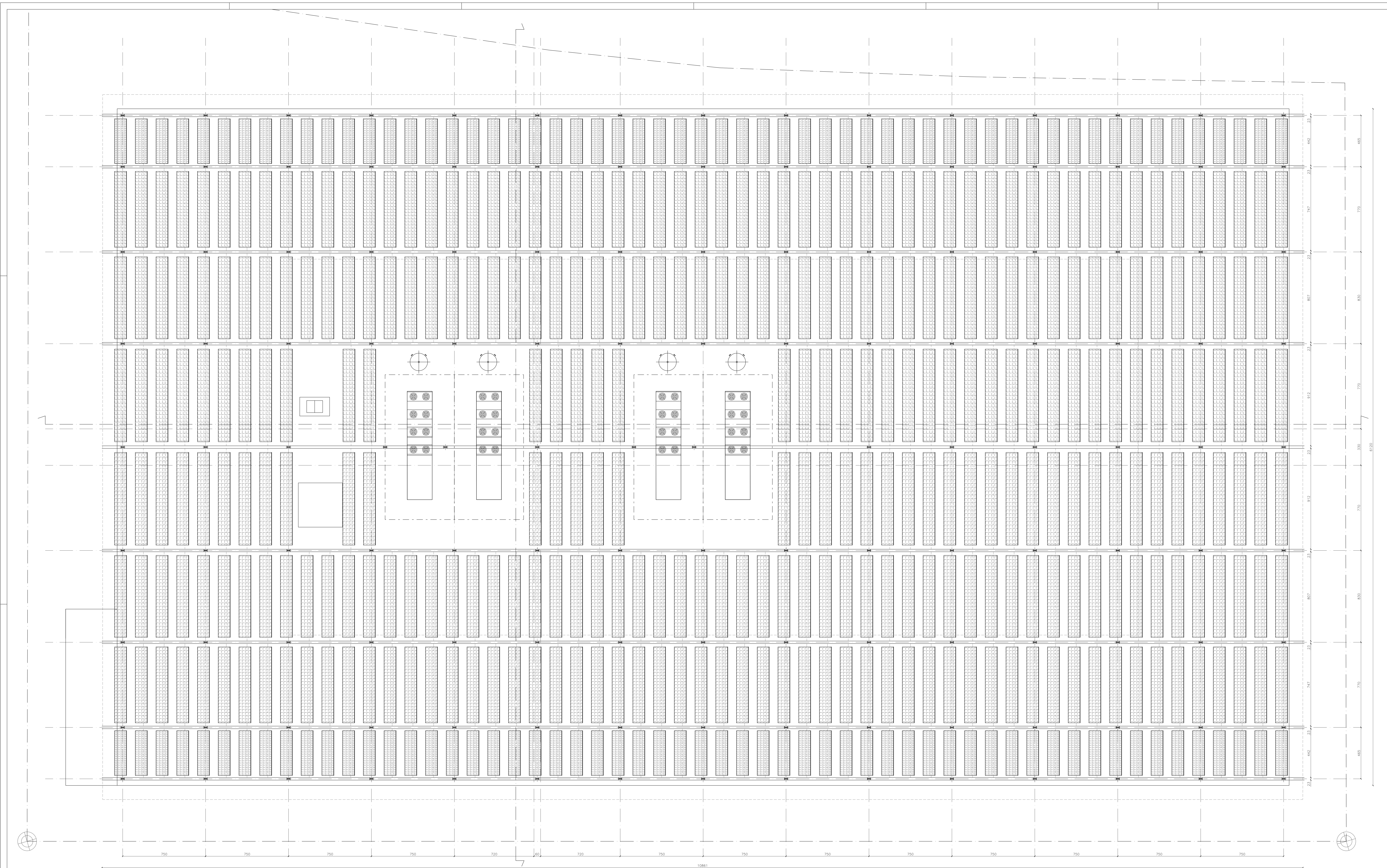
PIANTA COPERTURA
