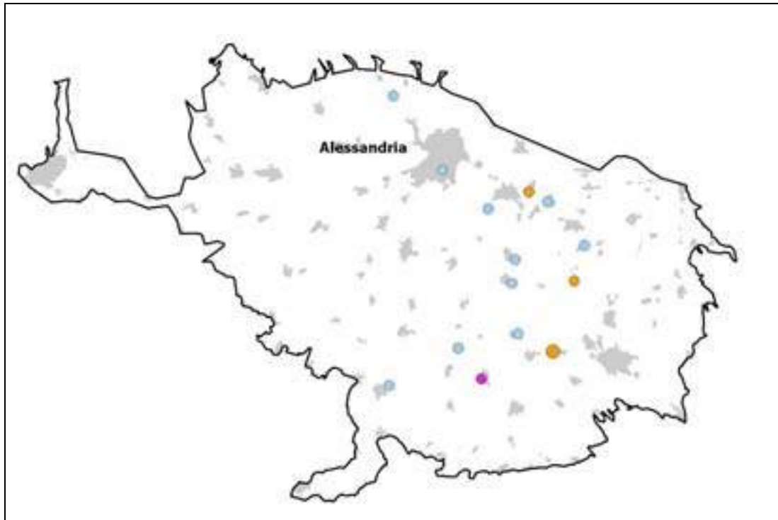
Figura 7.4.4 - Impatto puntuale VOC nel triennio 2012-2014 in GWB-P4
