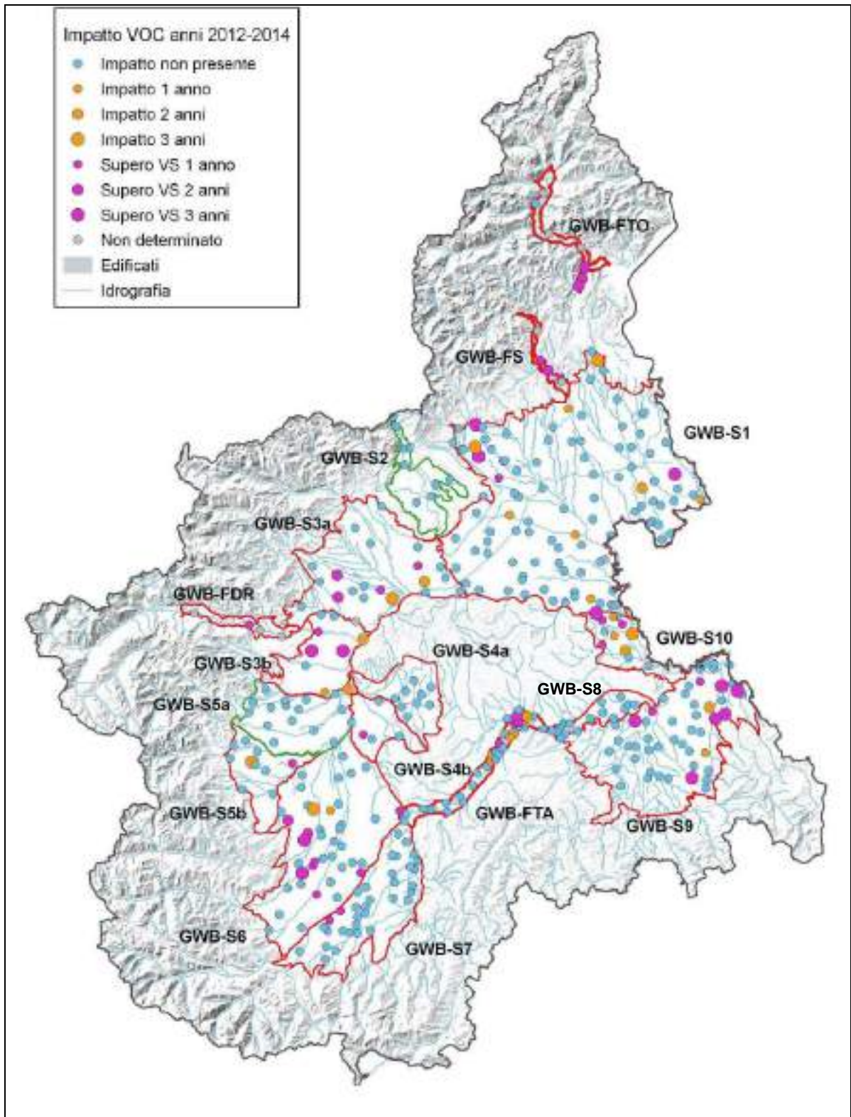
Figura 4.1 - Impatto puntuale VOC e SC triennio 2012-2014 acquifero superficiale
