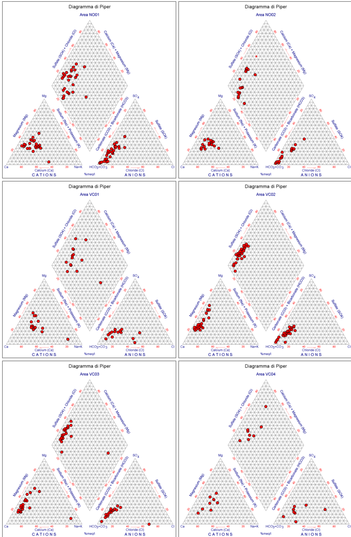
Figura 4.27: Diagrammi di Piper delle Aree Idrogeologiche che compongono il GWB-S1
