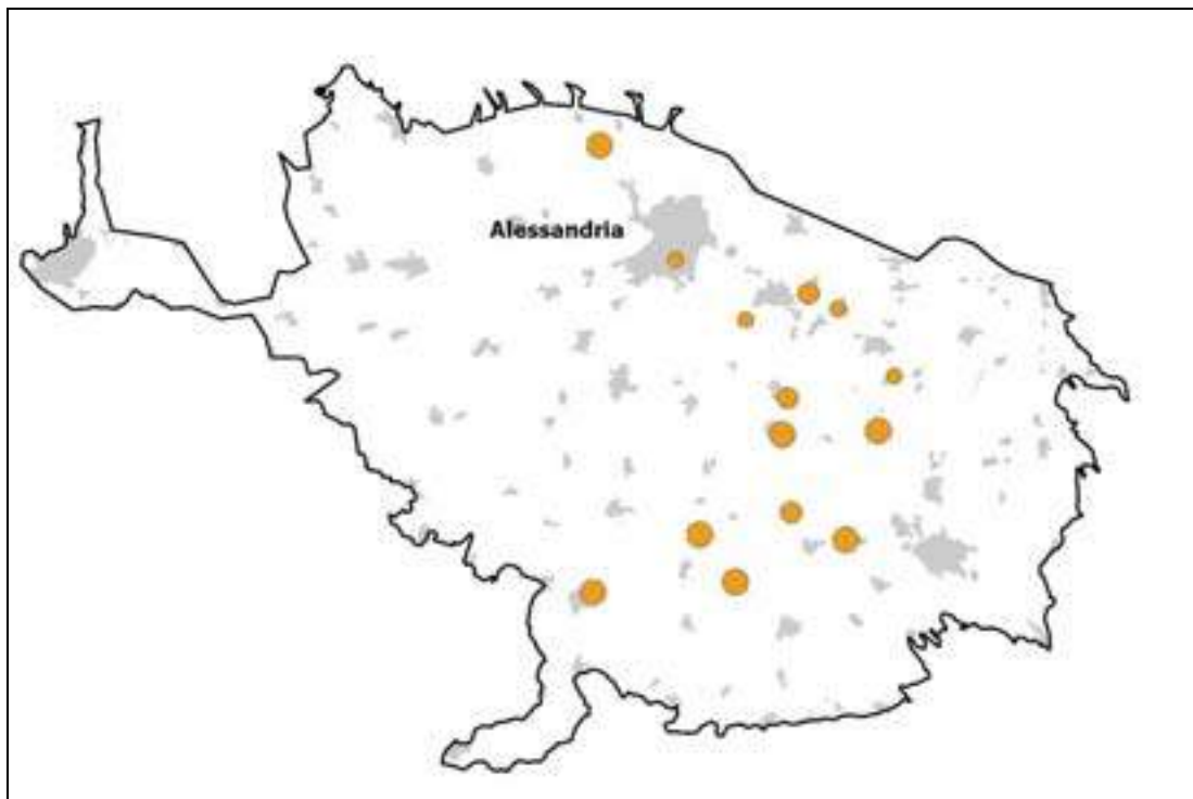
Figura 7.4.5 - Impatto puntuale Nichel nel triennio 2012-2014 in GWB-P4
