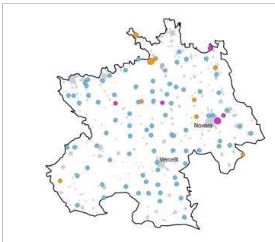
Figura 7.1.3 - Impatto puntuale dei VOC negli anni 2012-2014 in GWB-P1
