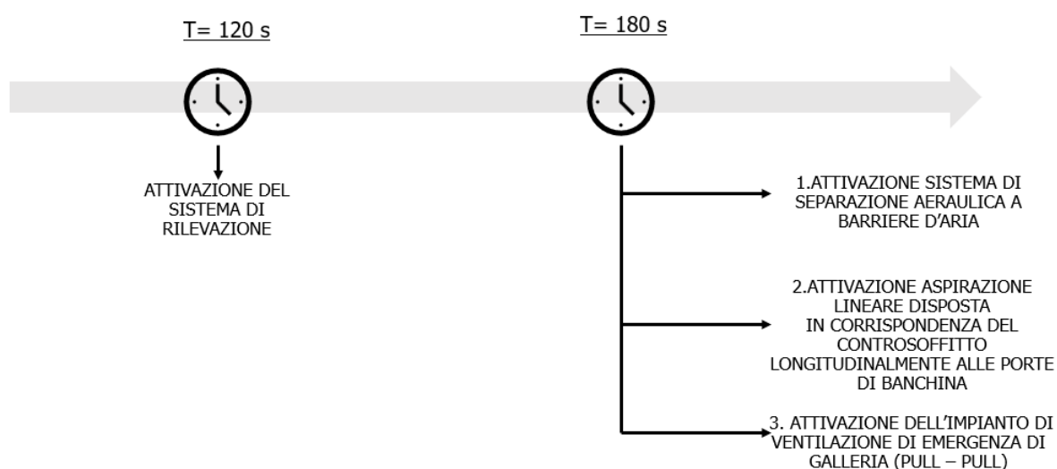
Figura 2 - Timing attivazione ventilazione Impianti e Sistemi (SCENARIO 1)
