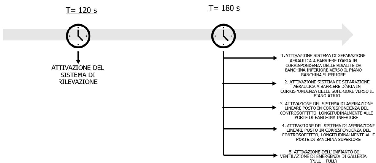
Figura 5. Timing attivazione ventilazione impianti e sistemi
