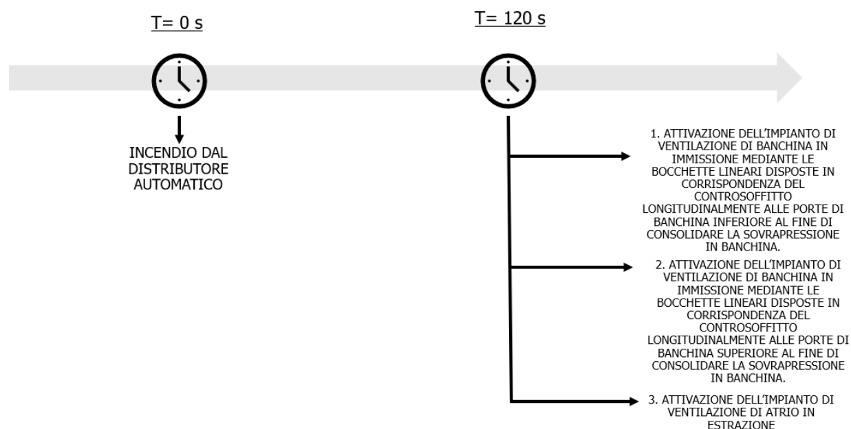
Figura 11 – Timing Attivazione ventilazione - Impianti e Sistemi
