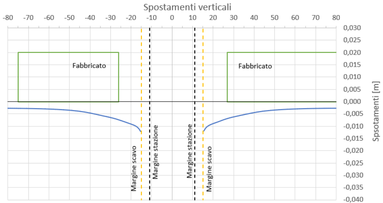
Figura 11. Spostamenti verticali
