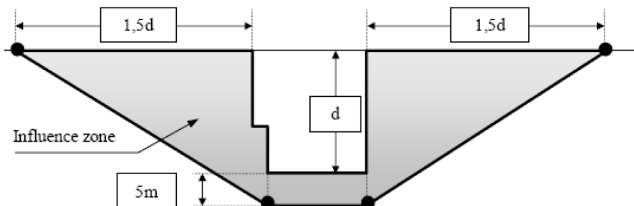
Figura 5. Zona di influenza minima per scavi in C&C
