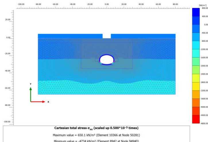
Figura 17. Sezione Galleria Banchina: s_{xx} , a fase 8
