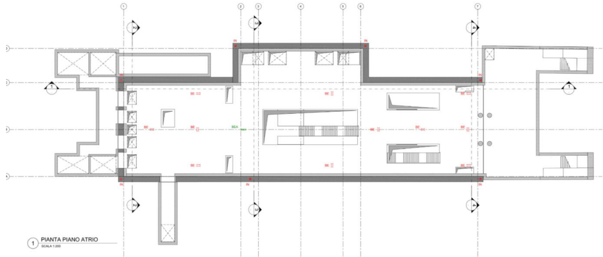
Figura 25. Schema di monitoraggio (MTL2T1A2DPRCSMOT001) – Planimetria. Per le rimanenti sezioni, vedasi la tavola di riferimento
