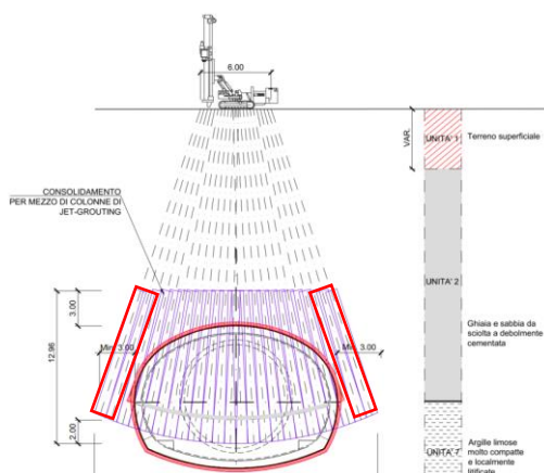
Consolidamento previsto per lo scavo delle gallerie di linea (MTL2T1A2DSTRSMOT002.2)
