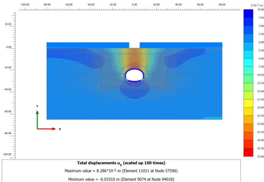
Figura 19. Sezione Galleria Banchina: Spostamenti verticali u_y a fase 8
