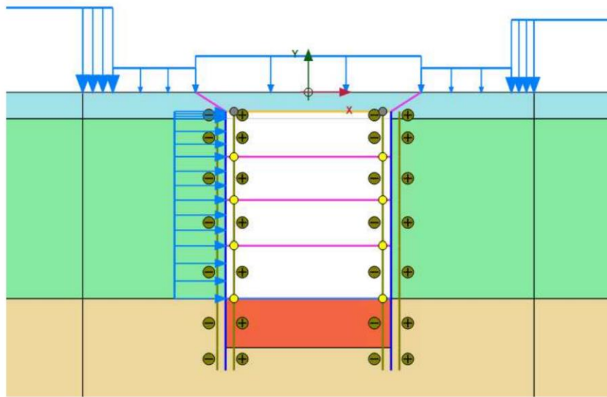
Figura 4. Modello geometrico corpo stazione (Cut&Cover)
