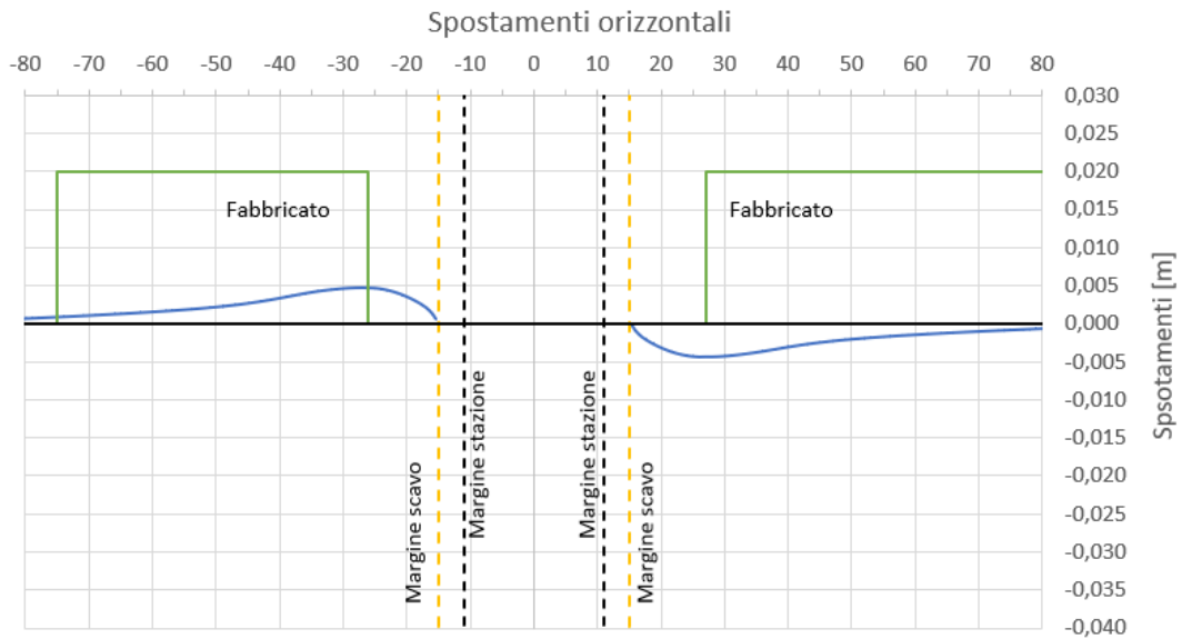
Figura 12. Spostamenti orizzontali
