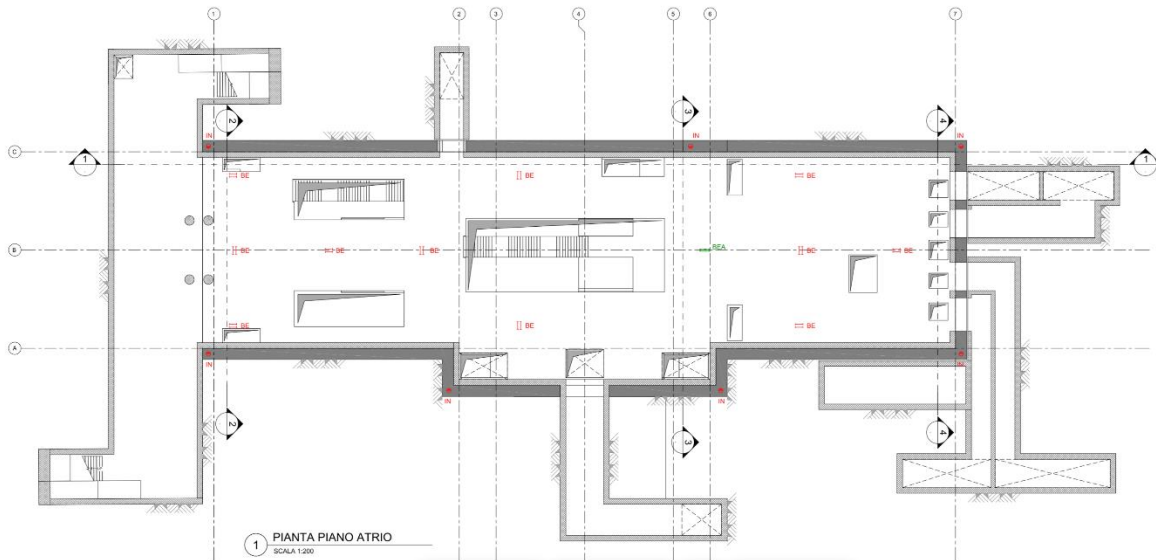
Figura 25. Schema di monitoraggio (MTL2T1A2DPRCSNOT001) – Planimetria. Per le rimanenti sezioni, vedasi la tavola di riferimento
