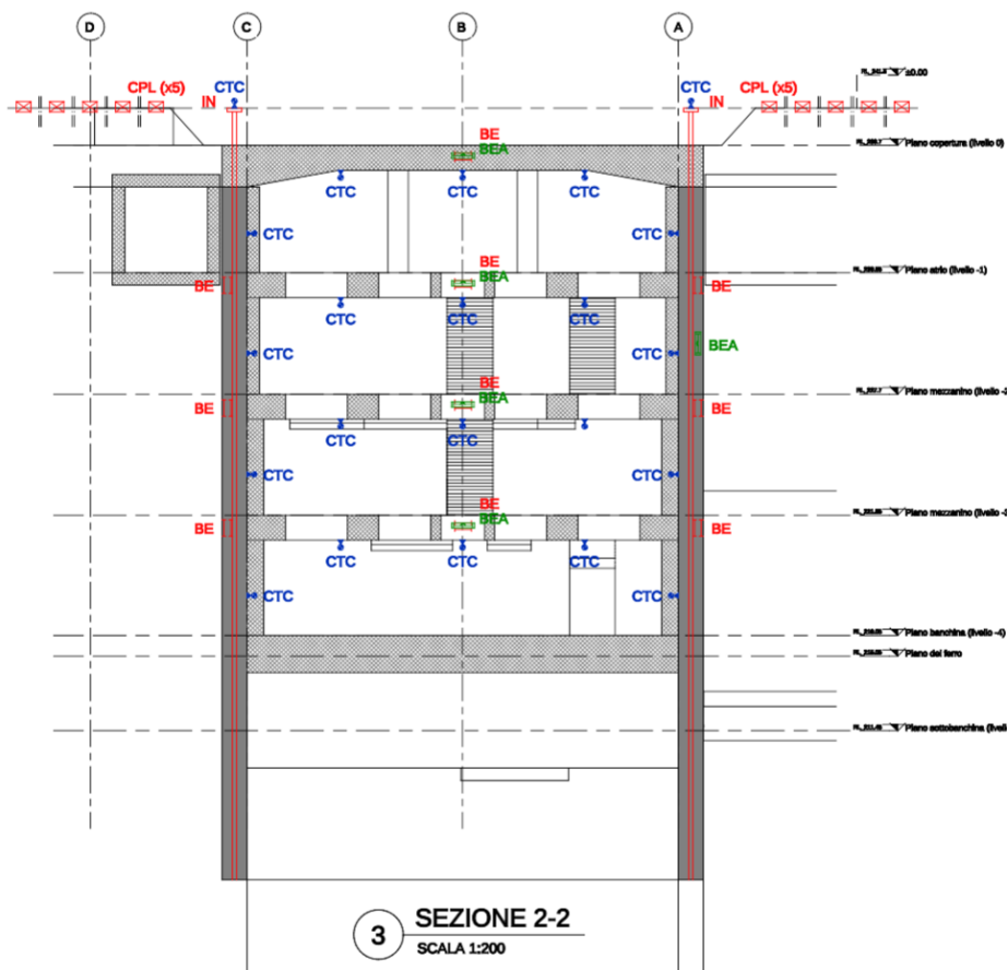
Figura 26. Schema di monitoraggio – Sezione 2-2 (MTL2T1A2DPRCSNOT001). Per le rimanenti sezioni, vedasi la tavola di riferimento.
