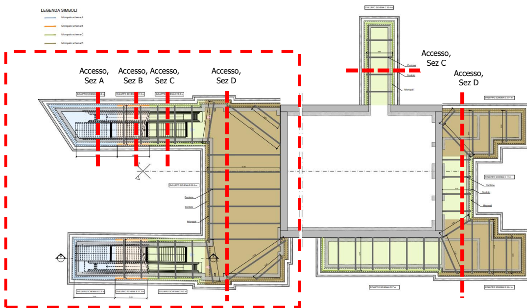
Figura 10. Tipologici delle sezioni di scavo degli accessi (MTL2T1A2DSTRSMOT020.1)
