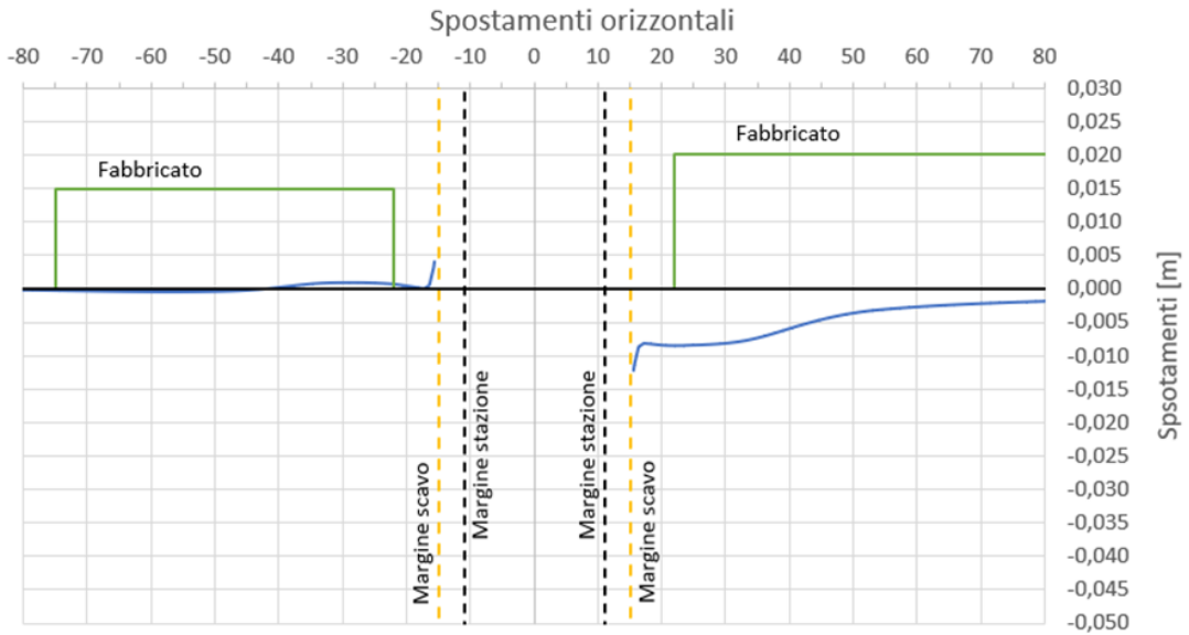
Figura 12. Spostamenti orizzontali
