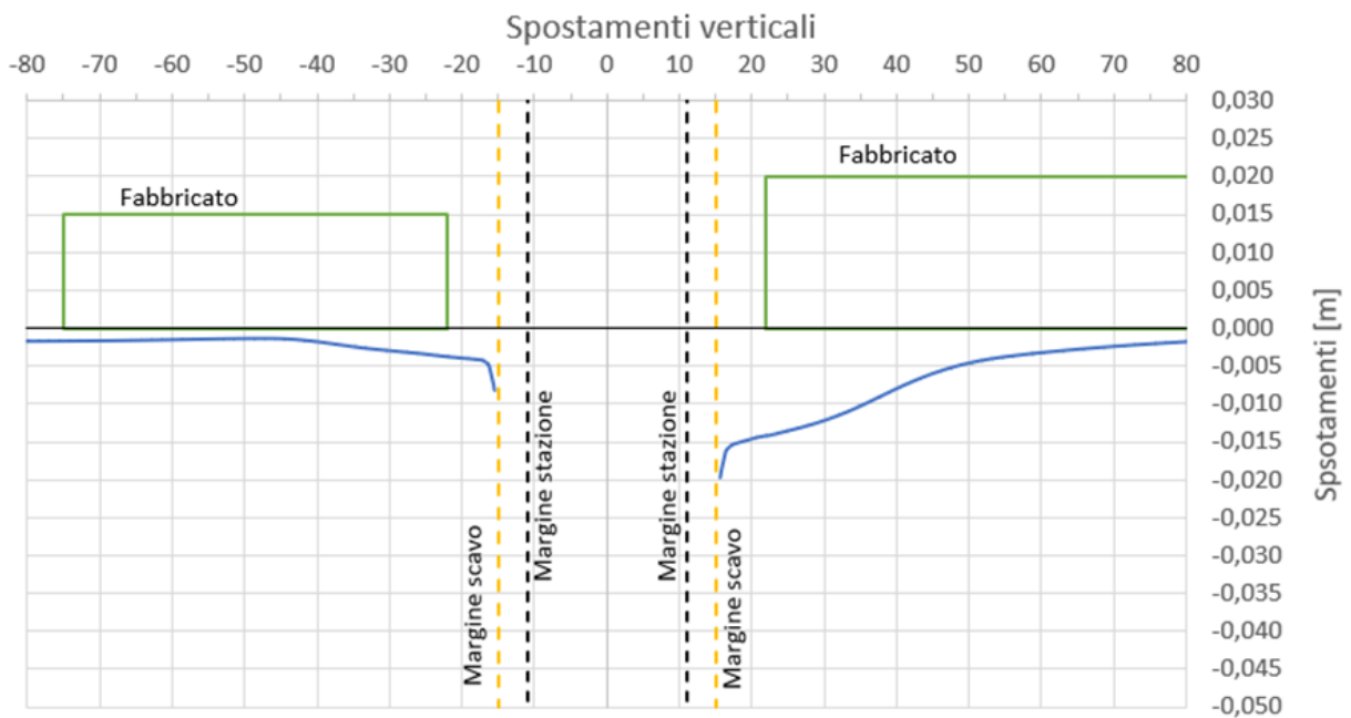
Figura 11. Spostamenti verticali
