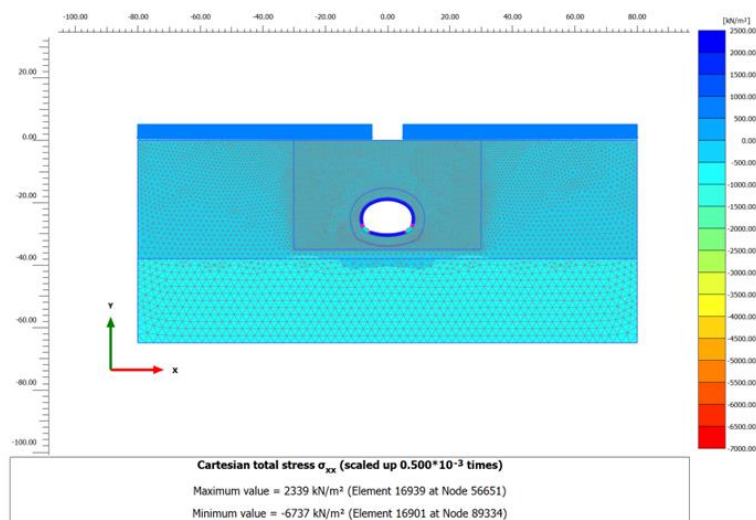
Figura 17. Sezione Galleria Banchina: \sigma_{xx} , a fase 8
