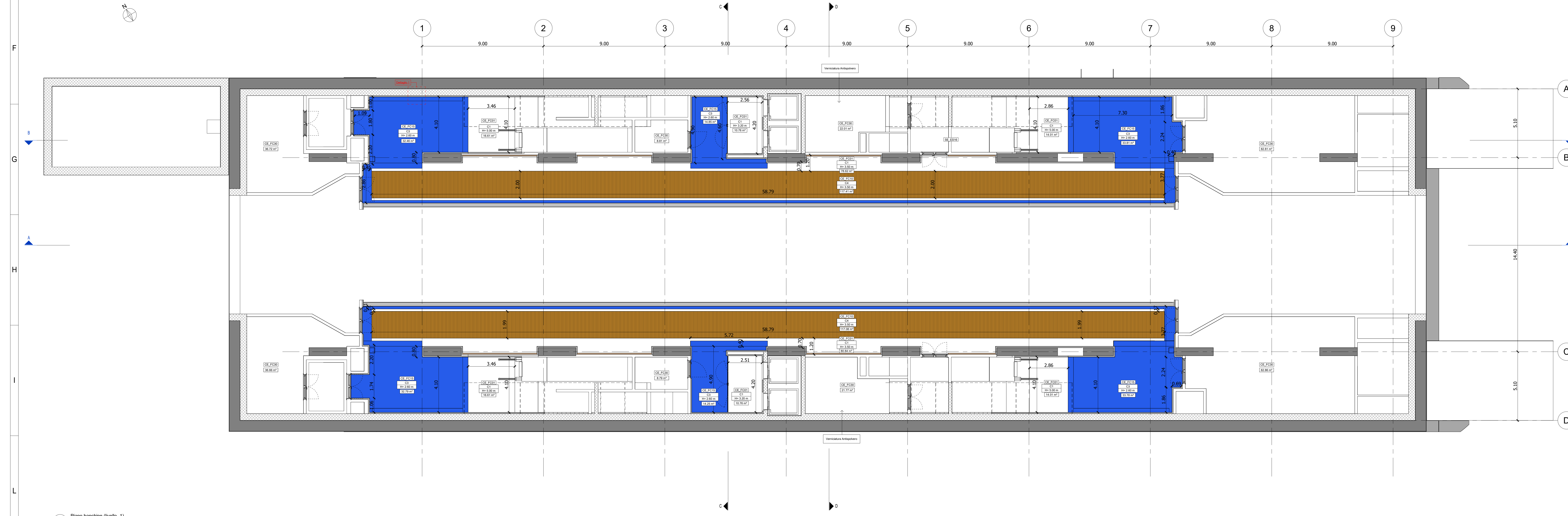
2 Piano banchine (livello -1)
