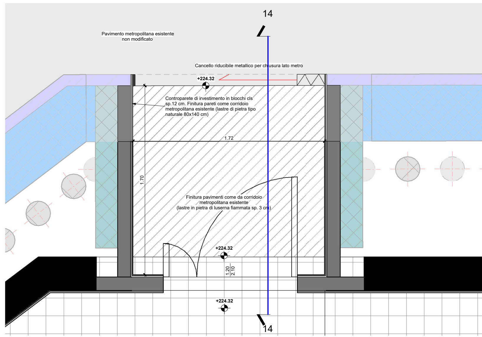
DETTAGLIO 01 COLLEGAMENTO METROPOLITANA NE 1 : 20
