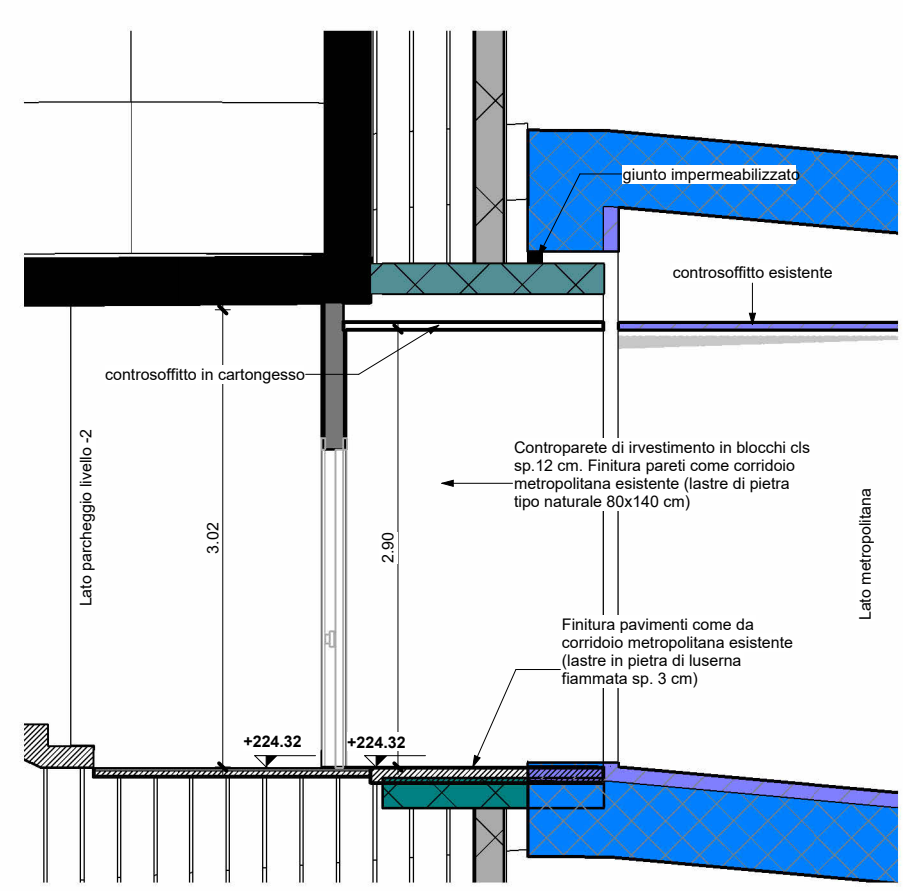
Sezione 14 1 : 50
