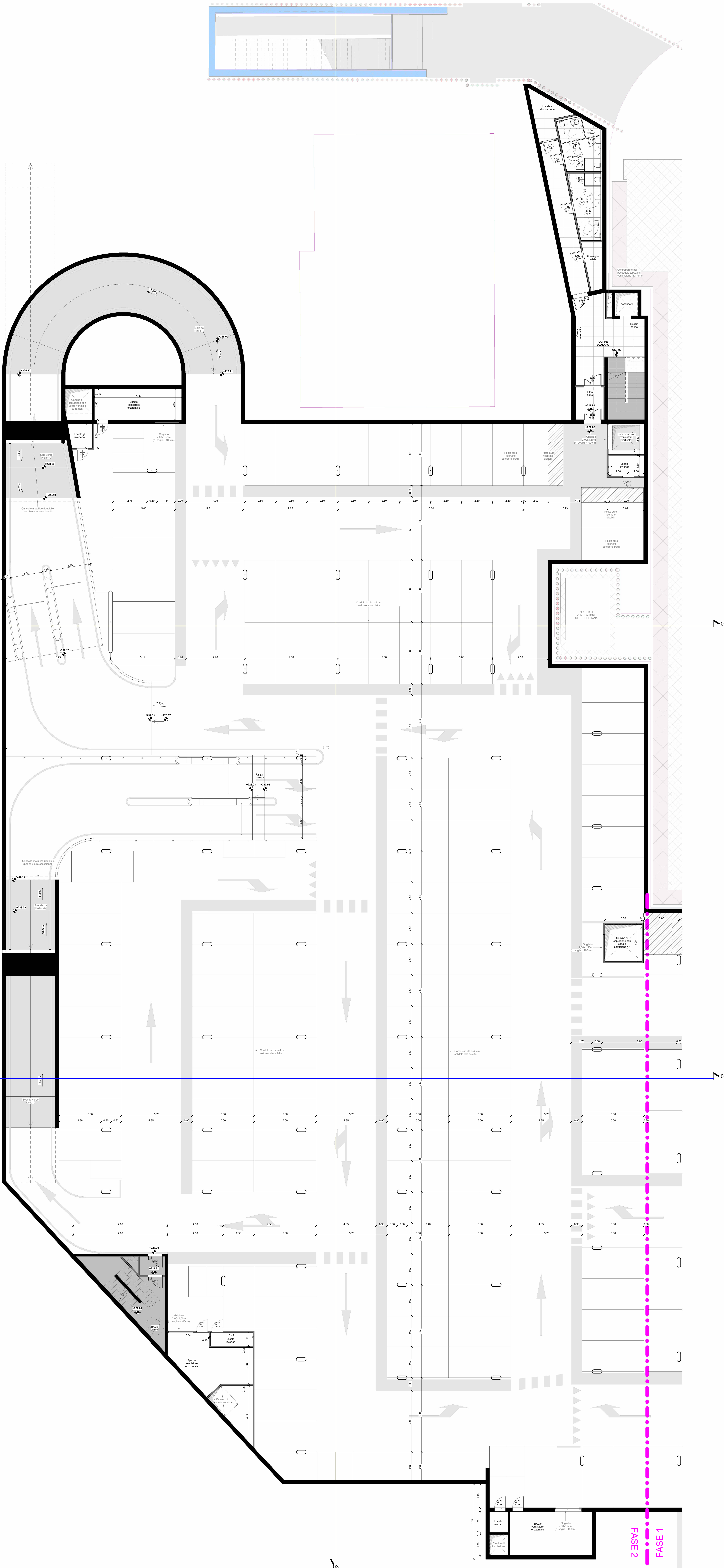
PIANTA LIVELLO -1 Blocco B 1 : 100
