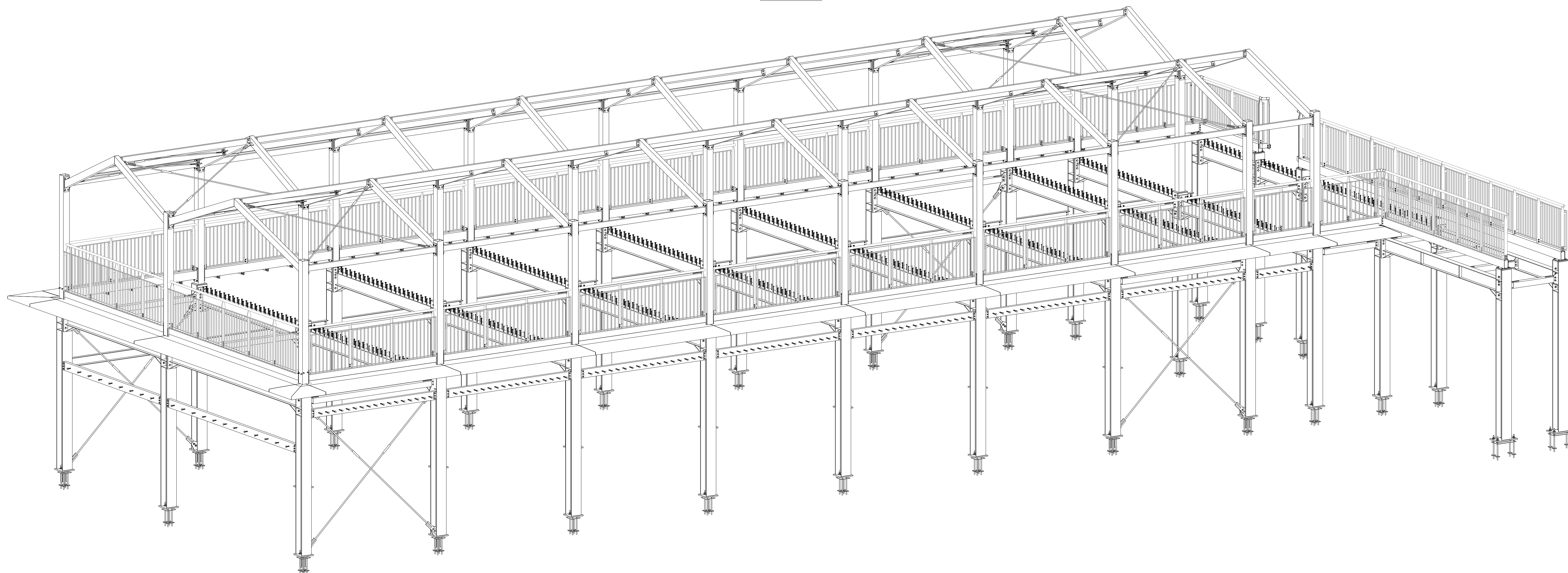
ASSONOMETRIA
