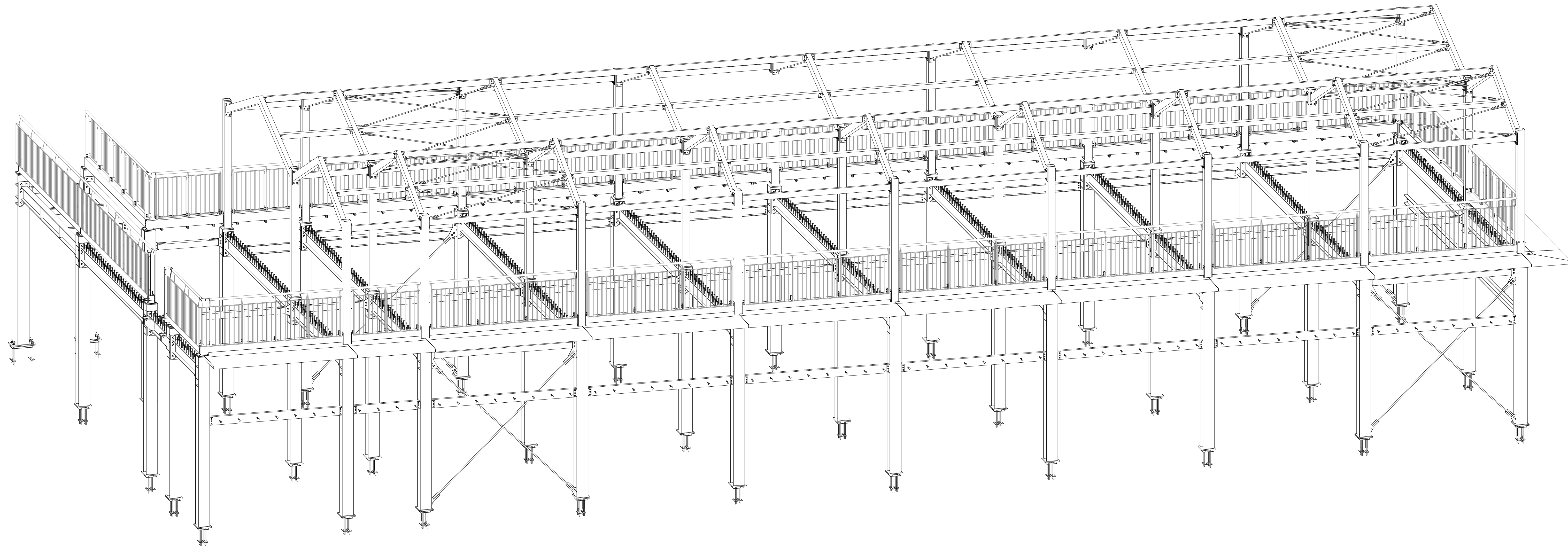
ASSONOMETRIA
