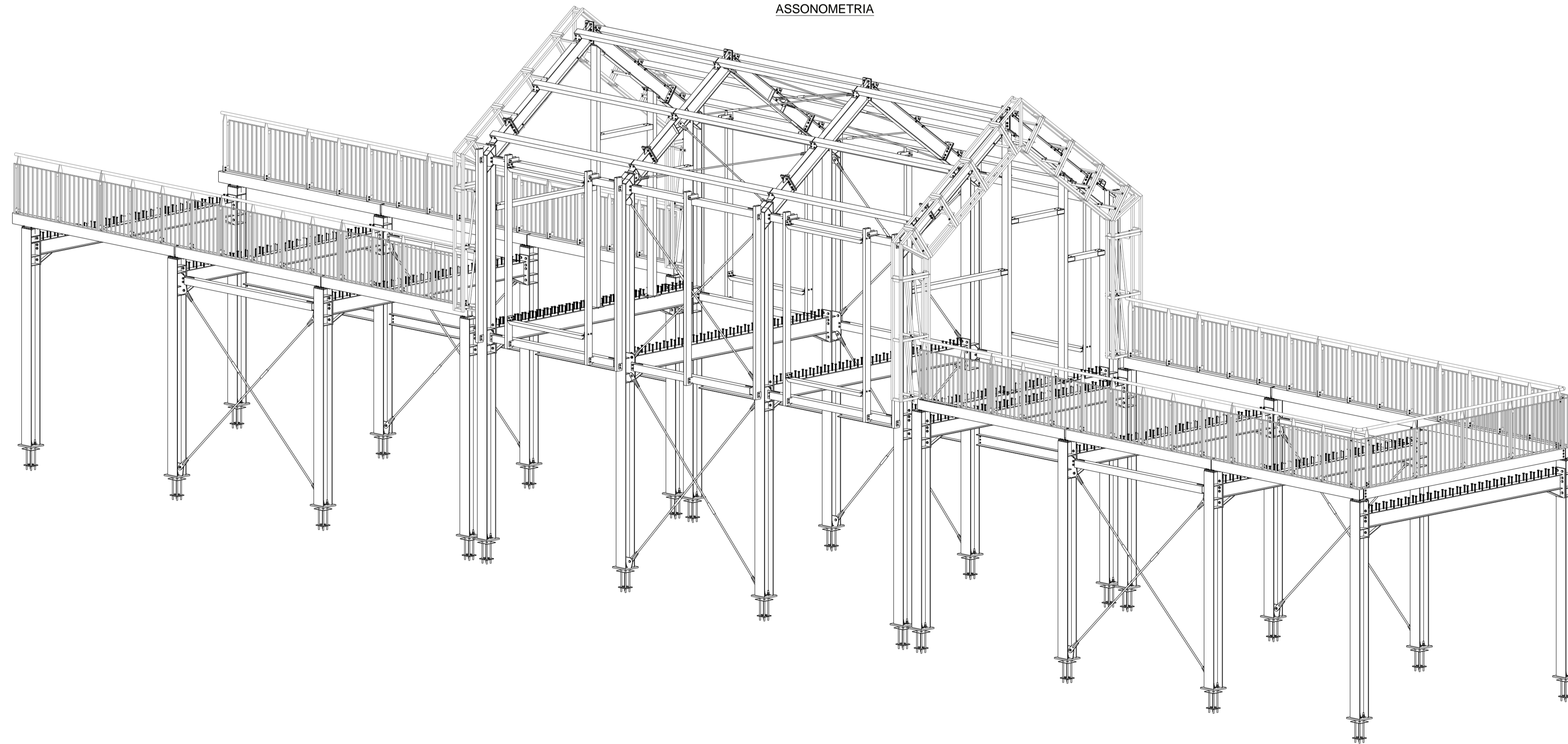
ASSONOMETRIA
