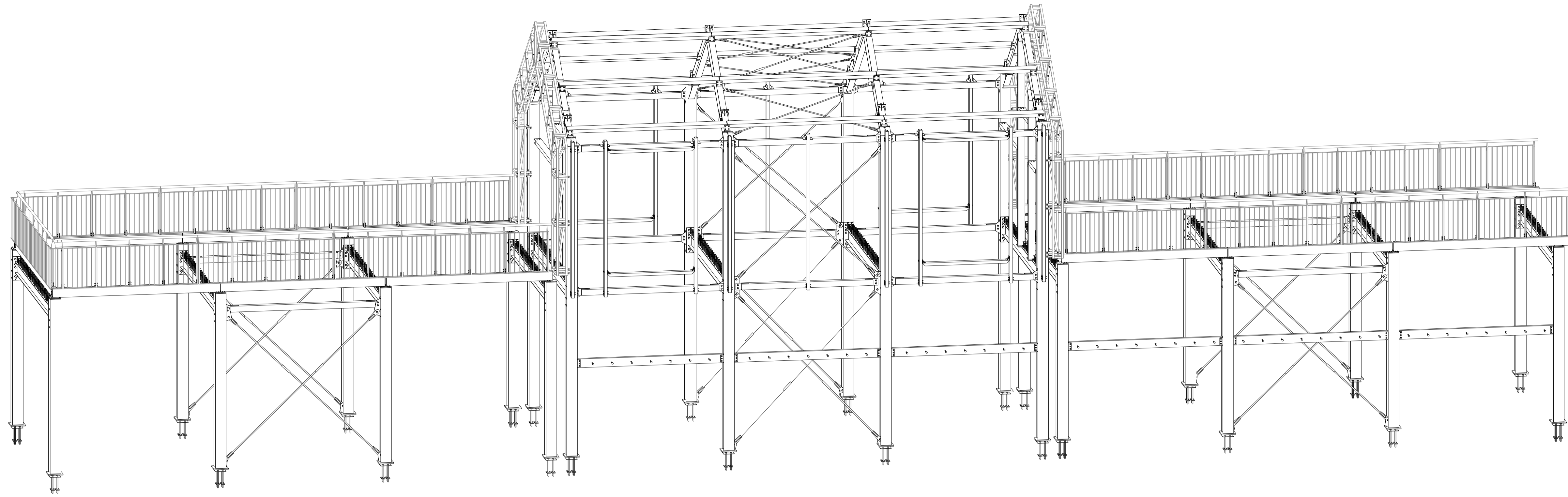
ASSONOMETRIA
