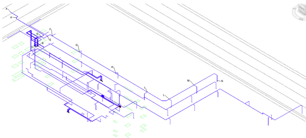
Figura 4 - Schema rete di adduzione idrica
