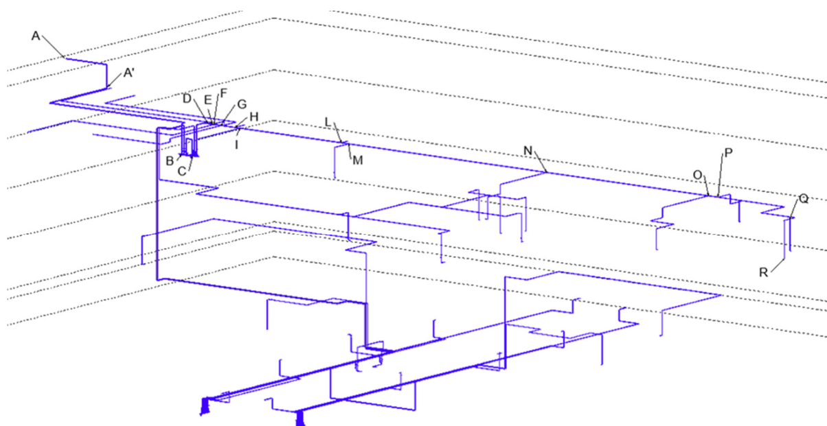
Figura 4 - Schema rete di adduzione idrica
