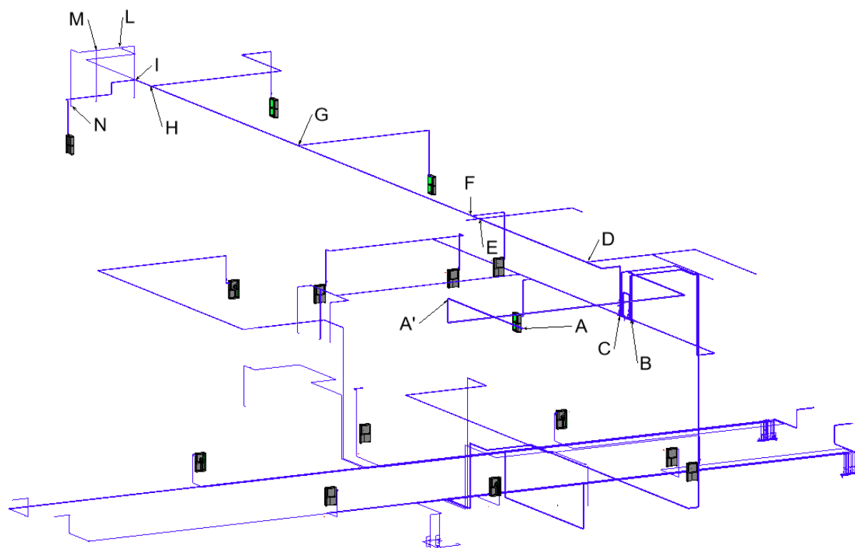
Figura 4 - Schema rete di adduzione idrica
