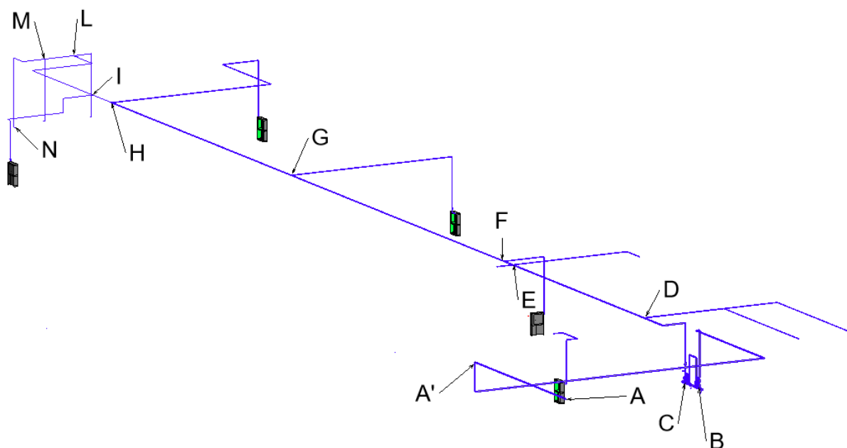
Figura 5 – Percorso critico
