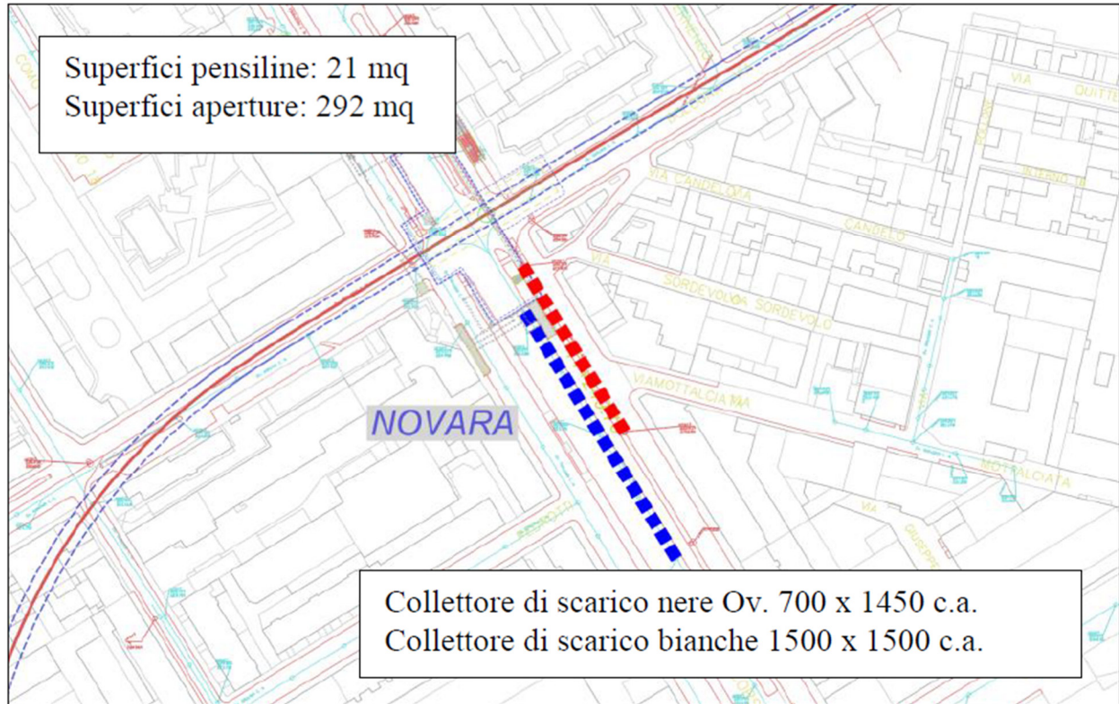
Figura 2. Individuazione superfici pensiline, aperture e individuazione recettore
