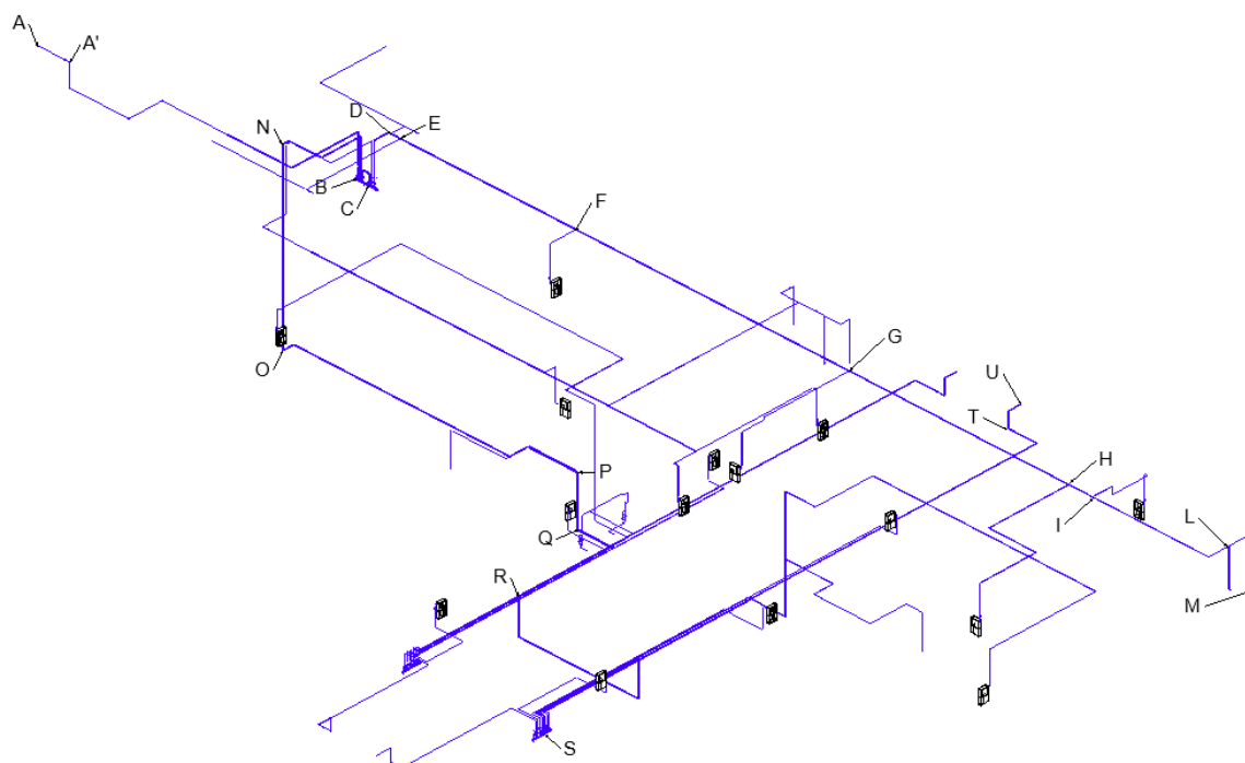
Figura 4 - Schema rete di adduzione idrica
