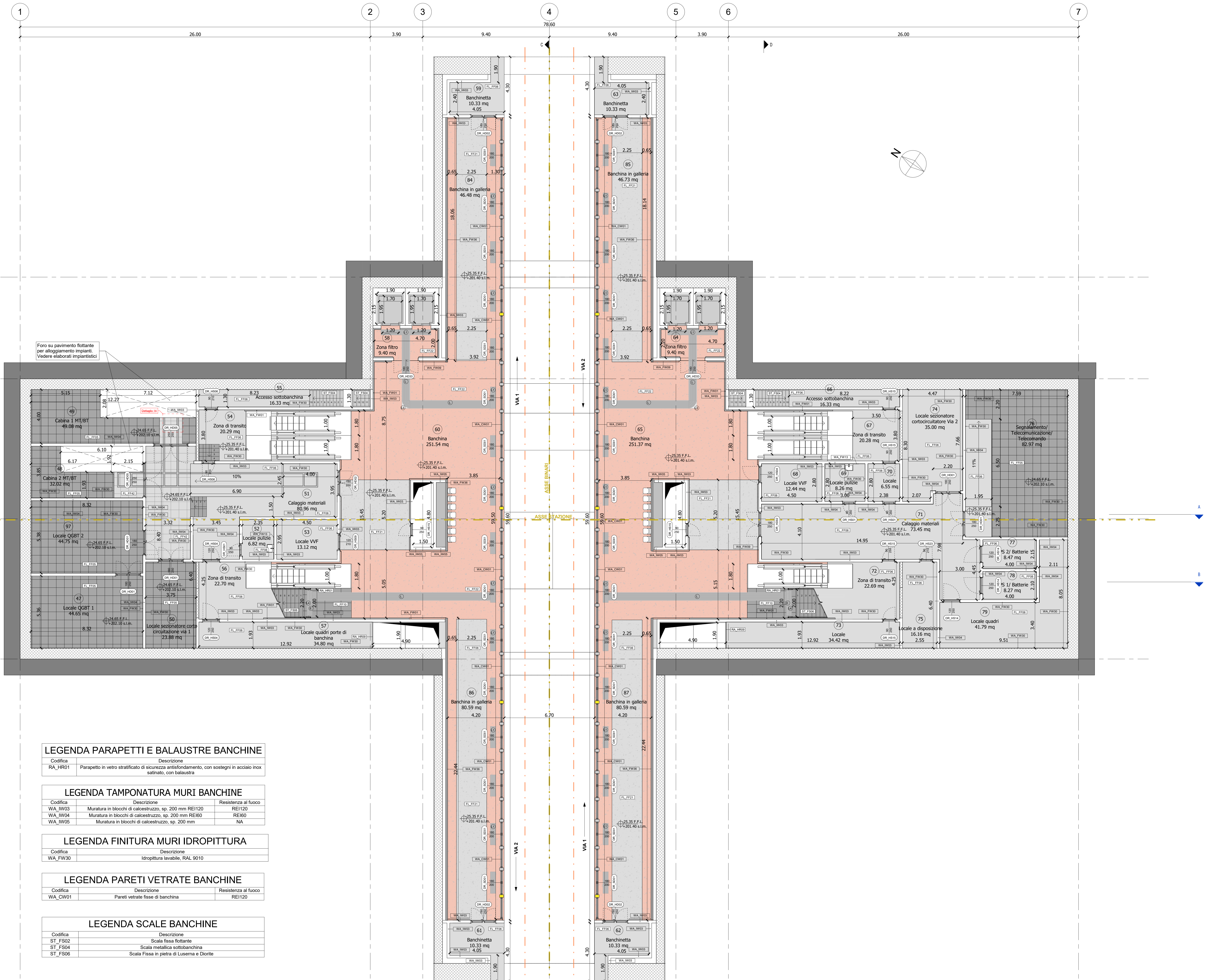
1 Piano banchine (livello -4)
