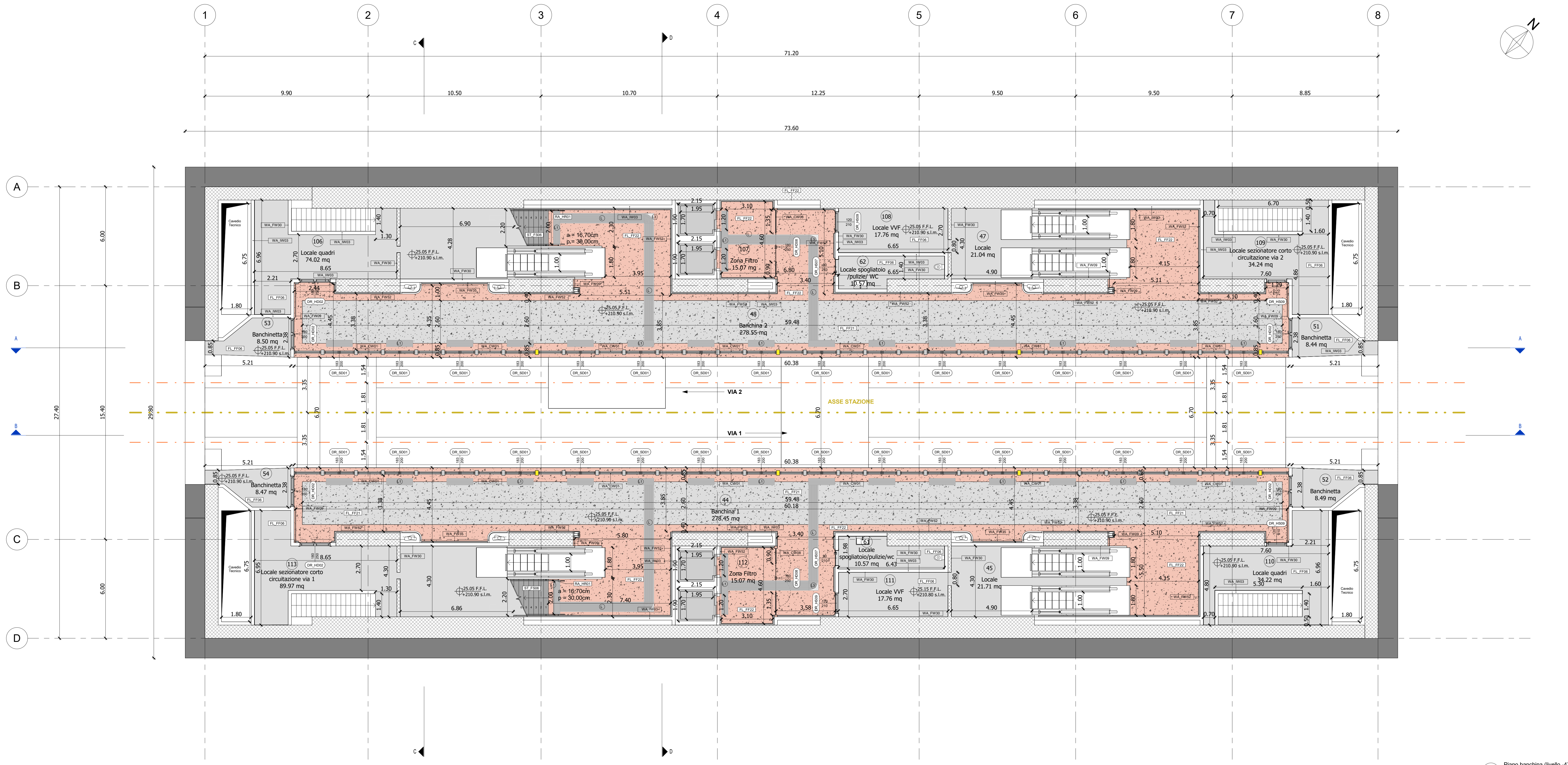
1 Piano banchina (livello -4)
