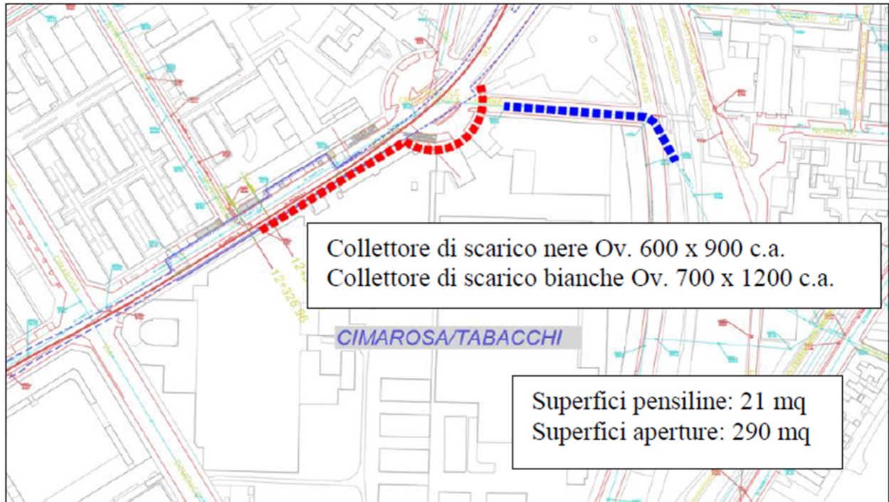
Figura 2. Individuazione superfici pensiline, aperture e individuazione recettore
