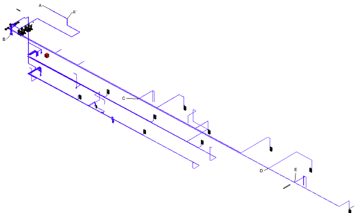
Figura 4 - Schema rete di adduzione idrica
