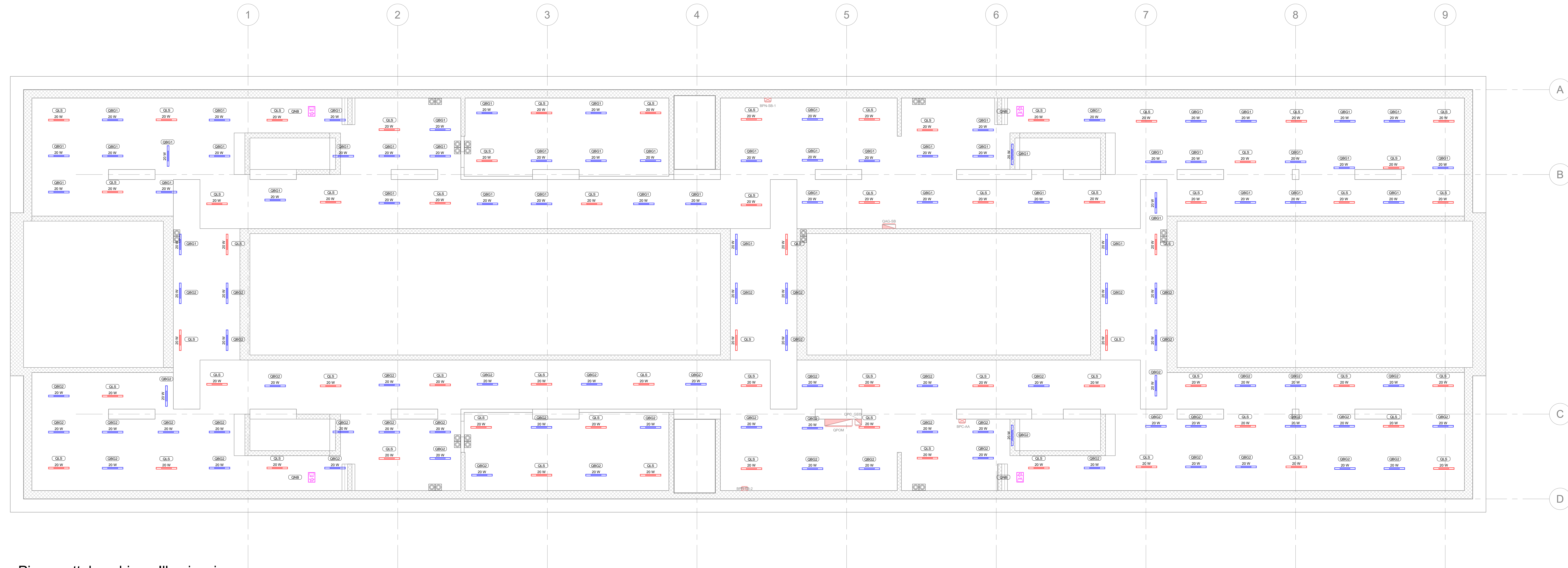
1 Piano sottobanchine - Illuminazione 1 : 100
