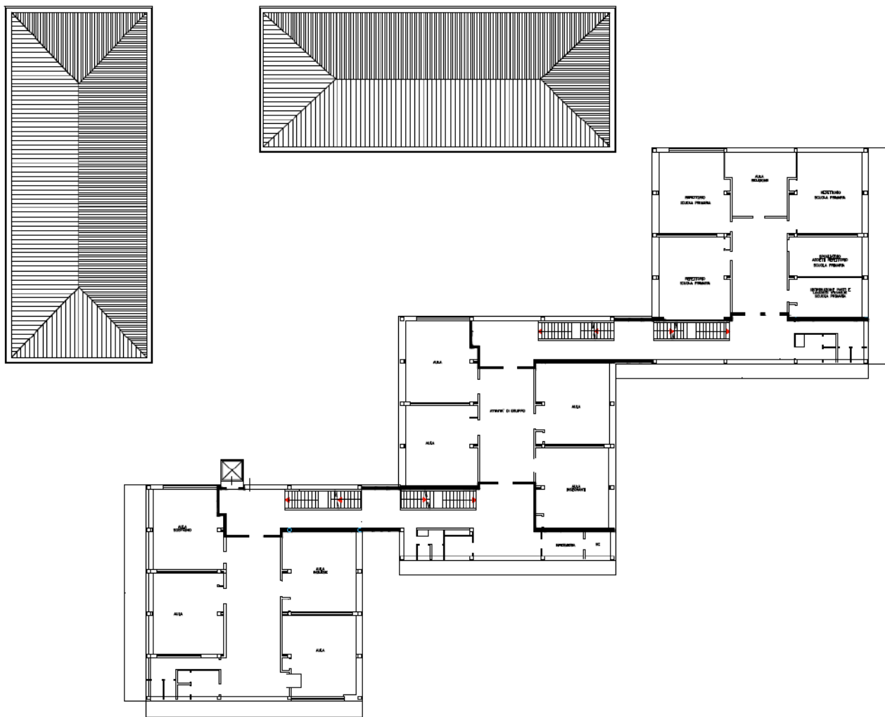
Figura 18 - Pianta piano secondo
