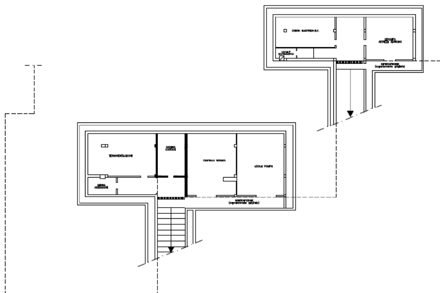
Figura 15 - Pianta piano seminterrato
