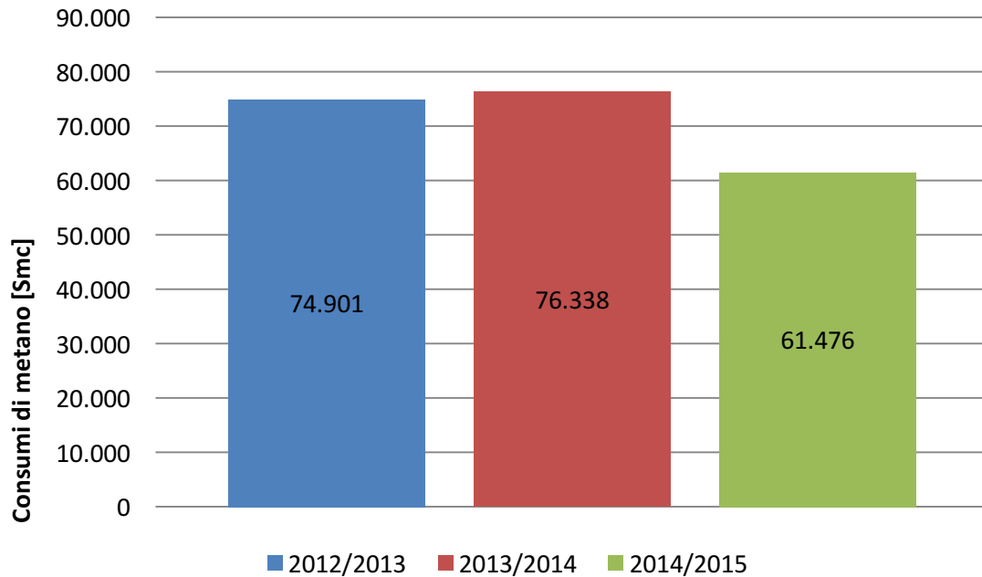
Figura 10 - Consumi di metano normalizzati ultime tre stagioni di riscaldamento
