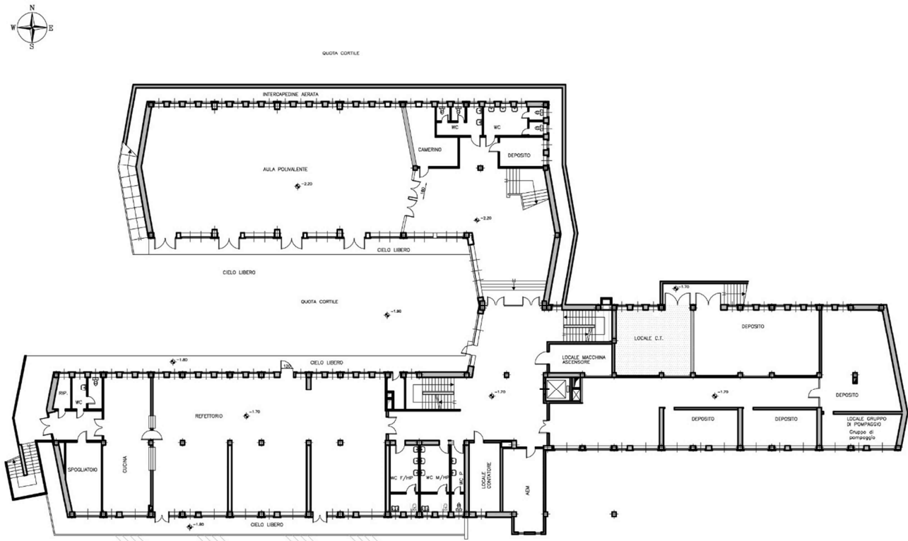
Figura 15 - Pianta piano seminterrato
