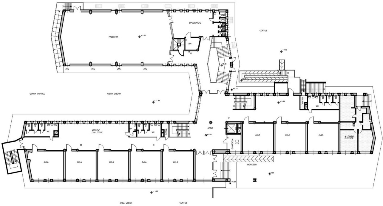
Figura 16 - Pianta piano terra
