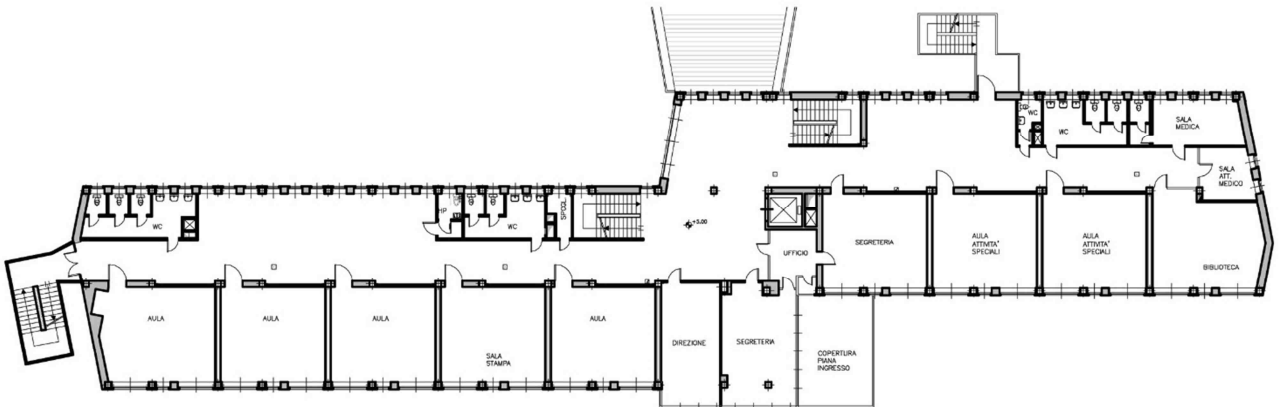
Figura 17 - Pianta piano primo
