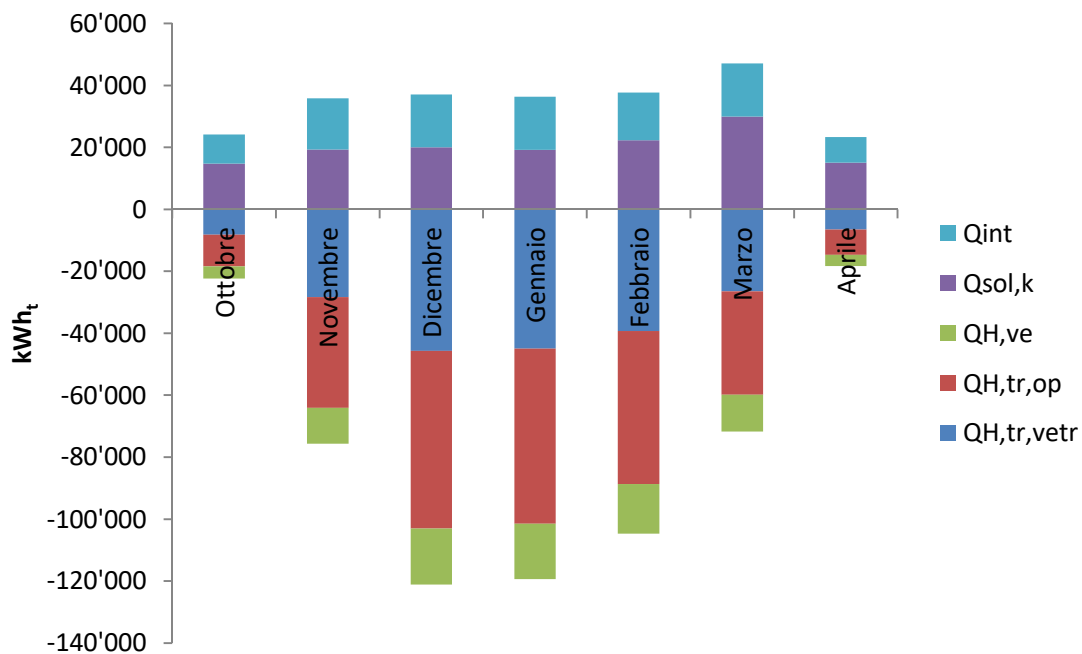
Figura 21 - Andamento mensile dispersioni ed apporti edificio
