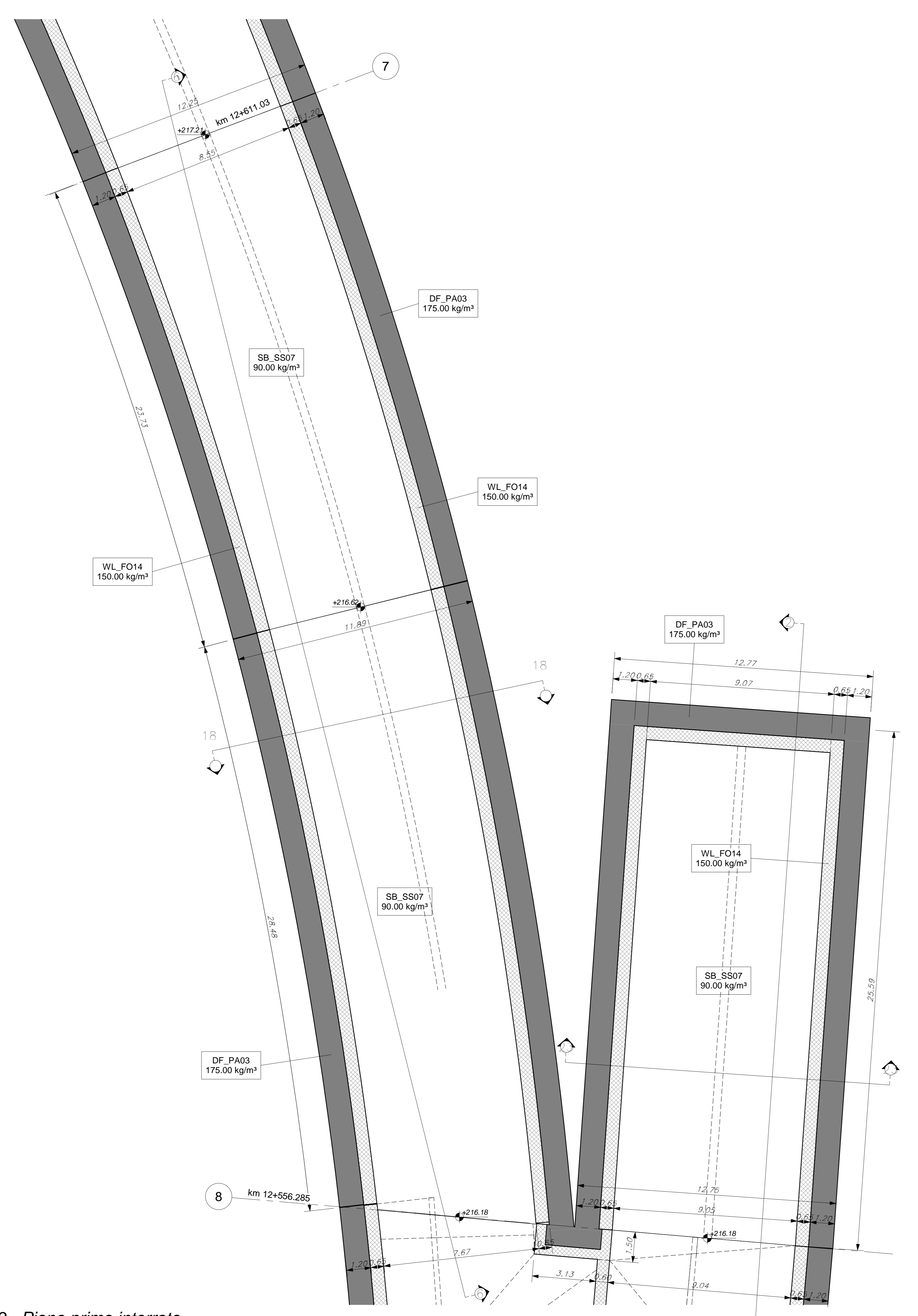
3 - Piano primo interrato Scala 1 : 100
