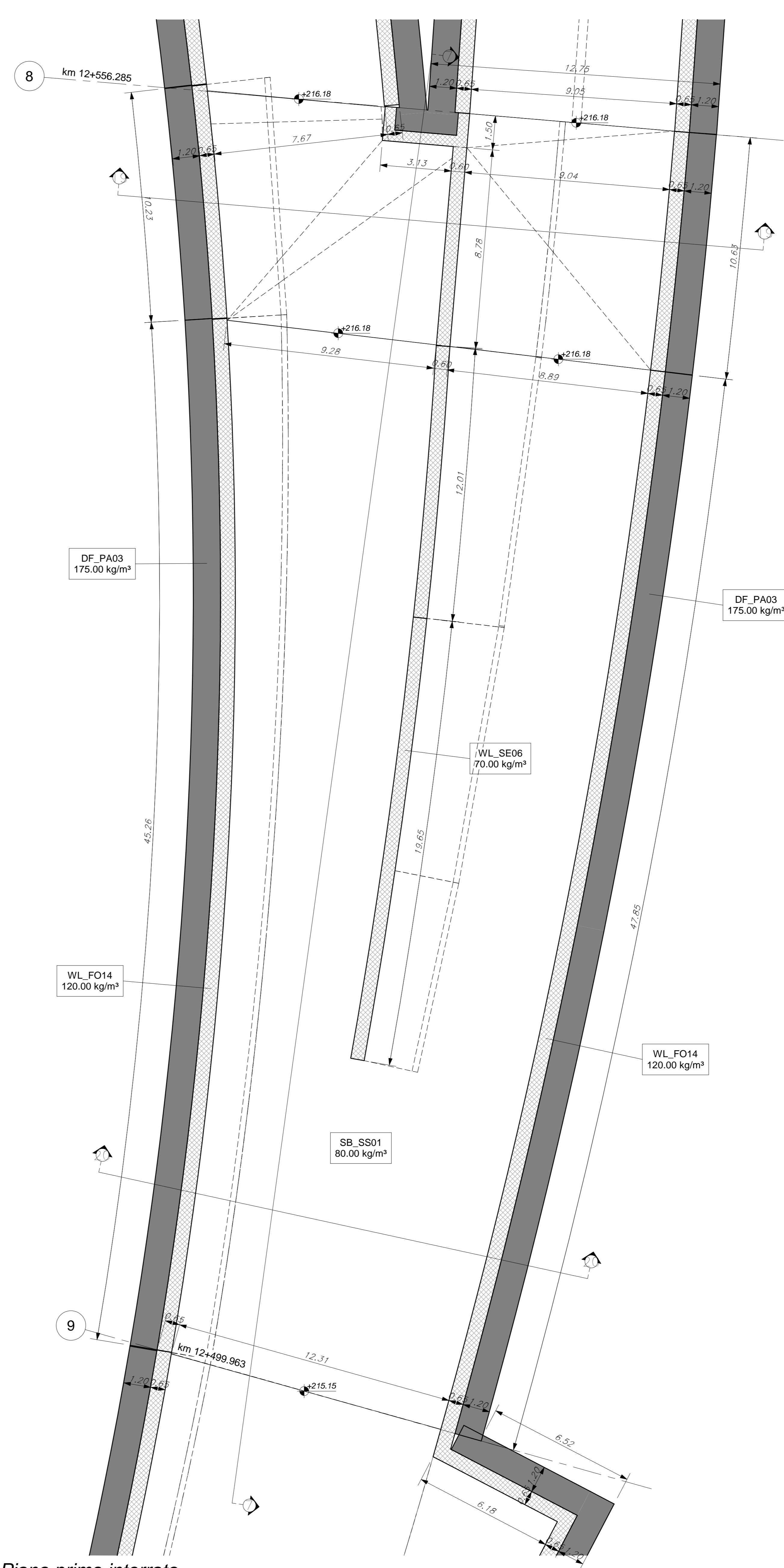
4 - Piano primo interrato Scala 1 : 100
