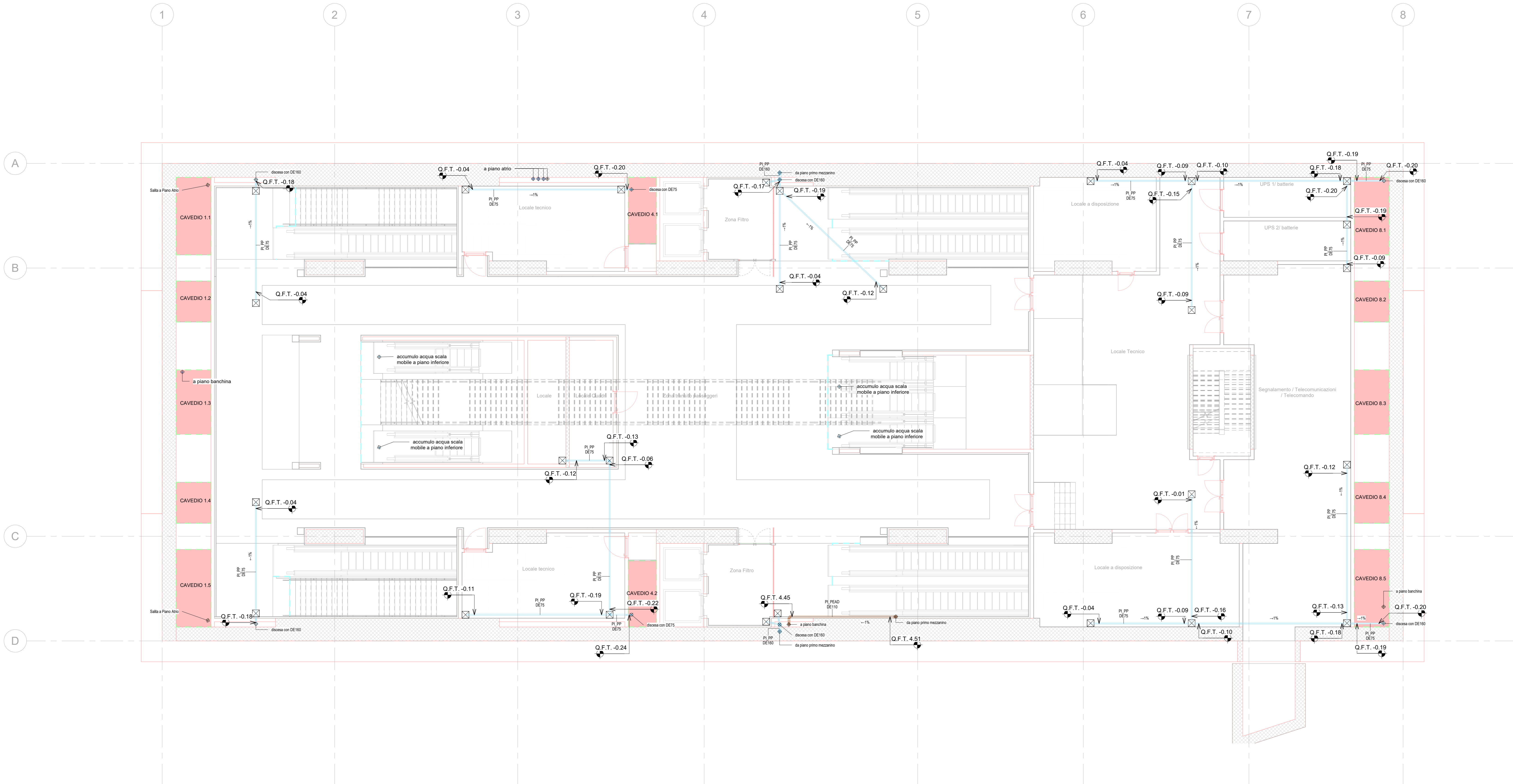
1 SC_Piano secondo mezzanino (livello -3) 1 : 100
