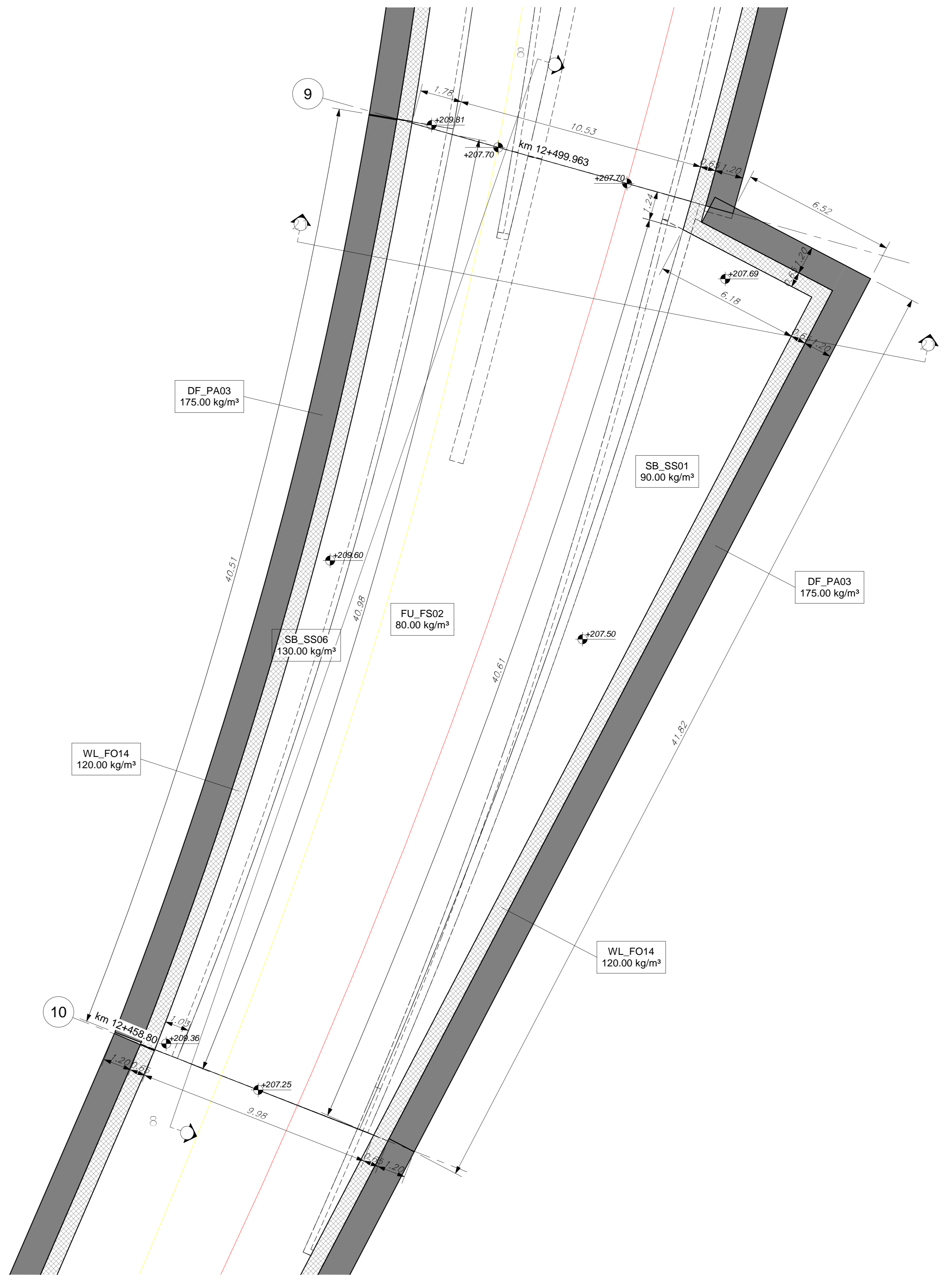
2 - Piano secondo interrato Scala 1 : 100
