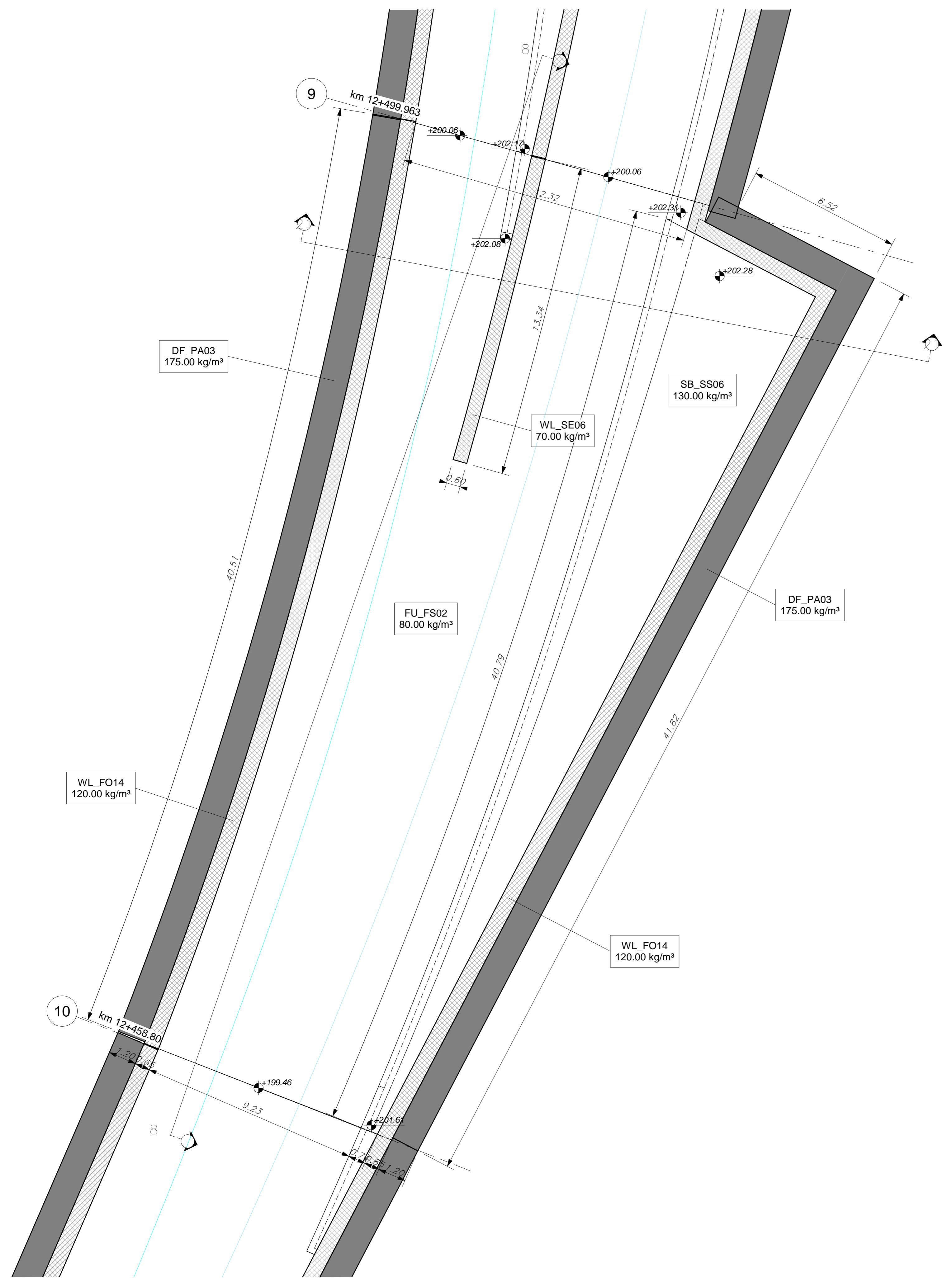
2 - Piano terzo interrato Scala 1 : 100
